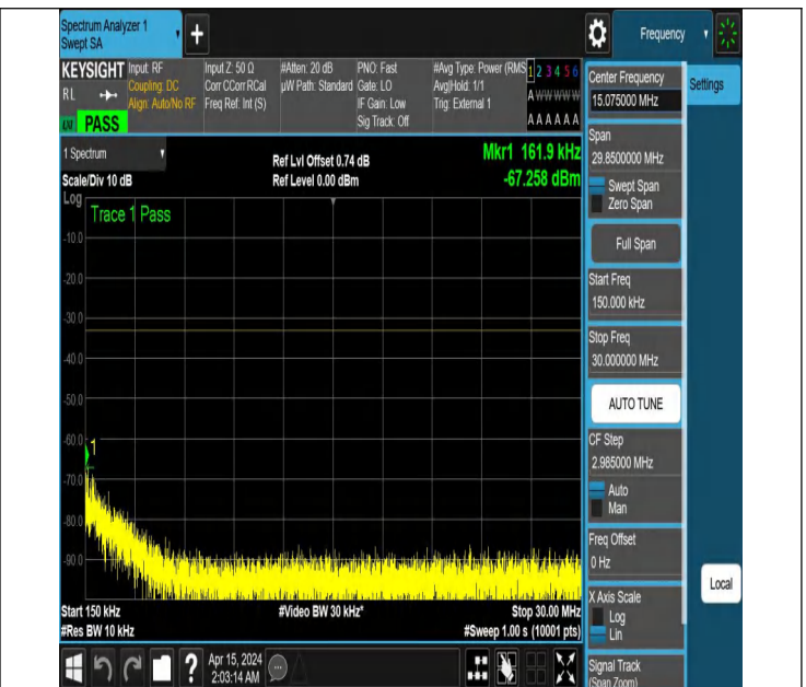
NTNV_N77-3450-3550_PC2_30_60_L_TID2_NS_01_0.15_30_#
