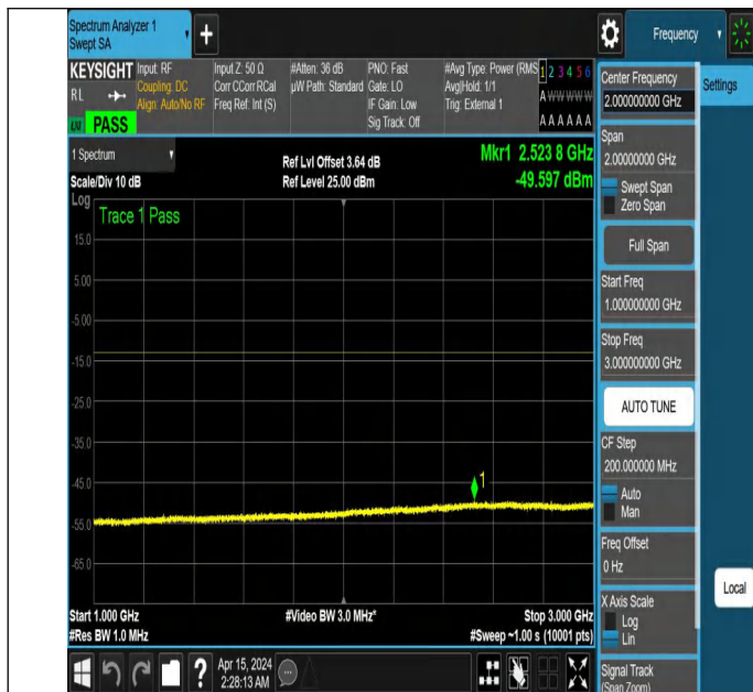
NTNV_N77-3450-3550_PC2_30_60_L_TID6 NS_01_1000_3000
