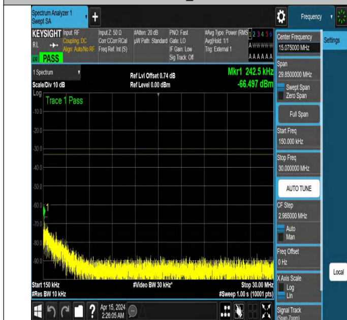
NTNV_N77-3450-3550_PC2_30_60_L_TID6_NS_01_0.15_30_#
