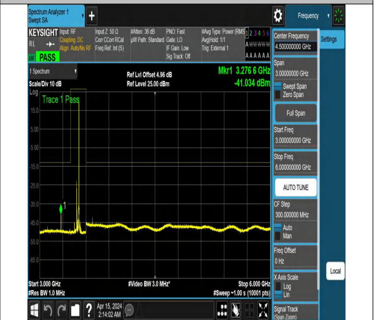
NTNV_N77-3450-3550_PC2_30_60_L_TID3_NS_01_3000_6000
