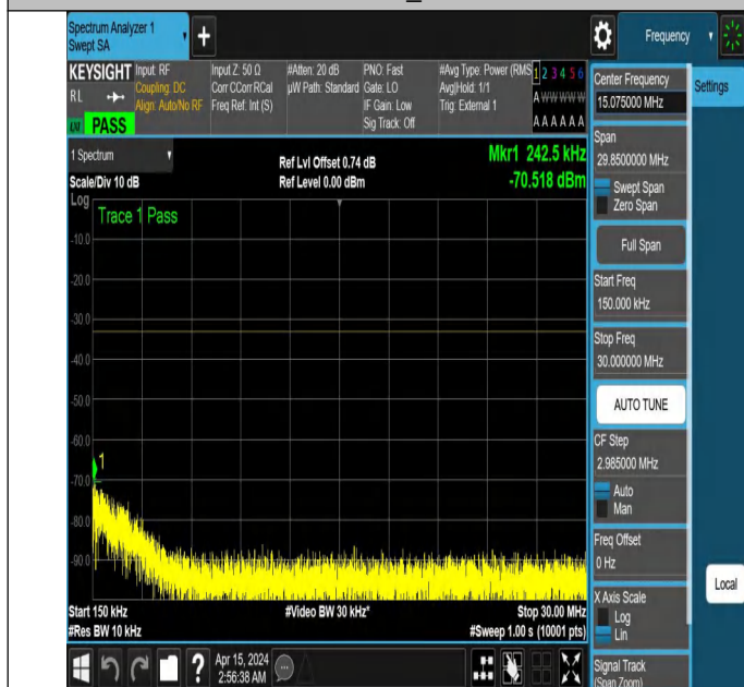
NTNV_N77-3450-3550_PC2_30_60_M_TID6_NS_01_0.15_30_#
