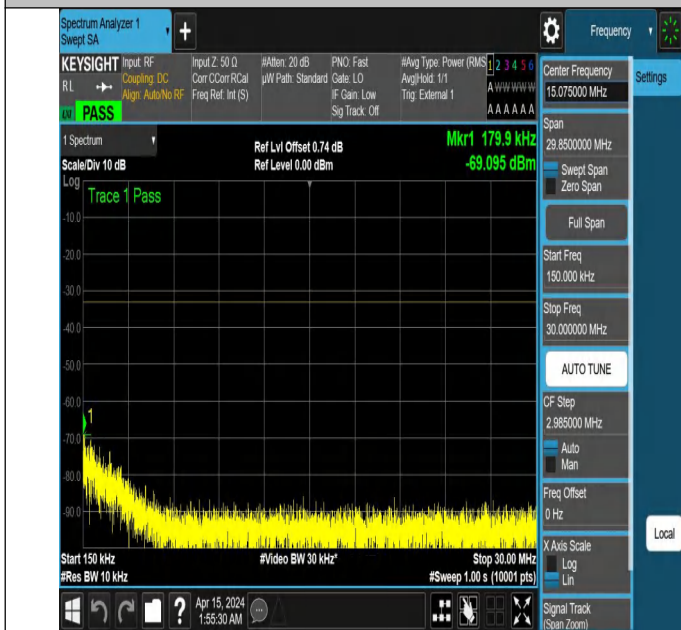
NTNV_N77-3450-3550_PC2_30_50_H_TID6_NS_01_0.15_30_#
