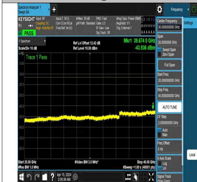
NTNV_N77-3450-3550_PC2_30_60_L_TID2_NS_01_20000_400
