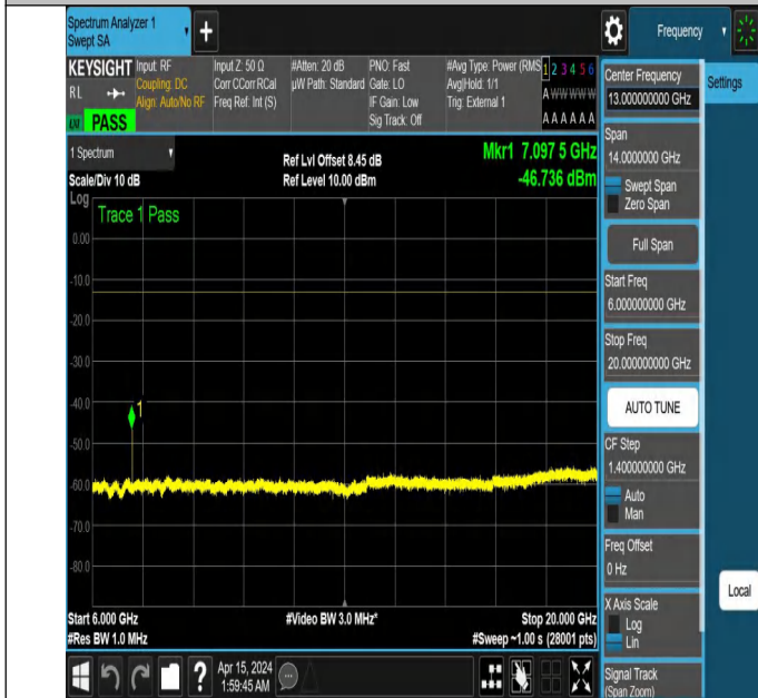
NTNV_N77-3450-3550_PC2_30_50_H_TID6_NS_01_6000_2000
