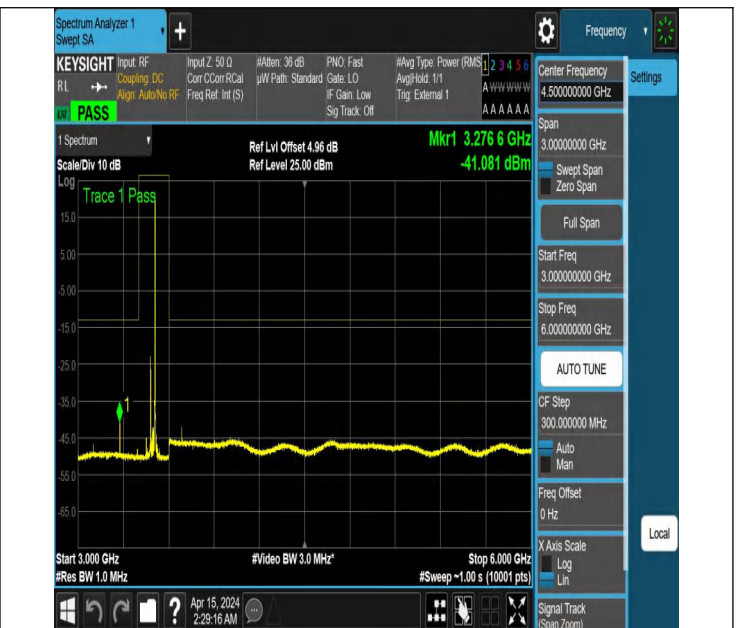
NTNV_N77-3450-3550_PC2_30_60_L_TID6_NS_01_3000_6000
