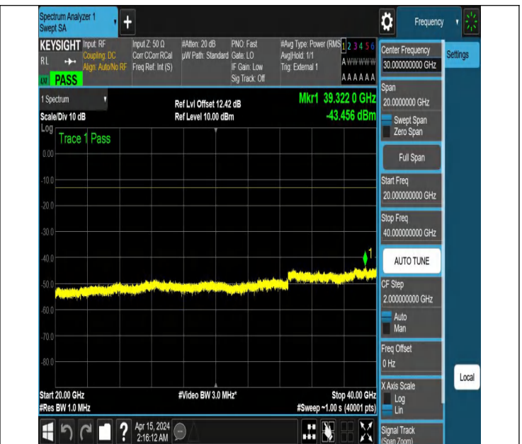
NTNV_N77-3450-3550_PC2_30_60_L_TID3_NS_01_20000_400
