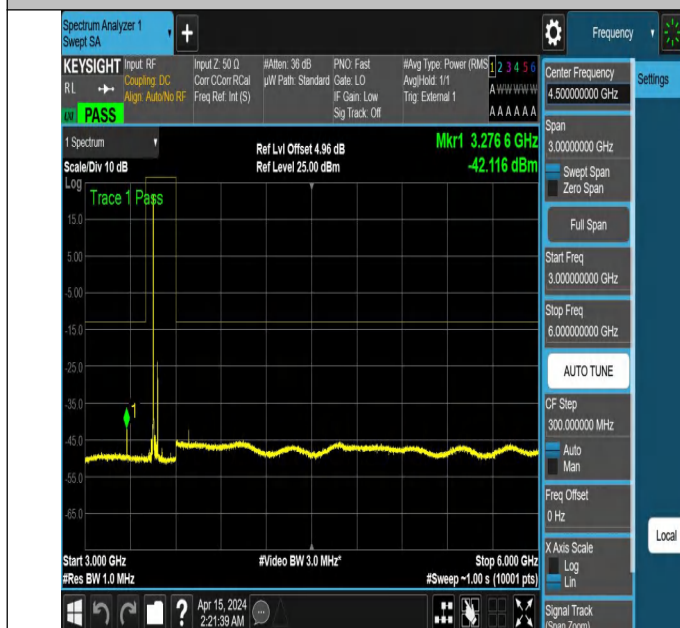
NTNV_N77-3450-3550_PC2_30_60_L_TID5_NS_01_3000_6000
