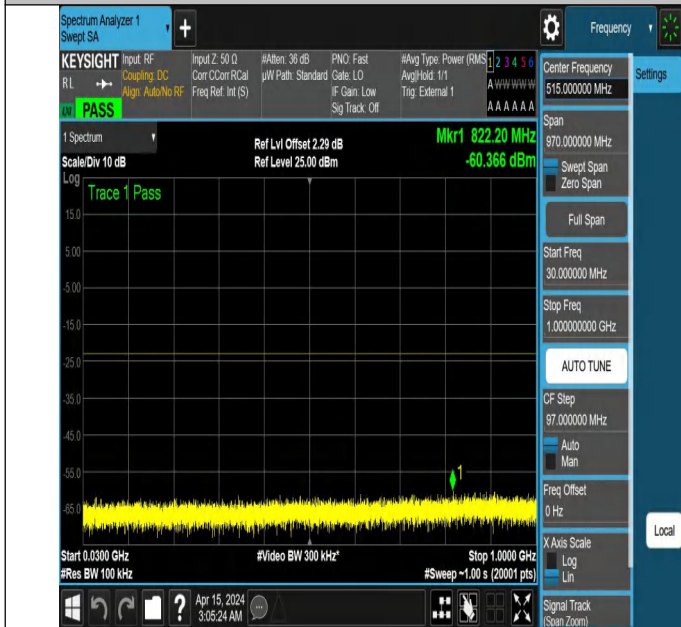
NTNV_N77-3450-3550_PC2_30_60_H_TID2_NS_01_30_1000_#
