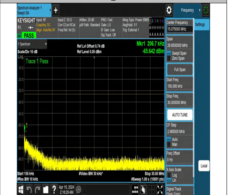
NTNV_N77-3450-3550_PC2_30_60_L_TID5_NS_01_0.15_30_#
