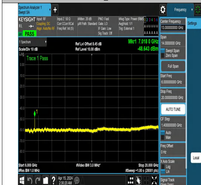
NTNV_N77-3450-3550_PC2_30_60_L_TID6_NS_01_6000_2000
