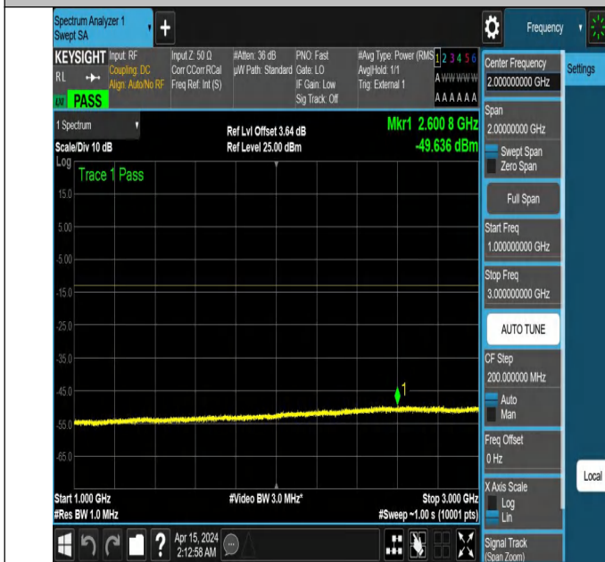
NTNV_N77-3450-3550_PC2_30_60_L_TID3_NS_01_1000_3000
