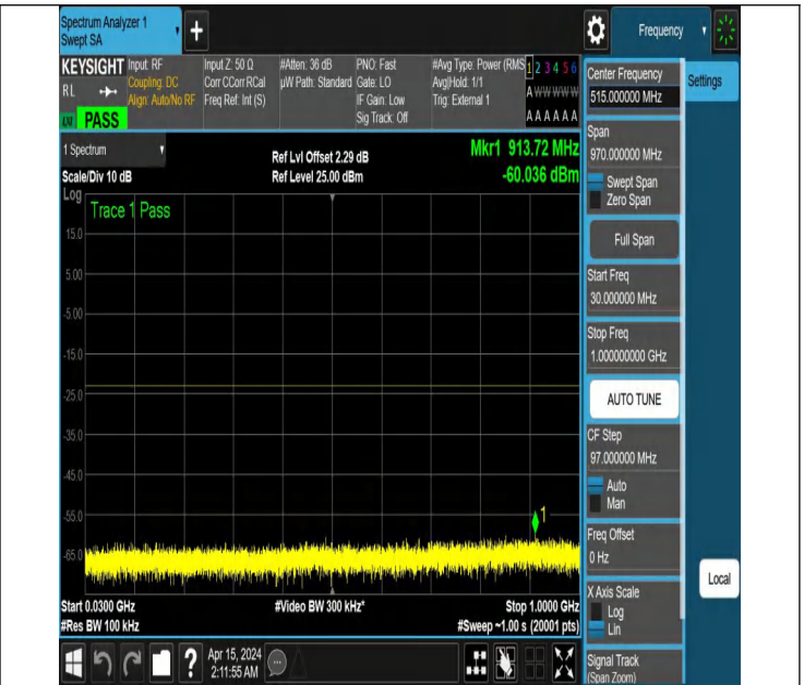
NTNV_N77-3450-3550_PC2_30_60_L_TID3_NS_01_30_1000_#
