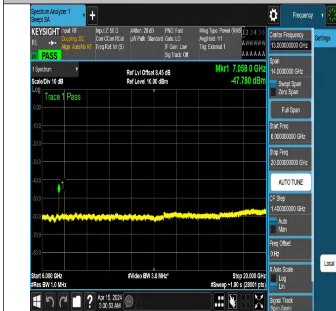
NTNV_N77-3450-3550_PC2_30_60_M_TID6_NS_01_6000_200
