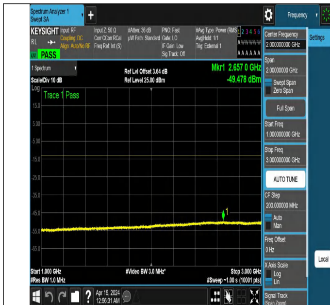
NTNV_N77-3450-3550_PC2_30_50_L_TID6 NS_01_1000_3000
