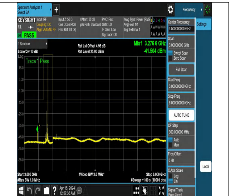
NTNV_N77-3450-3550_PC2_30_50_L_TID6_NS_01_3000_6000
