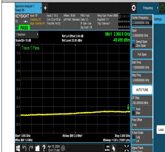
NTNV_N77-3450-3550_PC2_30_50_L_TID3_NS_01_1000_3000
