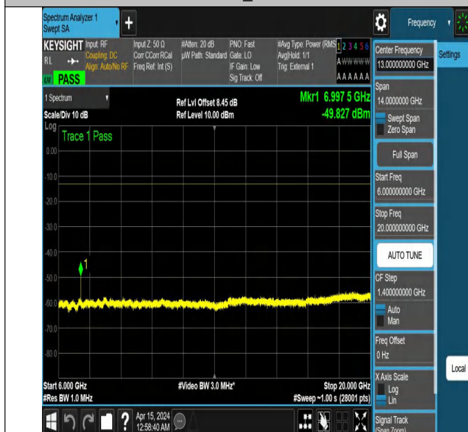
NTNV_N77-3450-3550_PC2_30_50_L_TID6_NS_01_6000_2000
