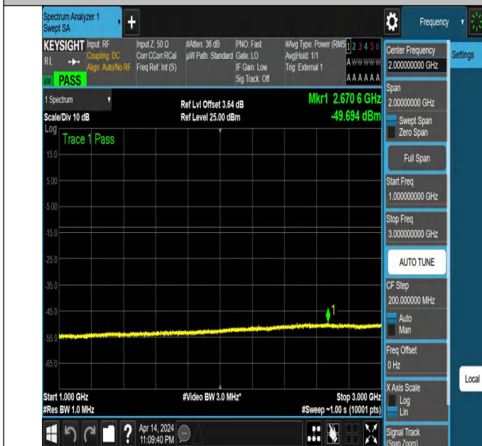
NTNV_N77-3450-3550_PC2_30_40_L_TID3_NS_01_1000_3000
