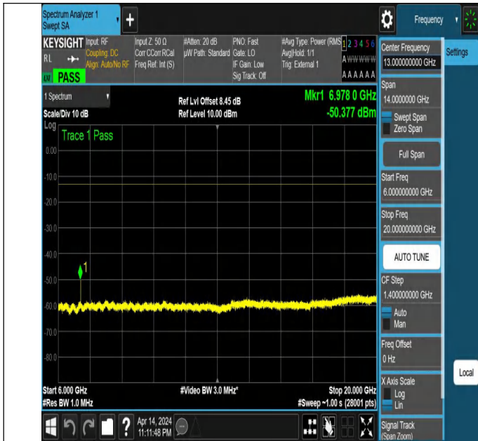
NTNV_N77-3450-3550_PC2_30_40_L_TID3_NS_01_6000_2000
