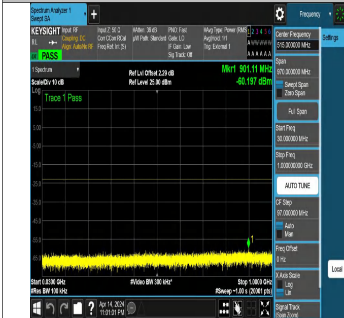
NTNV_N77-3450-3550_PC2_30_40_L_TID2_NS_01_30_1000_#
