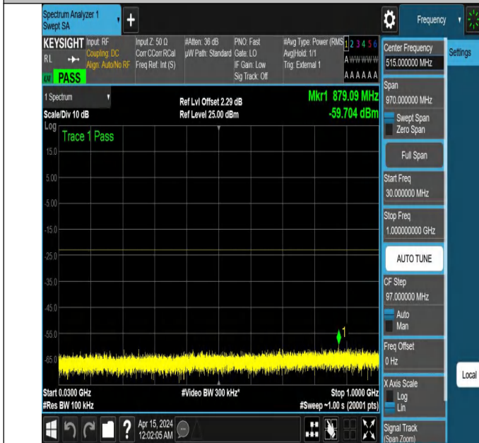
NTNV_N77-3450-3550_PC2_30_40_H_TID2_NS_01_30_1000_#
