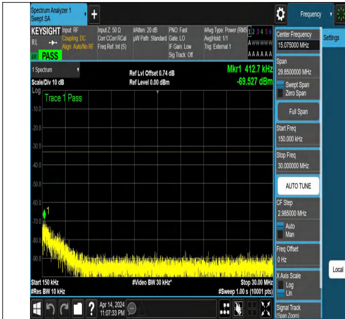
NTNV_N77-3450-3550_PC2_30_40_L_TID3_NS_01_0.15_30_#
