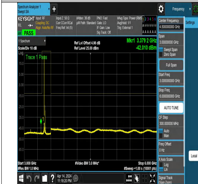
NTNV_N77-3450-3550_PC2_30_40_L_TID5_NS_01_3000_6000
