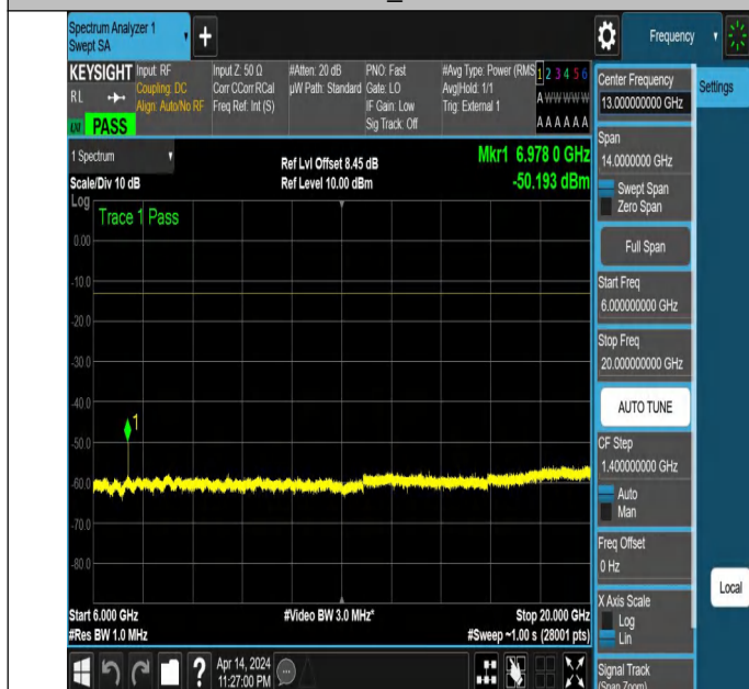
NTNV_N77-3450-3550_PC2_30_40_L_TID6_NS_01_6000_2000
