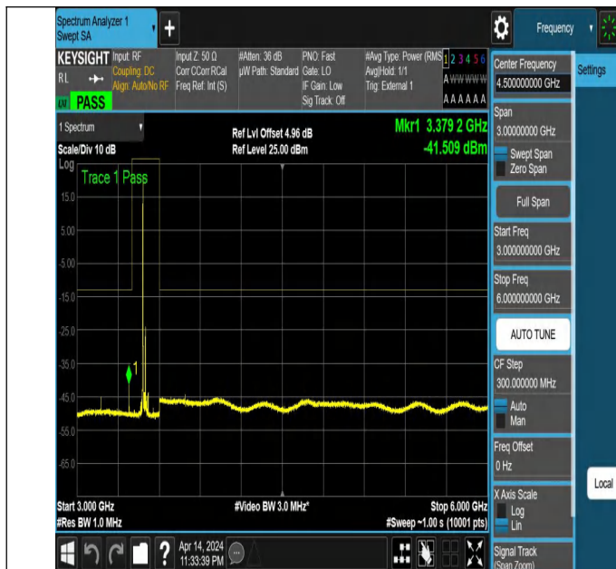
NTNV_N77-3450-3550_PC2_30_40_M_TID2_NS_01_3000_600
