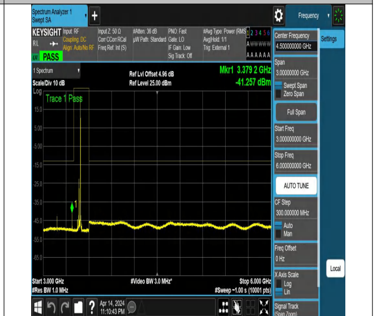
NTNV_N77-3450-3550_PC2_30_40_L_TID3_NS_01_3000_6000
