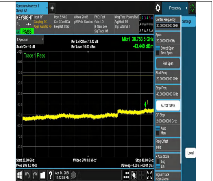
NTNV_N77-3450-3550_PC2_30_40_L_TID3_NS_01_20000_400
