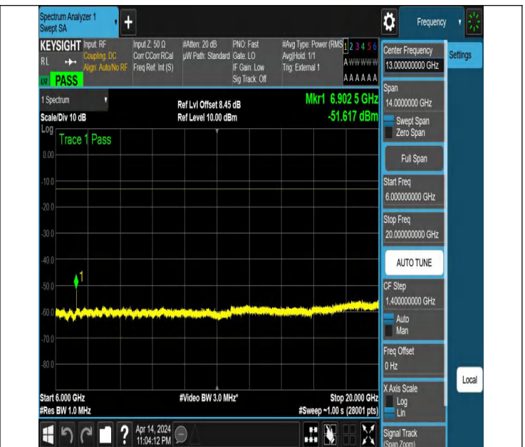
NTNV_N77-3450-3550_PC2_30_40_L_TID2_NS_01_6000_2000
