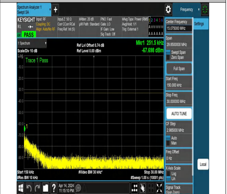
NTNV_N77-3450-3550_PC2_30_40_L_TID5_NS_01_0.15_30_#
