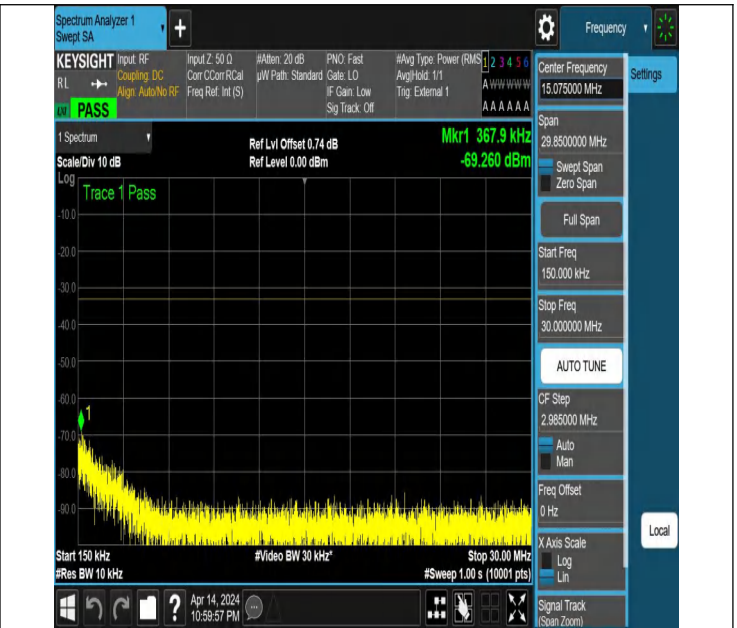
NTNV_N77-3450-3550_PC2_30_40_L_TID2_NS_01_0.15_30_#
