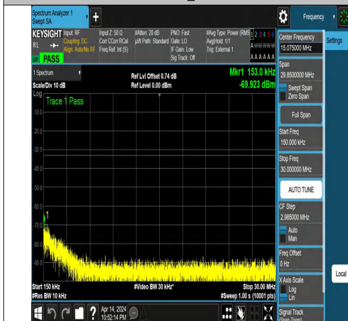
NTNV_N77-3450-3550_PC2_30_30_H_TID6_NS_01_0.15_30_# 1
