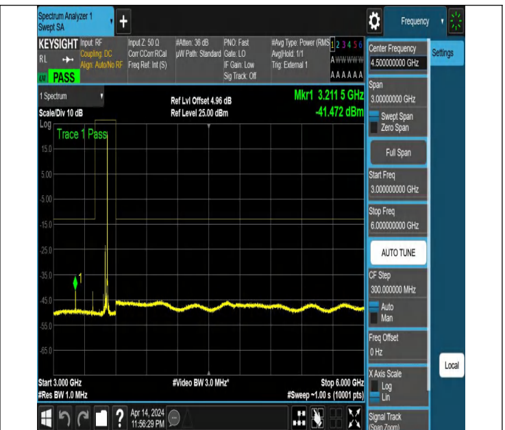
NTNV_N77-3450-3550_PC2_30_40_M_TID6_NS_01_3000_600
