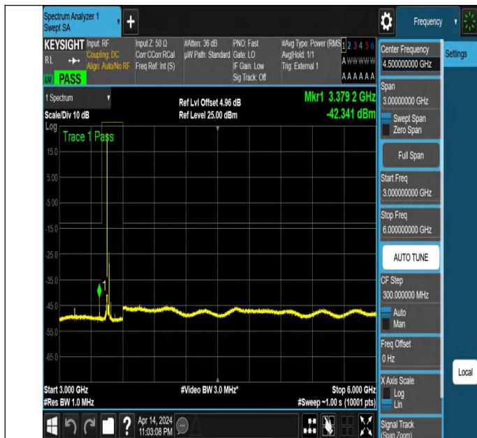
NTNV_N77-3450-3550_PC2_30_40_L_TID2_NS_01_3000_6000
