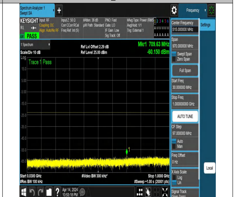
NTNV_N77-3450-3550_PC2_30_30_H_TID6_NS_01_30_1000_#
