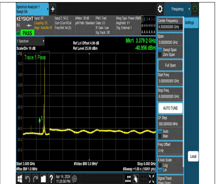
NTNV_N77-3450-3550_PC2_30_40_L_TID6_NS_01_3000_6000
