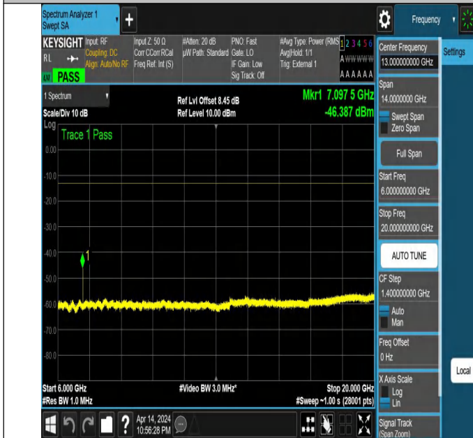
NTNV_N77-3450-3550_PC2_30_30_H_TID6_NS_01_6000_2000
