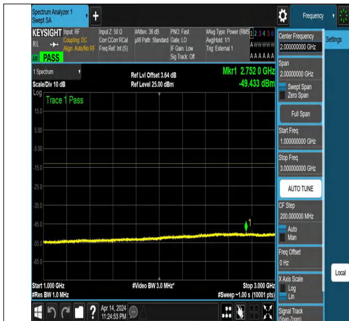
NTNV_N77-3450-3550_PC2_30_40_L_TID6 NS_01_1000_3000
