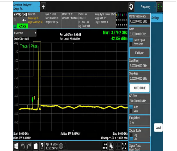
NTNV_N77-3450-3550_PC2_30_30_H_TID6_NS_01_3000_6000
