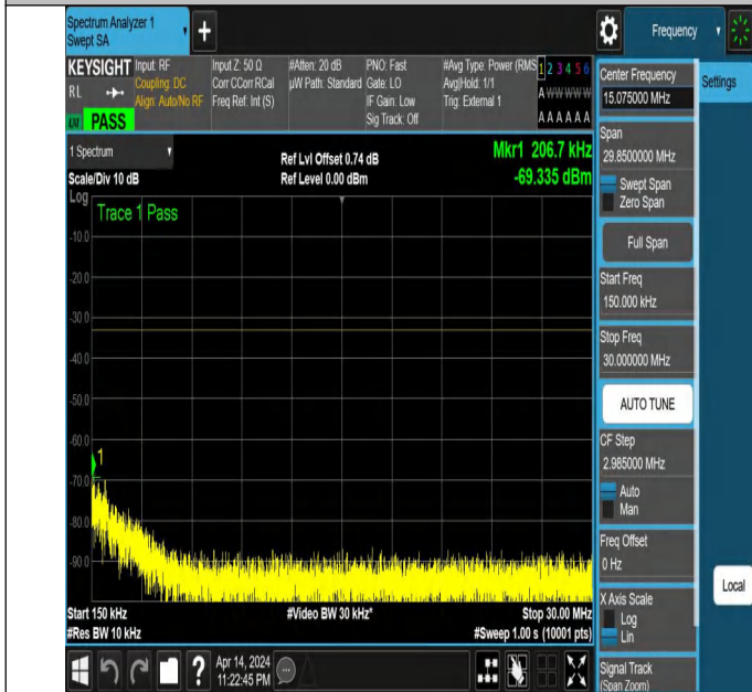
NTNV_N77-3450-3550_PC2_30_40_L_TID6_NS_01_0.15_30_#
