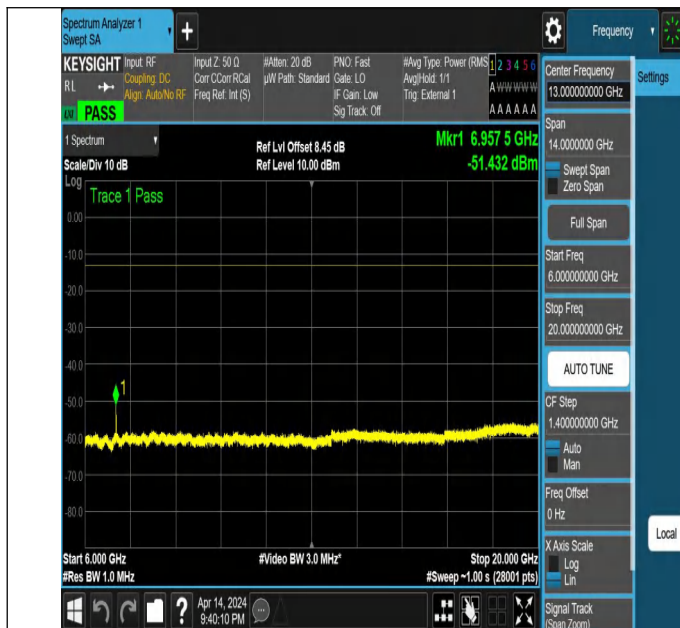
NTNV_N77-3450-3550_PC2_30_30_L_TID3_NS_01_6000_2000
