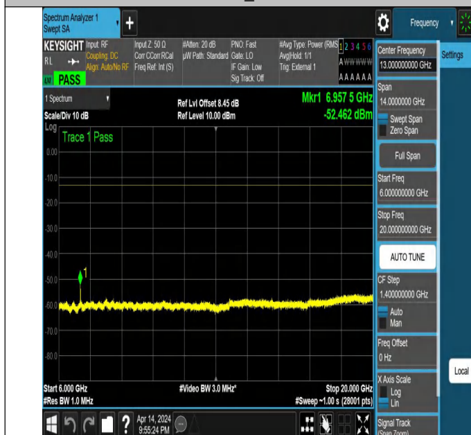
NTNV_N77-3450-3550_PC2_30_30_L_TID6_NS_01_6000_2000
