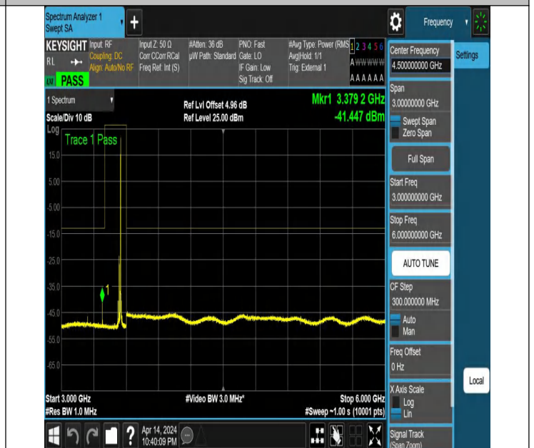
NTNV_N77-3450-3550_PC2_30_30_H_TID3_NS_01_3000_6000
