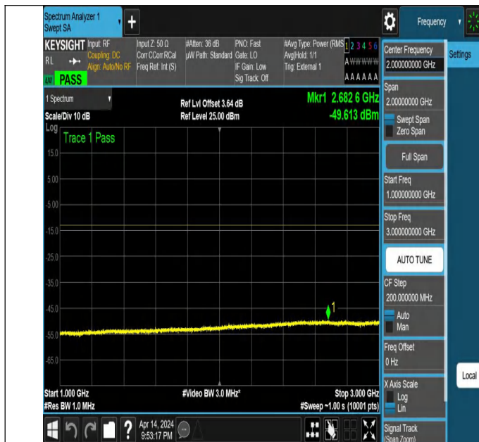
NTNV_N77-3450-3550_PC2_30_30_L_TID6 NS_01_1000_3000
