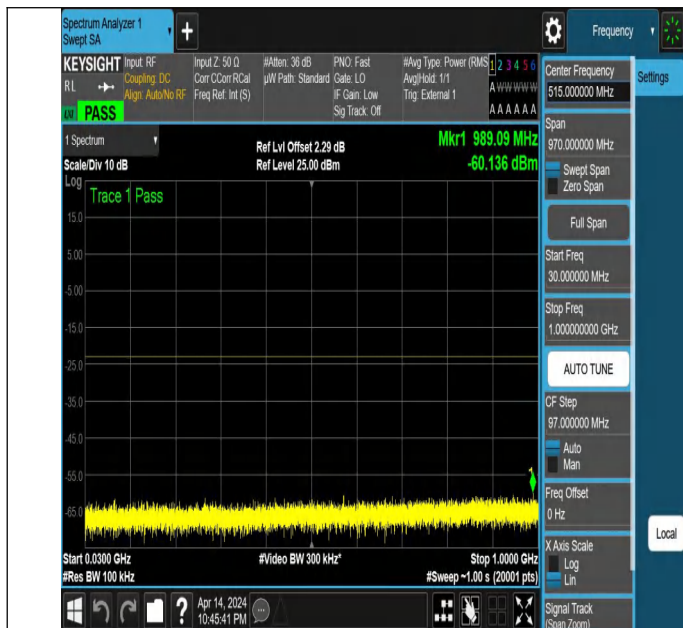
NTNV_N77-3450-3550_PC2_30_30_H_TID5 NS_01_30_1000_#
