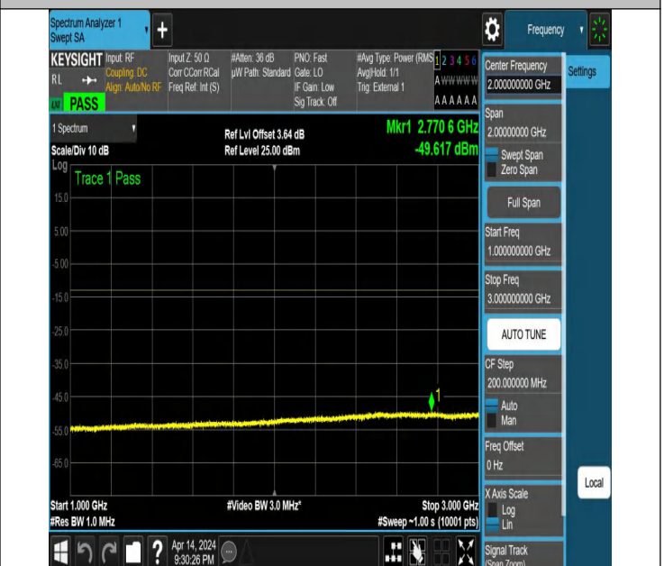
NTNV_N77-3450-3550_PC2_30_30_L_TID2_NS_01_1000_3000
