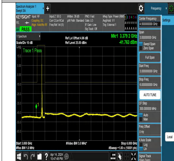
NTNV_N77-3450-3550_PC2_30_30_H_TID5_NS_01_3000_6000
