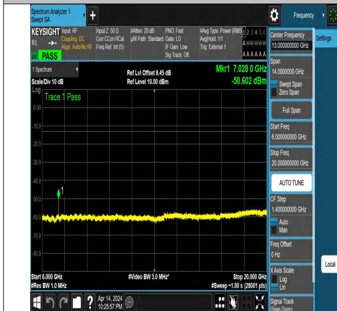
NTNV_N77-3450-3550_PC2_30_30_M_TID6_NS_01_6000_200
