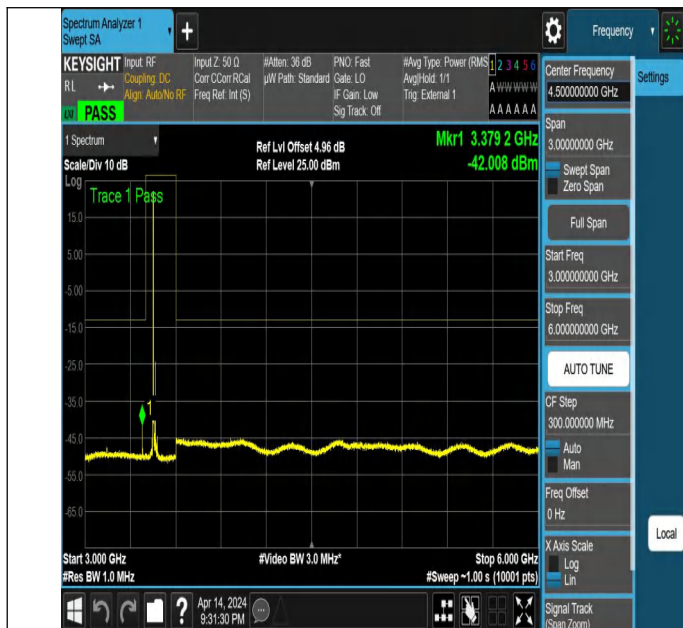
NTNV_N77-3450-3550_PC2_30_30_L_TID2_NS_01_3000_6000
