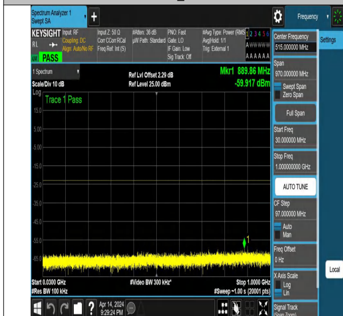
NTNV_N77-3450-3550_PC2_30_30_L_TID2_NS_01_30_1000_#
