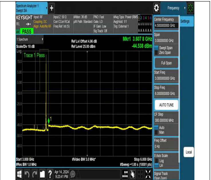
NTNV_N77-3450-3550_PC2_30_20_H_TID6_NS_01_3000_6000
