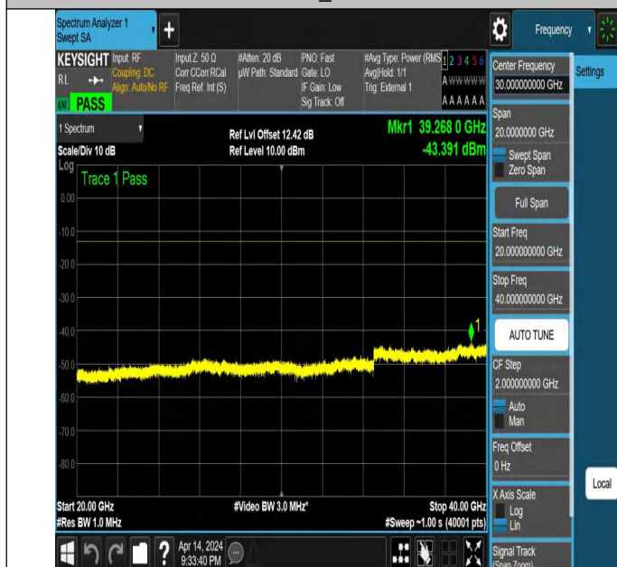
NTNV_N77-3450-3550_PC2_30_30_L_TID2_NS_01_20000_400
