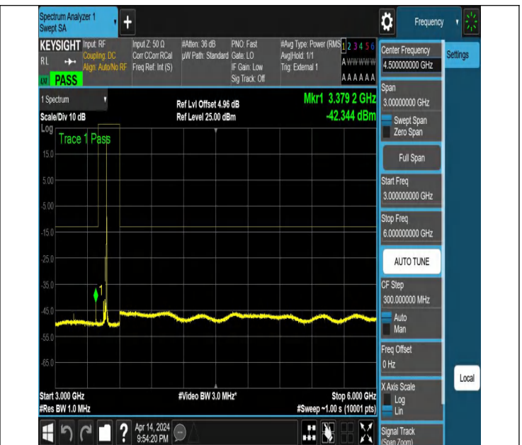
NTNV_N77-3450-3550_PC2_30_30_L_TID6_NS_01_3000_6000
