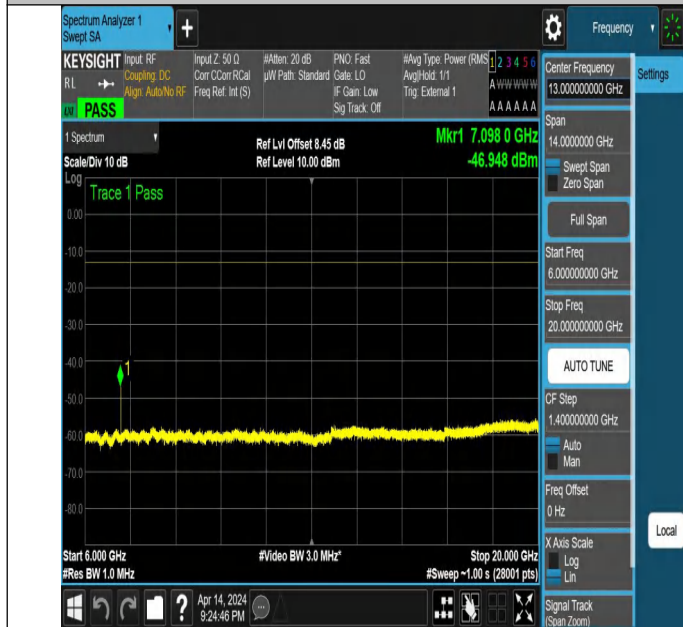
NTNV_N77-3450-3550_PC2_30_20_H_TID6_NS_01_6000_2000
