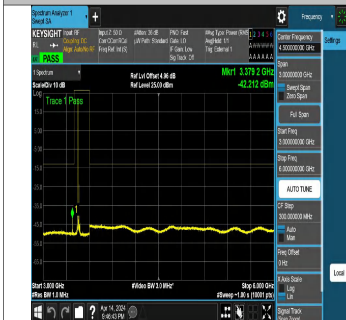
NTNV_N77-3450-3550_PC2_30_30_L_TID5_NS_01_3000_6000
