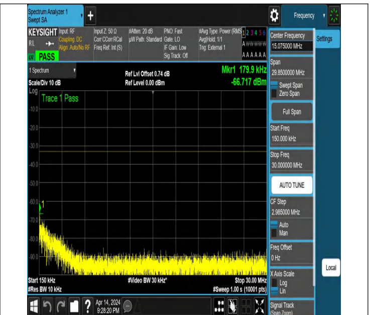
NTNV_N77-3450-3550_PC2_30_30_L_TID2_NS_01_0.15_30_#
