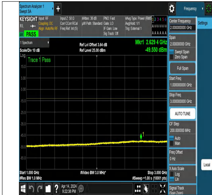
NTNV_N77-3450-3550_PC2_30_20_H_TID6_NS_01_1000_3000
