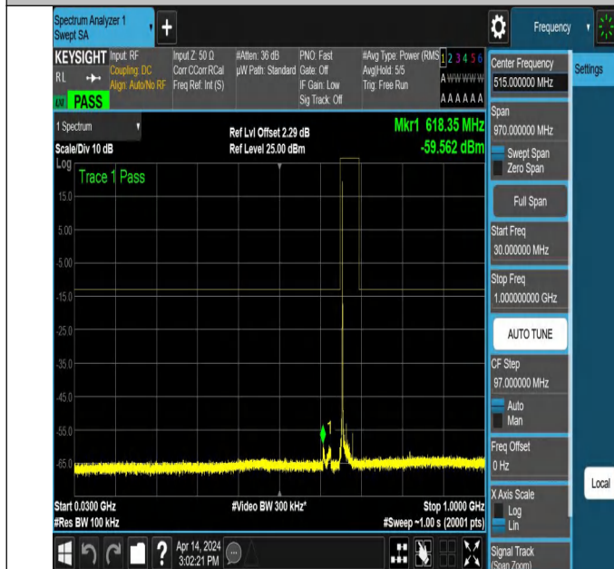
NTNV_N71_PC3_15_20_L_TID2_NS_01_30_1000_#1
