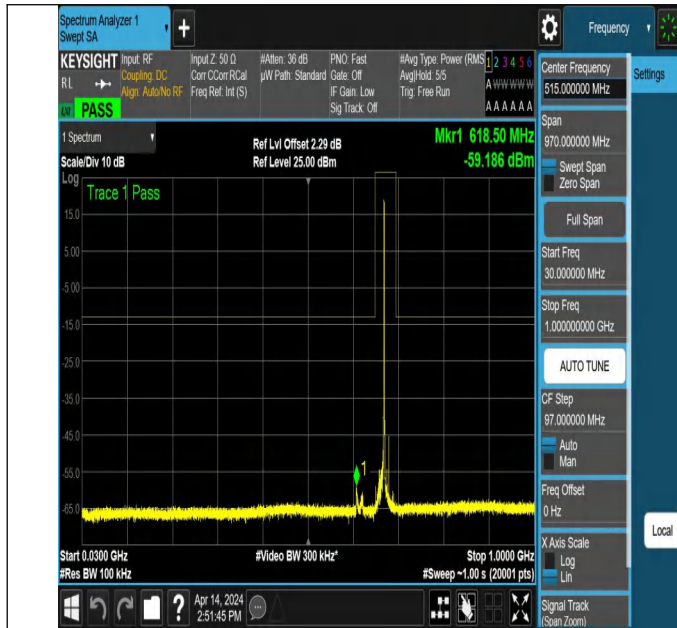
NTNV_N71_PC3_15_15_L_TID6_NS_01_30_1000_#1
