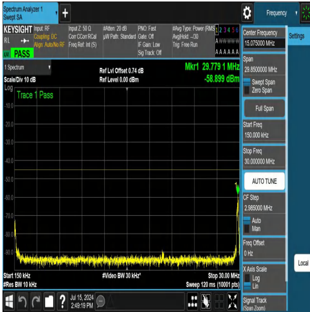
NTNV-N41-PC3-30-100-H-DFT-QPSK-Edge_1RB_Left-0.15-30-A nt1-PASS
