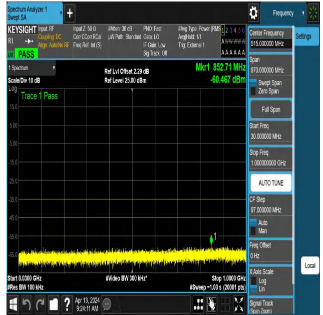
NTNV-N41-PC3-30-100-M-DFT-QPSK-Edge_1RB_Left-30-1000- Ant1-PASS
