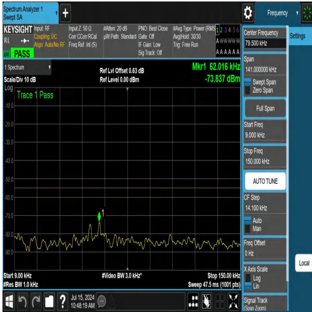
NTNV-N41-PC3-30-30-M-DFT-PI2BPSK-Edge_1RB_Left-0.009-0. 15-Ant1-PASS
