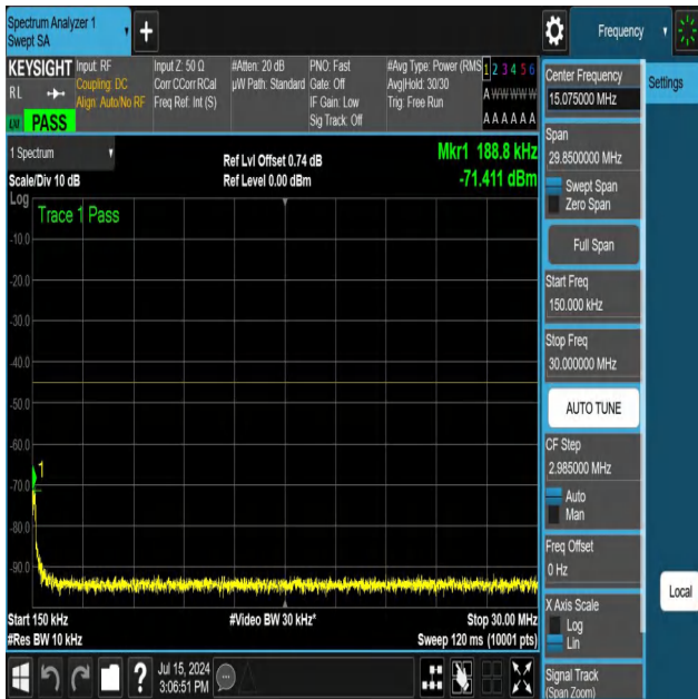
NTNV-N41-PC3-30-30-M-DFT-QPSK-Edge_1RB_Right-0.15-30-A nt1-PASS
