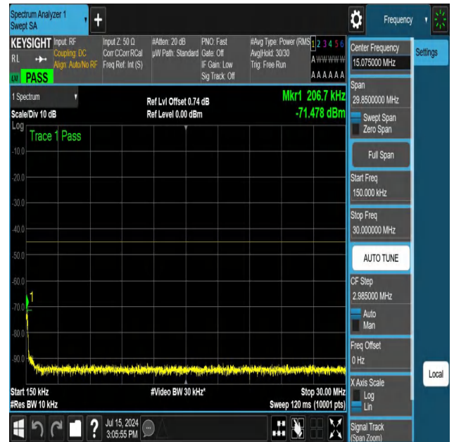
NTNV-N41-PC3-30-30-L-DFT-QPSK-Edge_1RB_Right-0.15-30-A nt1-PASS
