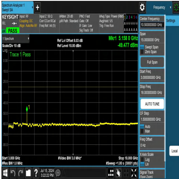
NTNV-N41-PC3-30-30-M-DFT-QPSK-Edge_1RB_Left-3000-1800 0-Ant1-PASS
