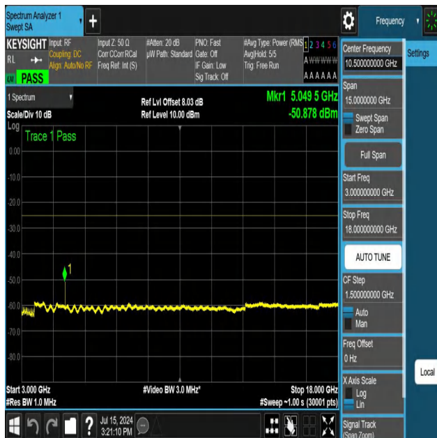
NTNV-N41-PC3-30-30-L-DFT-QPSK-Edge_1RB_Right-3000-1800 0-Ant1-PASS
