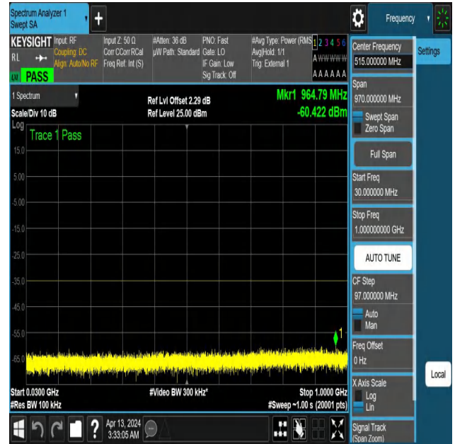
NTNV-N41-PC3-30-30-H-DFT-QPSK-Edge_1RB_Left-30-1000-A nt1-PASS
