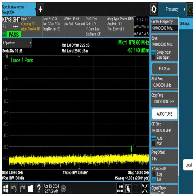
NTNV-N41-PC3-30-30-L-DFT-QPSK-Edge_1RB_Left-30-1000-Ant 1-PASS
