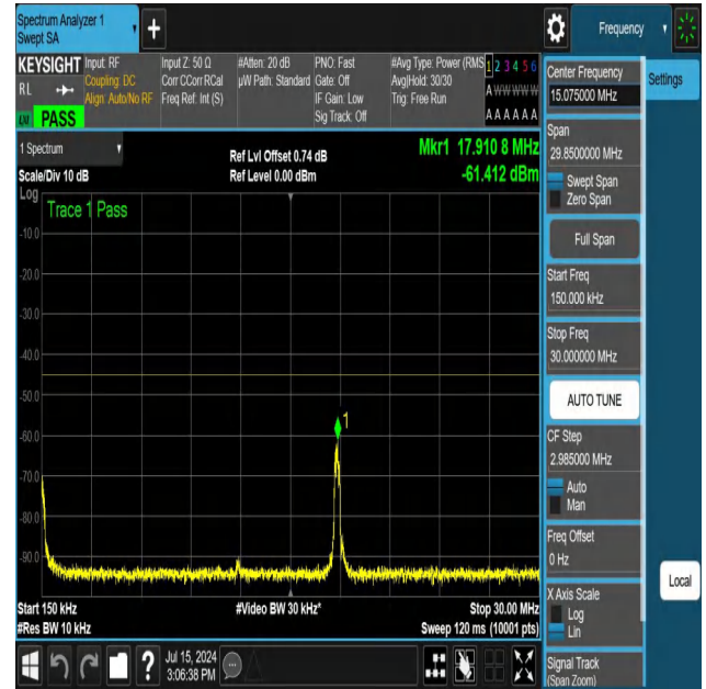
NTNV-N41-PC3-30-30-M-DFT-QPSK-Edge_1RB_Left-0.15-30-Ant1-PASS
