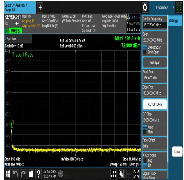
NTNV-N41-PC3-30-30-L-DFT-QPSK-Edge_1RB_Left-0.15-30-An t1-PASS
