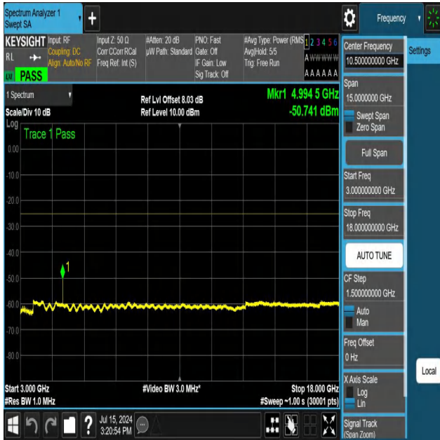
NTNV-N41-PC3-30-30-L-DFT-QPSK-Edge_1RB_Left-3000-18000 -Ant1-PASS
