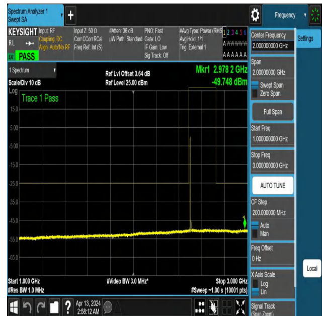
NTNV-N41-PC3-30-30-L-DFT-QPSK-Edge_1RB_Left-1000-3000- Ant1-PASS
