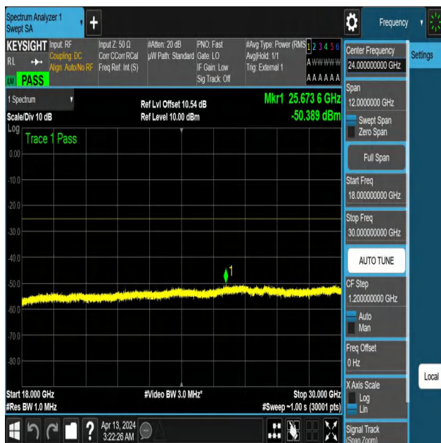
NTNV-N41-PC3-30-30-M-DFT-QPSK-Edge_1RB_Right-18000-30 000-Ant1-PASS
