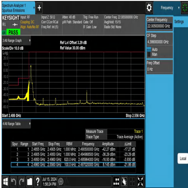
NTNV-N41-PC3-30-60-L-DFT-QPSK-Edge_1RB_Left-Ant1-PASS
