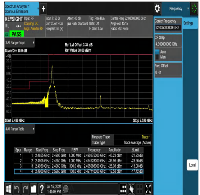
NTNV-N41-PC3-30-30-L-DFT-QPSK-Edge_1RB_Left-Ant1-PASS
