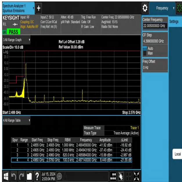
NTNV-N41-PC3-30-80-L-DFT-QPSK-Edge_1RB_Left-Ant1-PASS
