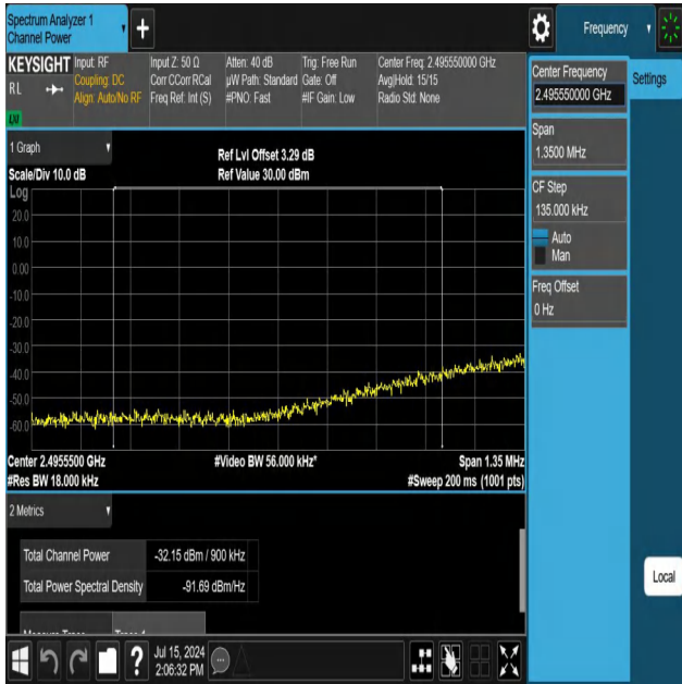
NTNV-N41-PC3-30-90-L-DFT-QPSK-Edge_1RB_Left-Ant1-PASS
