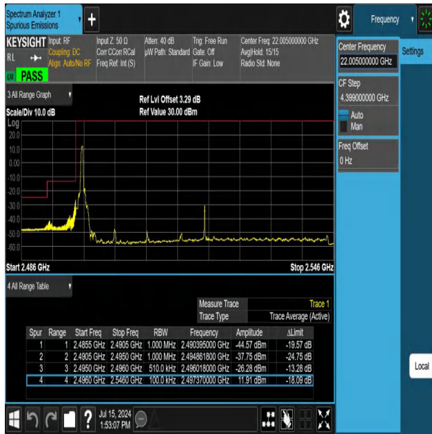
NTNV-N41-PC3-30-50-L-DFT-QPSK-Edge_1RB_Left-Ant1-PASS
