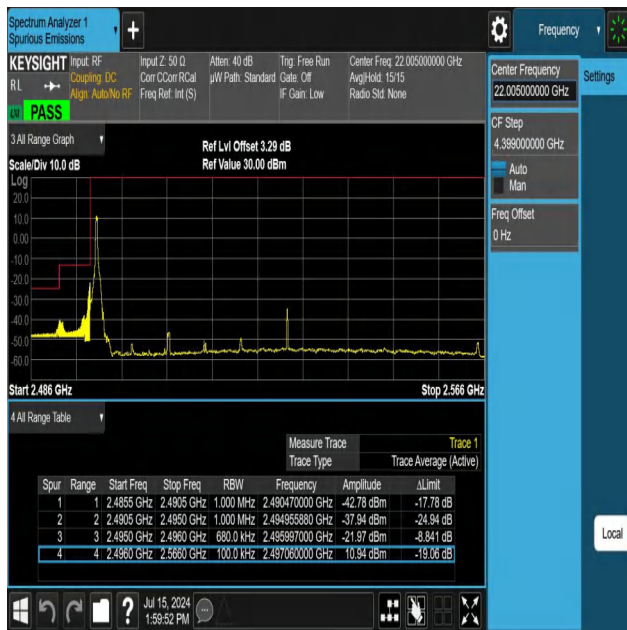
NTNV-N41-PC3-30-70-L-DFT-QPSK-Edge_1RB_Left-Ant1-PASS
