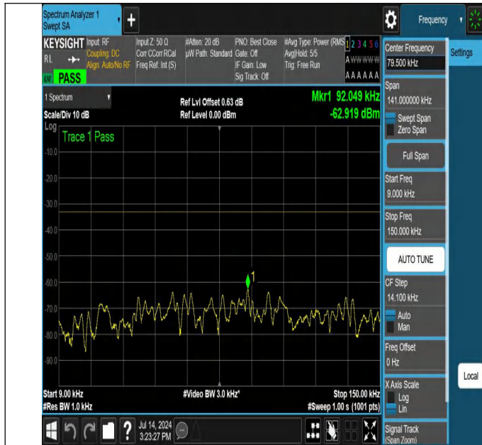
NTNV-N26-824-849-PC3-15-10-L-DFT-QPSK-Edge_1RB_Left-0.
