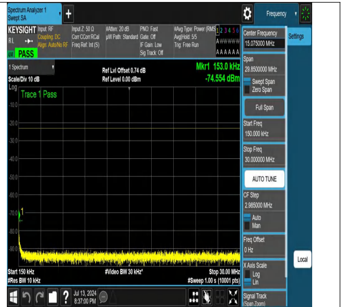
NTNV-N26-824-849-PC3-15-10-M-DFT-QPSK-Edge_1RB_Left-0. 15-30-Ant1-PASS
