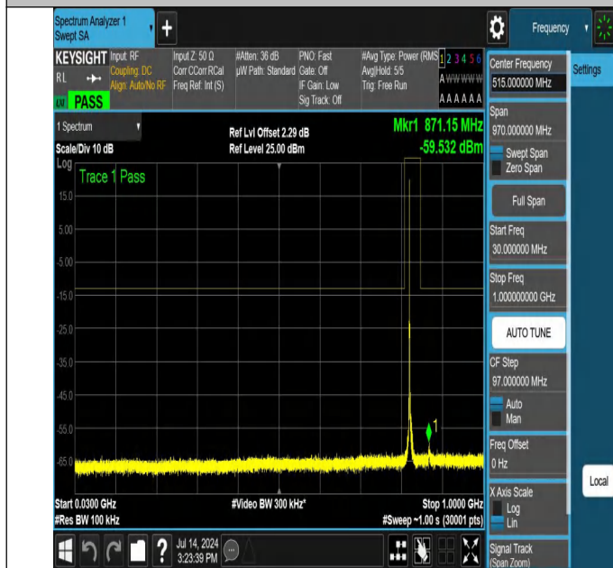
NTNV-N26-824-849-PC3-15-10-L-DFT-QPSK-Edge_1RB_Left-30
