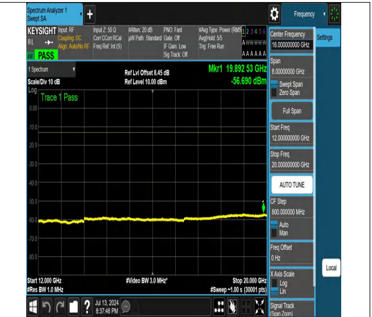
NTNV-N26-824-849-PC3-15-10-M-DFT-QPSK-Edge_1RB_Left-12 000-20000-Ant1-PASS
