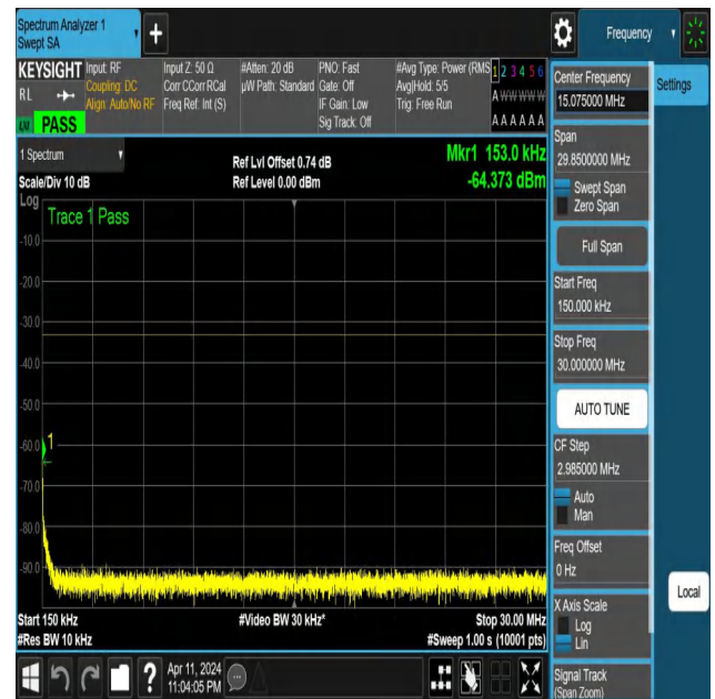
NTNV-N25-PC3-15-20-L-DFT-QPSK-Edge_1RB_Right-0.15-30-A nt1-PASS
