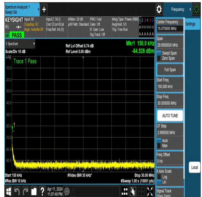
NTNV-N25-PC3-15-20-M-DFT-QPSK-Edge_1RB_Right-0.15-30-A nt1-PASS
