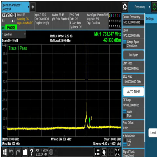
NTNV-N12-PC3-15-10-M-DFT-QPSK-Edge_1RB_Left-30-1000-A nt1-PASS
