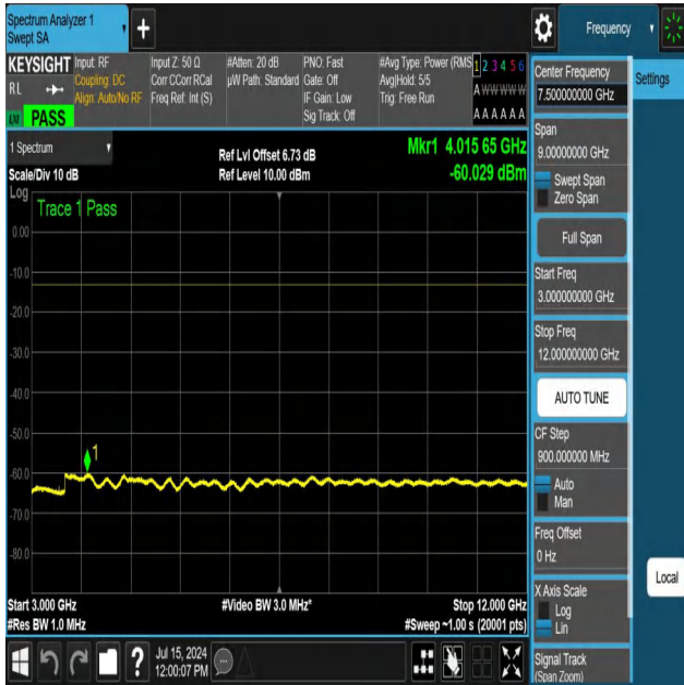
NTNV-N12-PC3-15-15-L-DFT-QPSK-Edge_1RB_Left-3000-1200 0-Ant1-PASS
