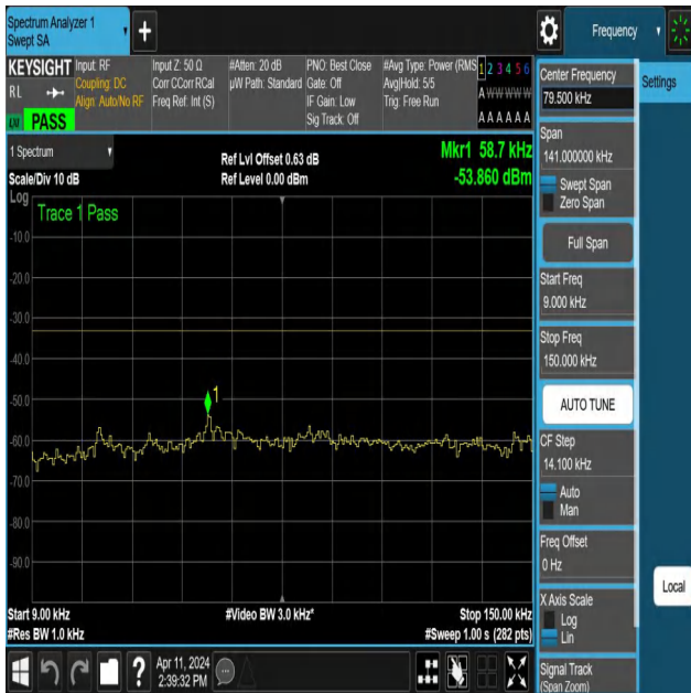
NTNV-N12-PC3-15-10-M-DFT-QPSK-Edge_1RB_Right-0.009-0. 15-Ant1-PASS
