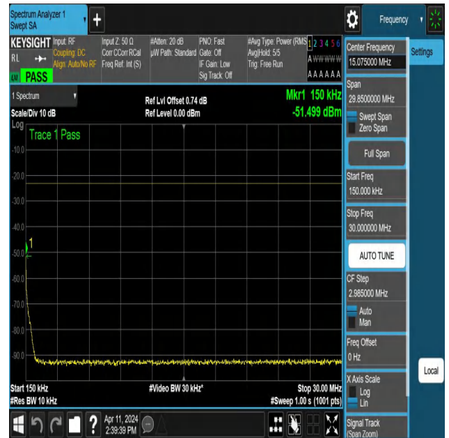
NTNV-N12-PC3-15-10-M-DFT-QPSK-Edge_1RB_Right-0.15-30-A nt1-PASS
