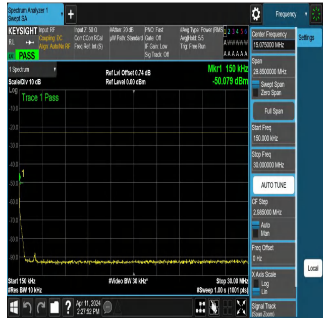
NTNV-N12-PC3-15-5-M-DFT-QPSK-Edge_1RB_Left-0.15-30-Ant1 -PASS
