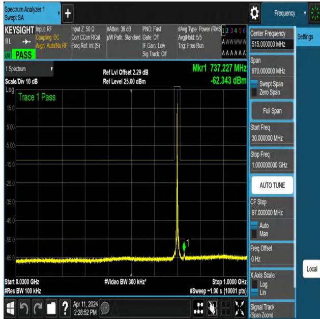
NTNV-N12-PC3-15-5-M-DFT-QPSK-Edge_1RB_Right-30-1000-A nt1-PASS
