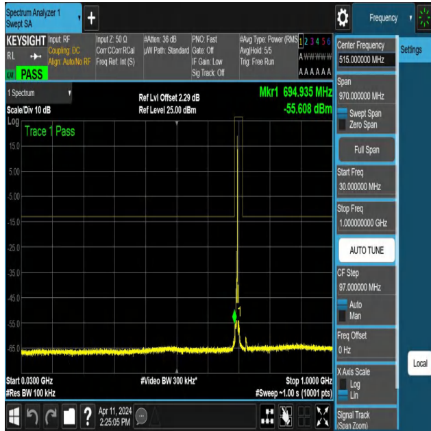
NTNV-N12-PC3-15-5-L-DFT-QPSK-Edge_1RB_Right-30-1000-A nt1-PASS
