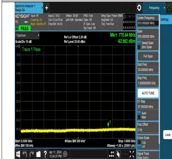
NTNV-N7-PC3-15-40-L-DFT-QPSK-Edge_1RB_Left-30-1000-Ant1-PASS
