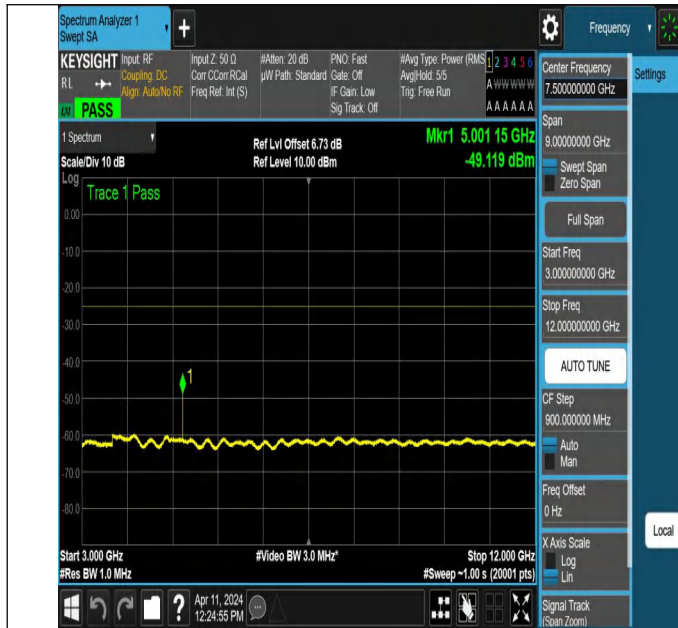
NTNV-N7-PC3-15-40-L-DFT-QPSK-Edge_1RB_Left-3000-12000- Ant1-PASS
