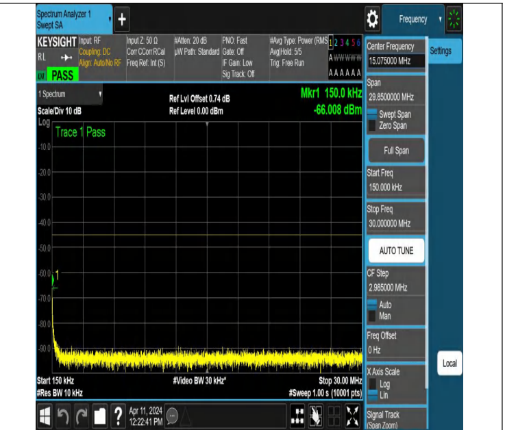
NTNV-N7-PC3-15-40-L-DFT-PI2BPSK-Edge_1RB_Left-0.15-30-A nt1-PASS
