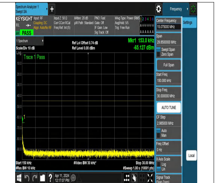
NTNV-N7-PC3-15-30-M-DFT-QPSK-Edge_1RB_Left-0.15-30-Ant1 -PASS
