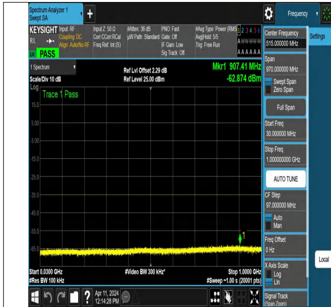
NTNV-N7-PC3-15-30-L-DFT-QPSK-Edge_1RB_Right-30-1000-A nt1-PASS
