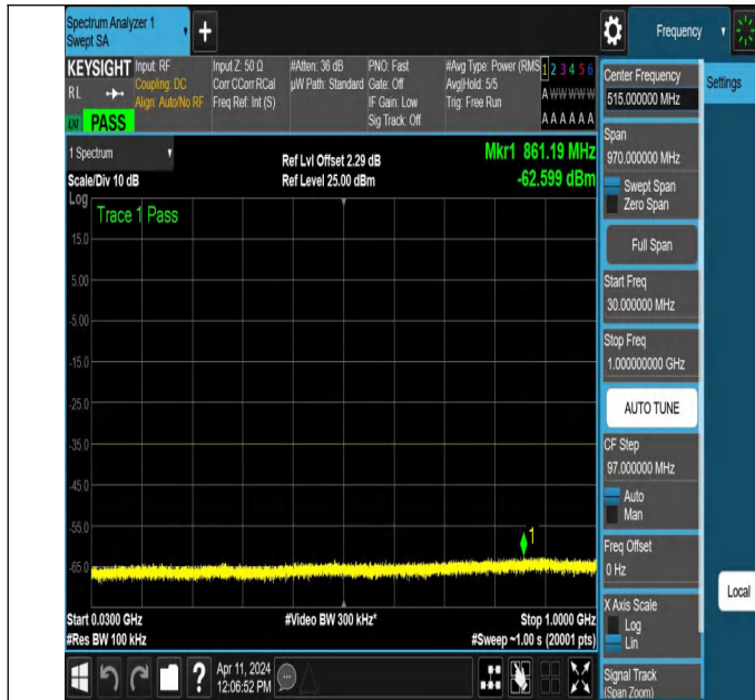
NTNV-N7-PC3-15-25-M-DFT-QPSK-Edge_1RB_Right-30-1000-A nt1-PASS
