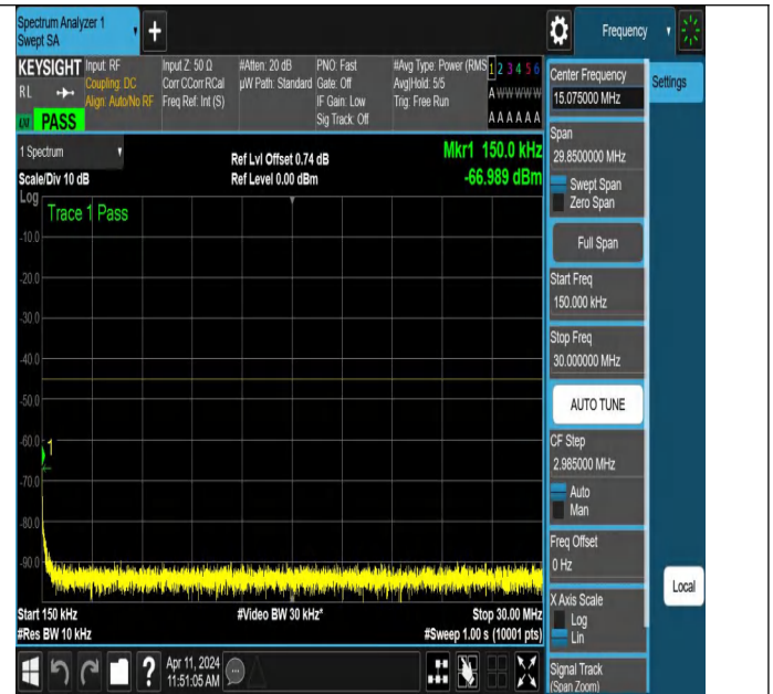
NTNV-N7-PC3-15-20-L-DFT-QPSK-Edge_1RB_Left-0.15-30-Ant1-PASS
