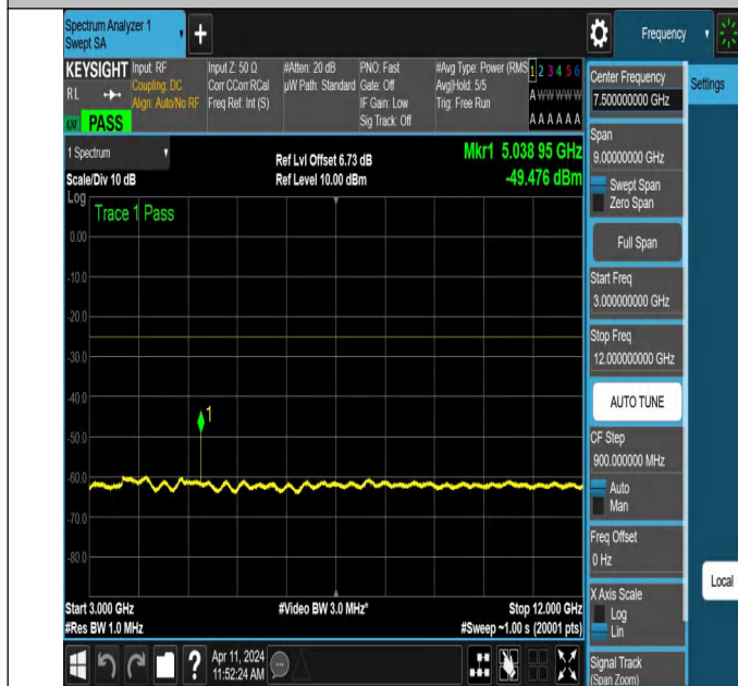
NTNV-N7-PC3-15-20-L-DFT-QPSK-Edge_1RB_Right-3000-1200 0-Ant1-PASS
