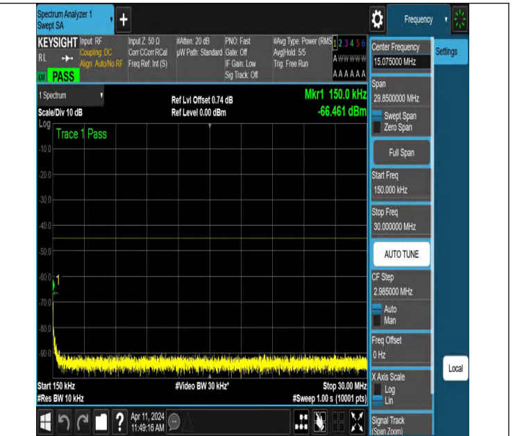
NTNV-N7-PC3-15-20-L-DFT-PI2BPSK-Edge_1RB_Left-0.15-30-A nt1-PASS
