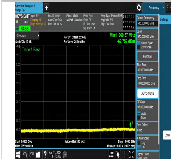
NTNV-N7-PC3-15-20-L-DFT-QPSK-Edge_1RB_Left-30-1000-Ant1-PASS
