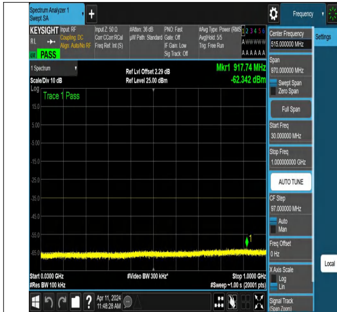
NTNV-N7-PC3-15-15-H-DFT-QPSK-Edge_1RB_Right-30-1000-A nt1-PASS
