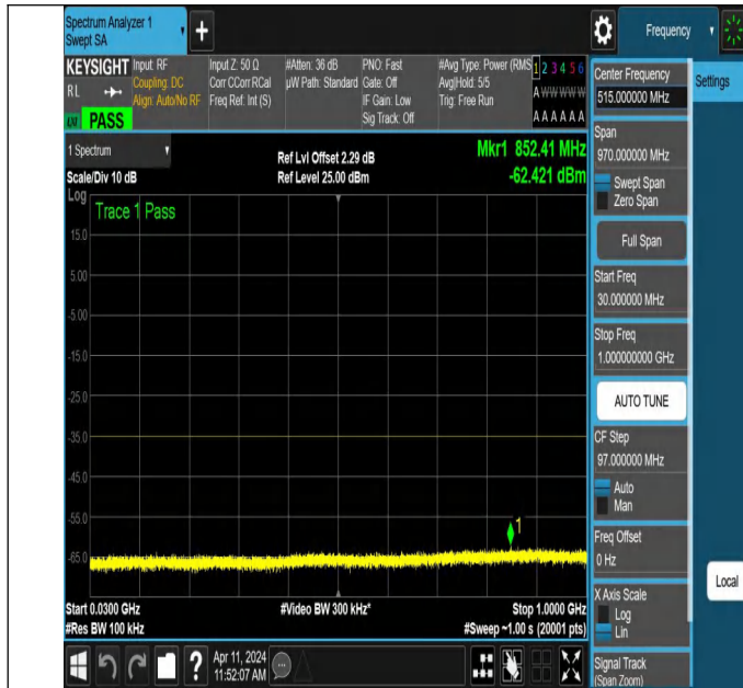
NTNV-N7-PC3-15-20-L-DFT-QPSK-Edge_1RB_Right-30-1000-A nt1-PASS
