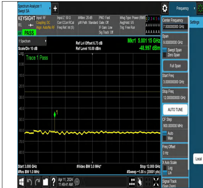
NTNV-N7-PC3-15-20-L-DFT-PI2BPSK-Edge_1RB_Left-3000-120 00-Ant1-PASS
