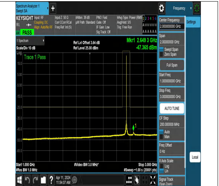
NTNV-N7-PC3-15-20-M-DFT-PI2BPSK-Edge_1RB_Right-1000-30 00-Ant1-PASS
