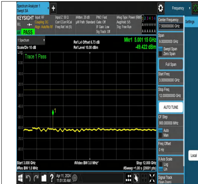
NTNV-N7-PC3-15-20-L-DFT-QPSK-Edge_1RB_Left-3000-12000- Ant1-PASS
