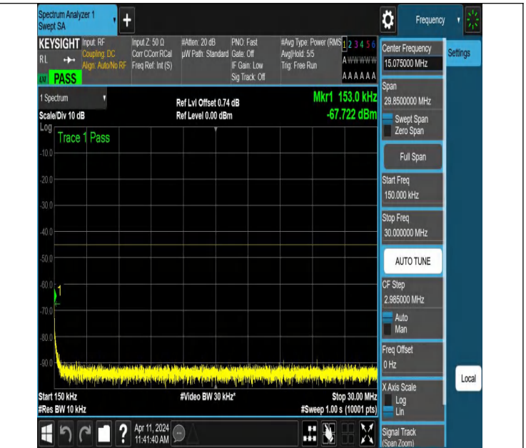
NTNV-N7-PC3-15-15-M-DFT-PI2BPSK-Edge_1RB_Left-0.15-30-A nt1-PASS
