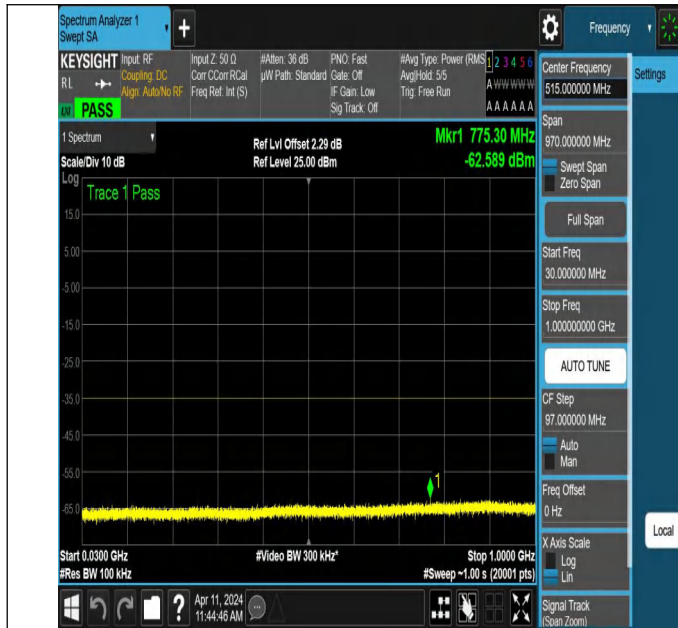
NTNV-N7-PC3-15-15-M-DFT-QPSK-Edge_1RB_Right-30-1000-A nt1-PASS
