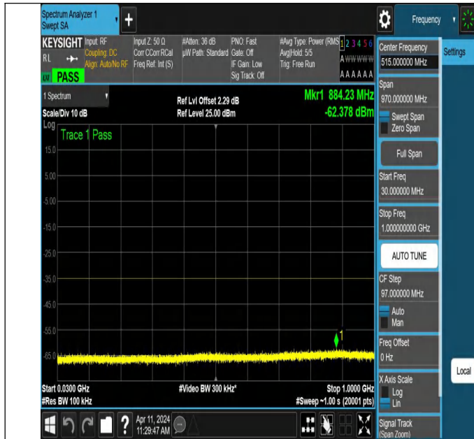
NTNV-N7-PC3-15-10-L-DFT-QPSK-Edge_1RB_Right-30-1000-A nt1-PASS
