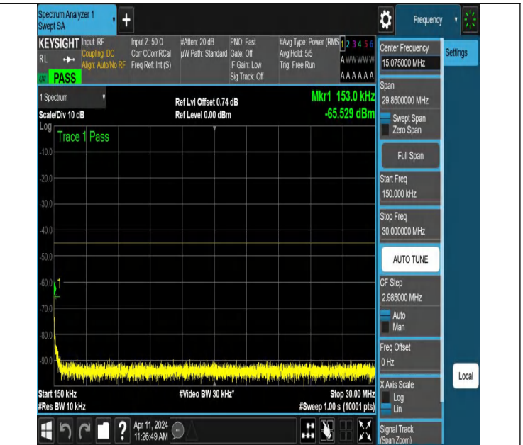
NTNV-N7-PC3-15-10-L-DFT-PI2BPSK-Edge_1RB_Left-0.15-30-A nt1-PASS
