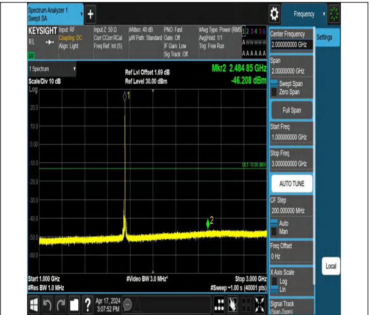
66-66-20MHz-20MHz-QPSK-QPSK-132323-132521-1RB#99-0RB B#0-1000~3000MHz-PASS
