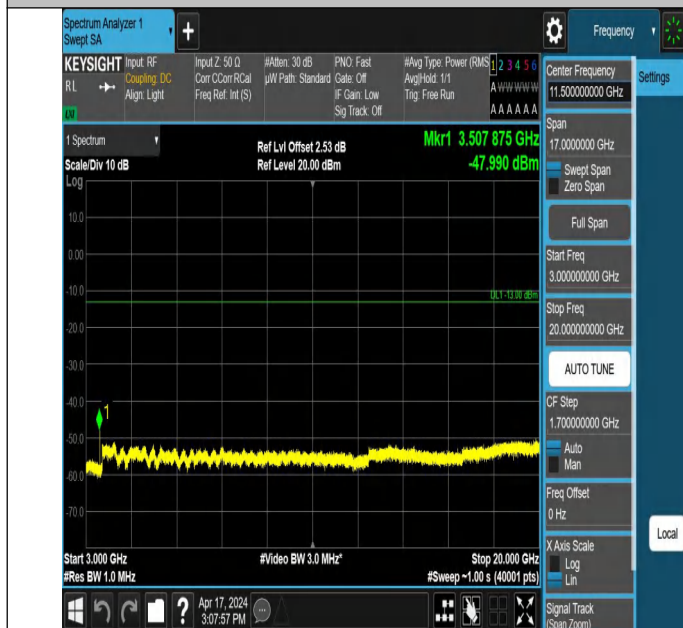
66-66-20MHz-20MHz-QPSK-QPSK-132323-132521-1RB#99-0RB #0-3000~20000MHz-PASS
