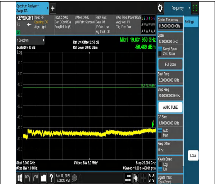
66-66-20MHz-20MHz-QPSK-QPSK-132323-132521-1RB#0-1RB #99-3000~20000MHz-PASS
