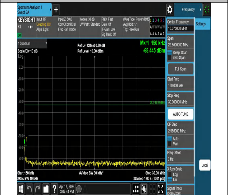
66-66-20MHz-20MHz-QPSK-QPSK-132323-132521-1RB#99-0R B#0-0.15~30MHz-PASS
