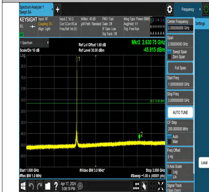
66-66-20MHz-20MHz-QPSK-QPSK-132072-132270-1RB#99-0RB #0-1000~3000MHz-PASS
