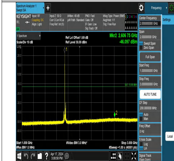
66-66-20MHz-20MHz-QPSK-QPSK-132374-132572-1RB#0-0RB# 0-1000~3000MHz-PASS
