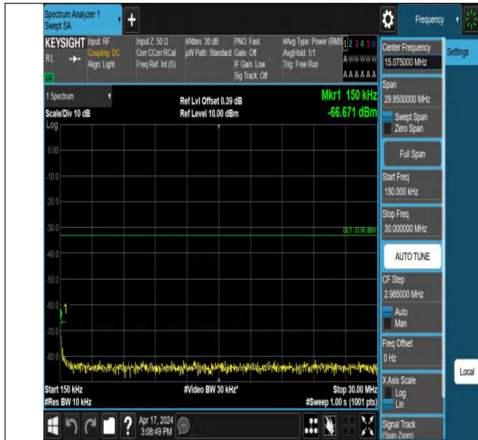
66-66-20MHz-20MHz-QPSK-QPSK-132374-132572-1RB#0-0RB# 0-0.15~30MHz-PASS
