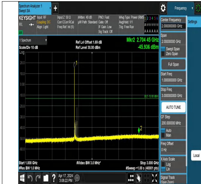
66-66-20MHz-20MHz-QPSK-QPSK-132323-132521-1RB#0-1RB# 99-1000~3000MHz-PASS
