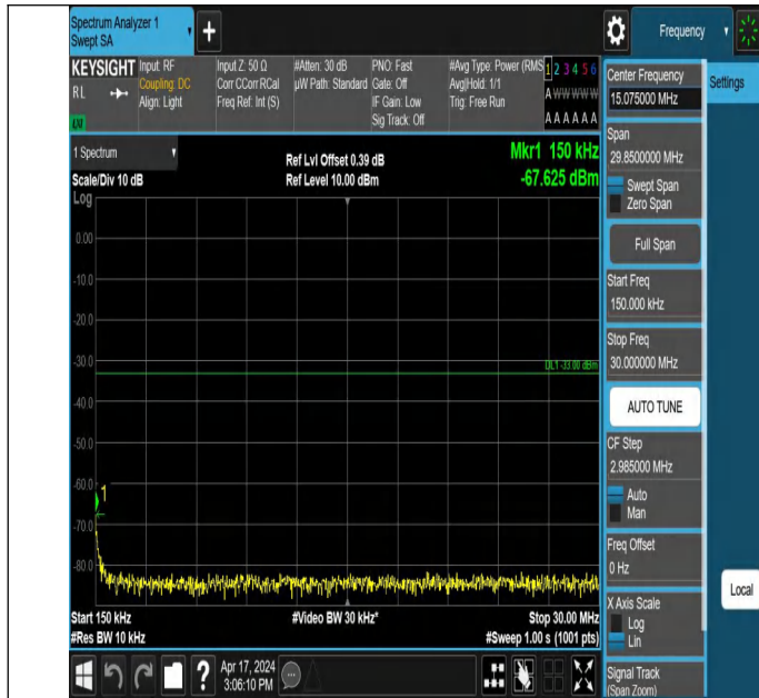
66-66-20MHz-20MHz-QPSK-QPSK-132072-132270-1RB#99-0RB #0-0.15~30MHz-PASS
