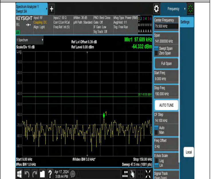
66-66-20MHz-20MHz-QPSK-QPSK-132374-132572-1RB#0-0RB #0-0.009~0.15MHz-PASS
