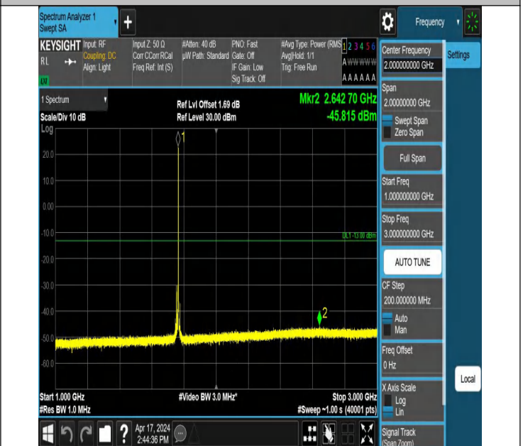
66-66-20MHz-15MHz-QPSK-QPSK-132423-132594-1RB#99-0RB B#0-1000~3000MHz-PASS
