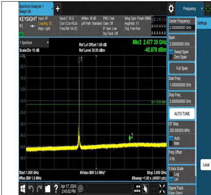
66-66-20MHz-15MHz-QPSK-QPSK-132348-132519-1RB#99-0RB #0-1000~3000MHz-PASS
