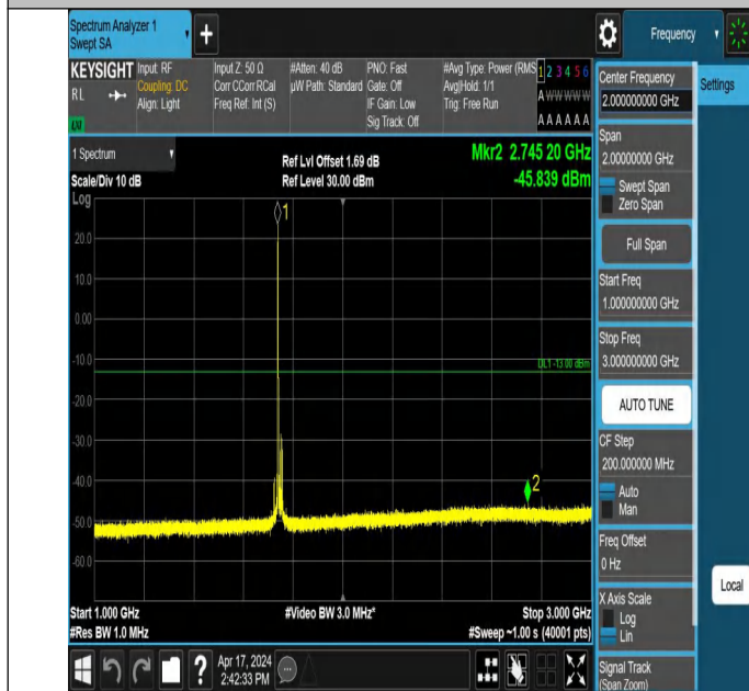
66-66-20MHz-15MHz-QPSK-QPSK-132348-132519-1RB#0-0RB# 0-1000~3000MHz-PASS
