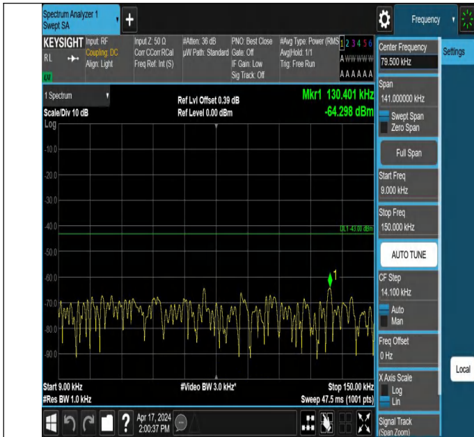
66-66-20MHz-10MHz-QPSK-QPSK-132373-132517-1RB#99-0RB #0-0.009~0.15MHz-PASS
