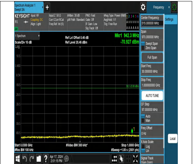
66-66-20MHz-10MHz-QPSK-QPSK-132373-132517-1RB#0-1RB #49-30~1000MHz-PASS
