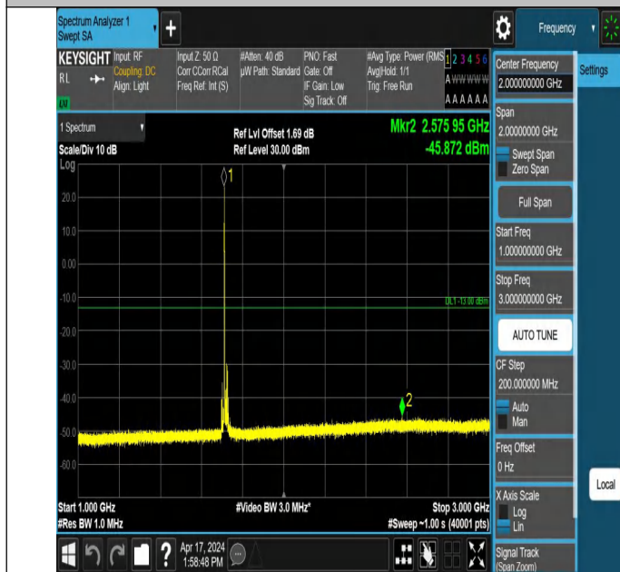
66-66-20MHz-10MHz-QPSK-QPSK-132072-132216-1RB#0-0RB# 0-1000~3000MHz-PASS
