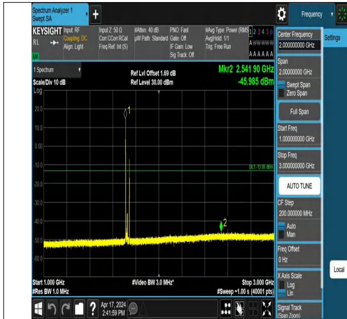
66-66-20MHz-15MHz-QPSK-QPSK-132072-132243-1RB#0-1RB# 74-1000~3000MHz-PASS
