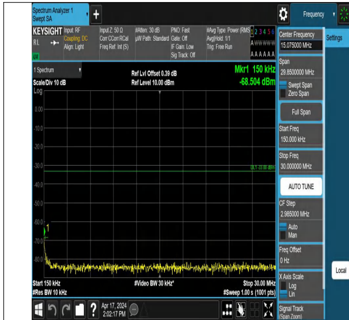
66-66-20MHz-10MHz-QPSK-QPSK-132473-132617-1RB#99-0RB #0-0.15~30MHz-PASS
