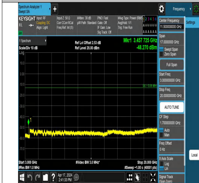
66-66-20MHz-15MHz-QPSK-QPSK-132072-132243-1RB#99-0RB #0-3000~20000MHz-PASS
