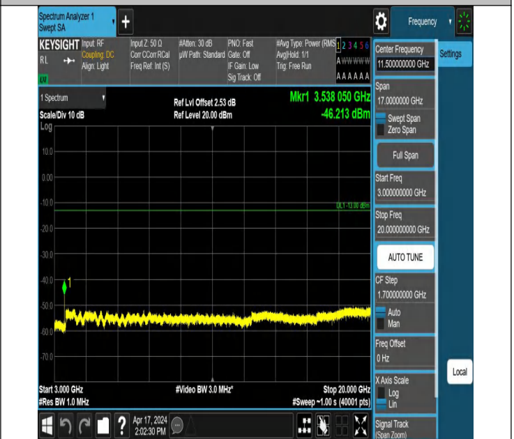
66-66-20MHz-10MHz-QPSK-QPSK-132473-132617-1RB#99-0RB B#0-3000~20000MHz-PASS
