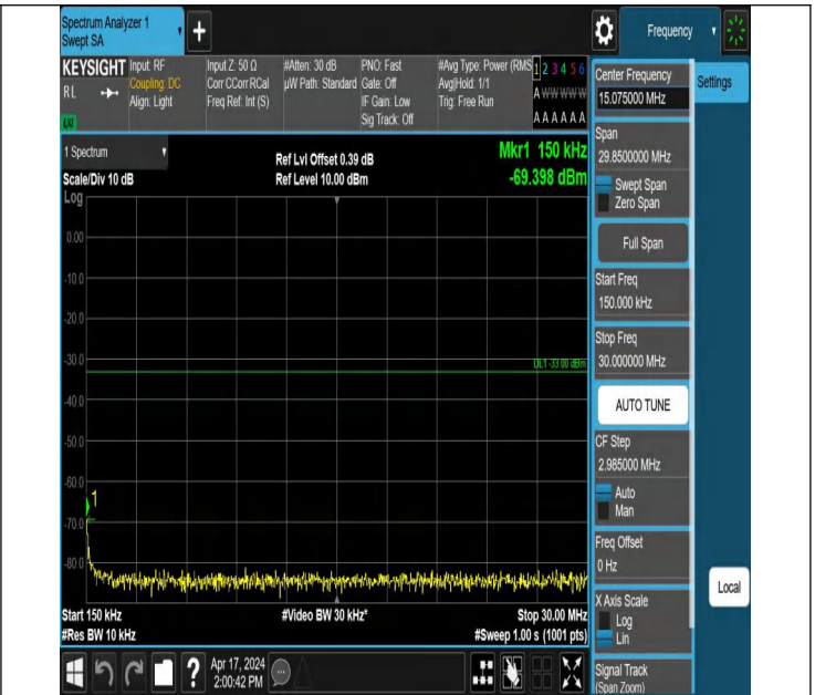
66-66-20MHz-10MHz-QPSK-QPSK-132373-132517-1RB#99-0RB B#0-0.15~30MHz-PASS
