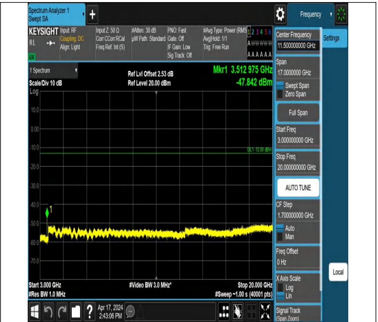
66-66-20MHz-15MHz-QPSK-QPSK-132348-132519-1RB#99-0R B#0-3000~20000MHz-PASS
