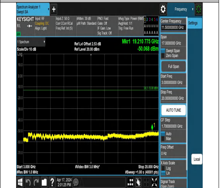
66-66-20MHz-10MHz-QPSK-QPSK-132373-132517-1RB#0-1RB #49-3000~20000MHz-PASS
