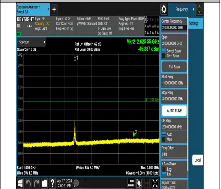
66-66-20MHz-10MHz-QPSK-QPSK-132373-132517-1RB#99-0RB B#0-1000~3000MHz-PASS
