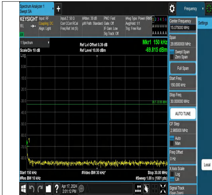
66-66-20MHz-10MHz-QPSK-QPSK-132373-132517-1RB#0-1RB# 49-0.15~30MHz-PASS
