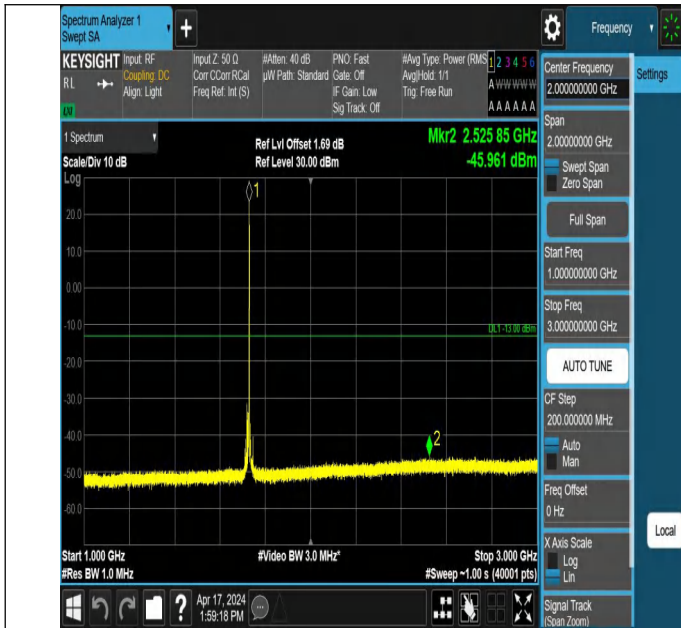
66-66-20MHz-10MHz-QPSK-QPSK-132072-132216-1RB#99-0RB #0-1000~3000MHz-PASS
