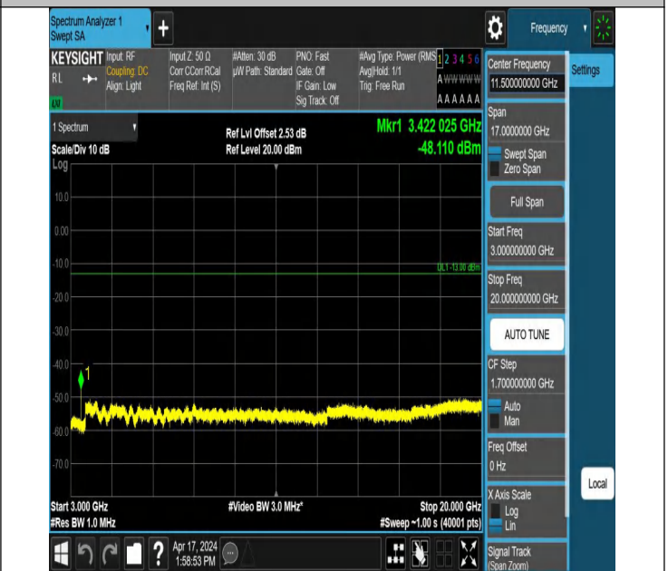
66-66-20MHz-10MHz-QPSK-QPSK-132072-132216-1RB#0-0RB# #0-3000~20000MHz-PASS
