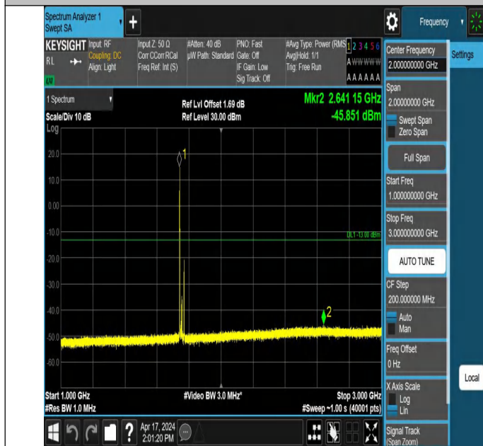
66-66-20MHz-10MHz-QPSK-QPSK-132373-132517-1RB#0-1RB# 49-1000~3000MHz-PASS
