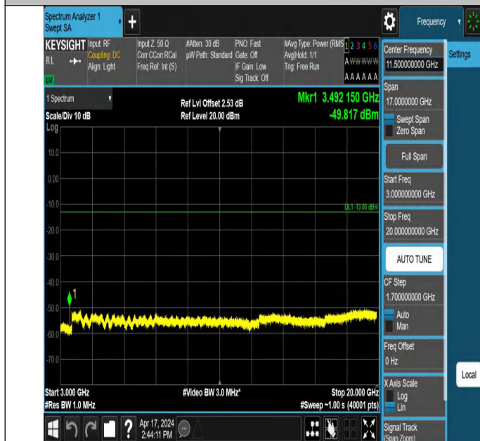
66-66-20MHz-15MHz-QPSK-QPSK-132423-132594-1RB#0-0RB# 0-3000~20000MHz-PASS
