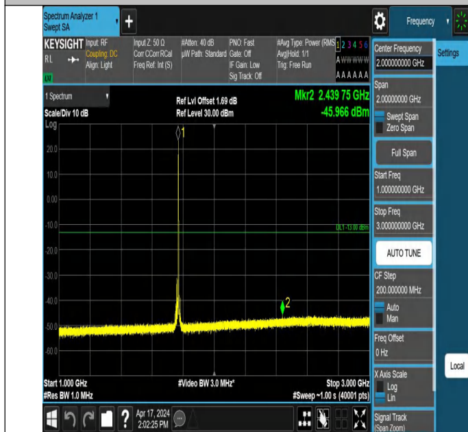
66-66-20MHz-10MHz-QPSK-QPSK-132473-132617-1RB#99-0RB #0-1000~3000MHz-PASS
