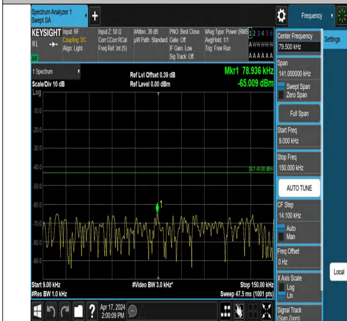
66-66-20MHz-10MHz-QPSK-QPSK-132373-132517-1RB#0-0RB# 0-0.009~0.15MHz-PASS
