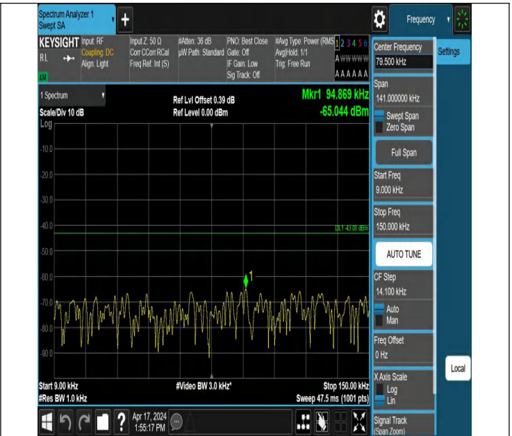
66-66-20MHz-5MHz-QPSK-QPSK-132397-132514-100RB#0-25R B#0-0.009~0.15MHz-PASS
