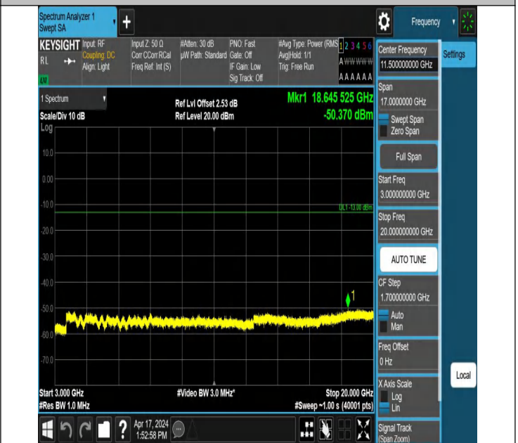
66-66-20MHz-5MHz-QPSK-QPSK-132072-132189-1RB#0-1RB# 24-3000~20000MHz-PASS
