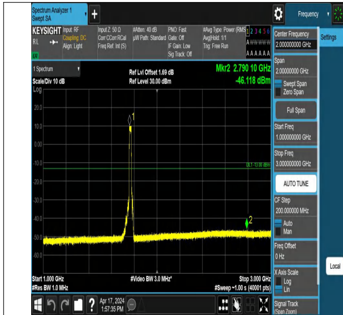
66-66-20MHz-5MHz-QPSK-QPSK-132522-132639-100RB#0-25R B#0-1000~3000MHz-PASS
