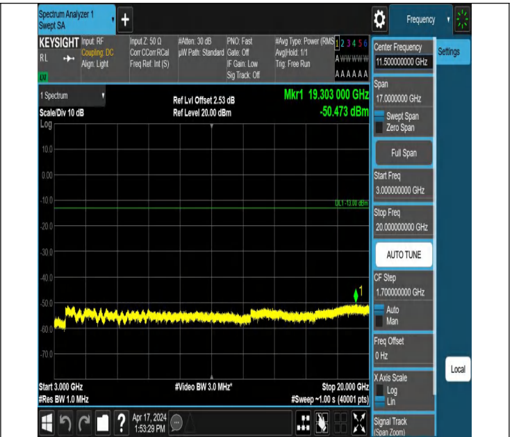
66-66-20MHz-5MHz-QPSK-QPSK-132072-132189-100RB#0-25R B#0-3000~20000MHz-PASS
