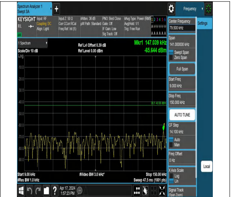
66-66-20MHz-5MHz-QPSK-QPSK-132522-132639-100RB#0-25R B#0-0.009~0.15MHz-PASS
