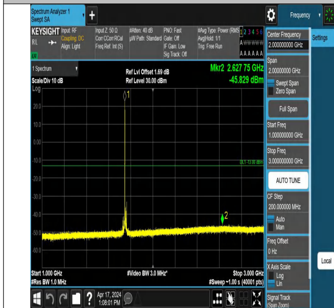
66-66-15MHz-20MHz-QPSK-QPSK-132401-132572-1RB#0-0RB#0-0-1000~3000MHz-PASS
