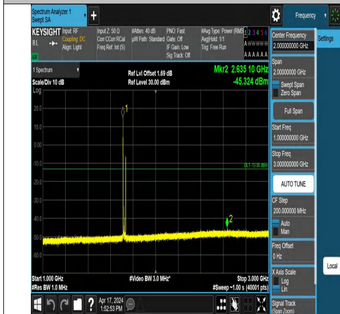
66-66-20MHz-5MHz-QPSK-QPSK-132072-132189-1RB#0-1RB#2 4-1000~3000MHz-PASS
