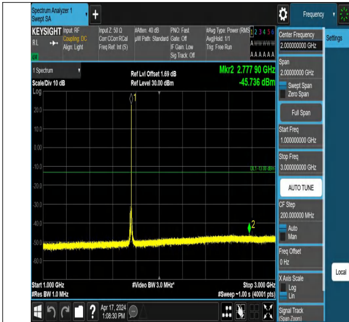
66-66-15MHz-20MHz-QPSK-QPSK-132401-132572-1RB#74-0RB #0-1000~3000MHz-PASS
