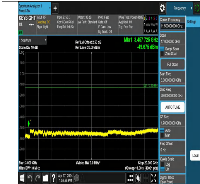
66-66-20MHz-5MHz-QPSK-QPSK-132072-132189-1RB#99-0RB# 0-3000~20000MHz-PASS
