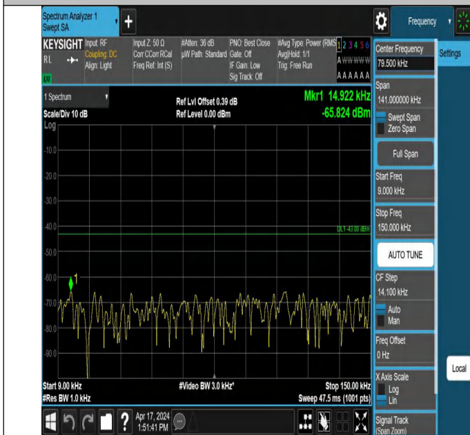
66-66-20MHz-5MHz-QPSK-QPSK-132072-132189-1RB#0-0RB#0 -0.009~0.15MHz-PASS
