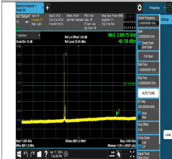
66-66-20MHz-5MHz-QPSK-QPSK-132397-132514-1RB#0-1RB#2 4-1000~3000MHz-PASS
