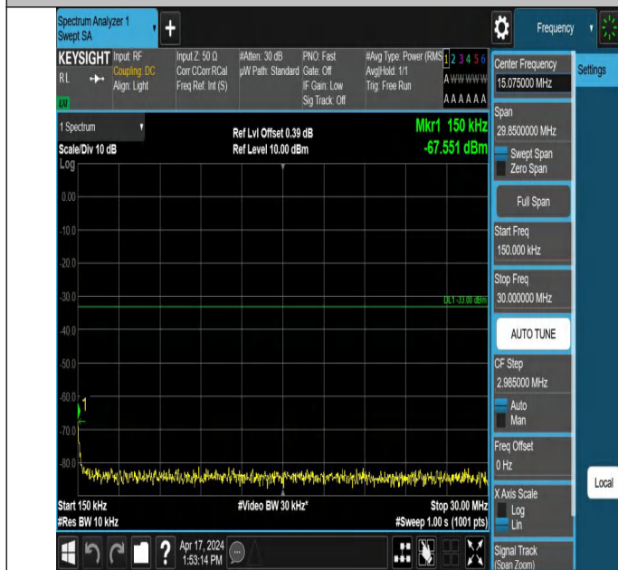
66-66-20MHz-5MHz-QPSK-QPSK-132072-132189-100RB#0-25R B#0-0.15~30MHz-PASS
