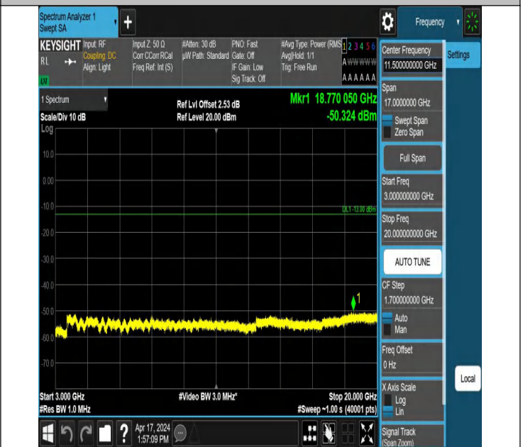
66-66-20MHz-5MHz-QPSK-QPSK-132522-132639-1RB#0-1RB# 24-3000~20000MHz-PASS
