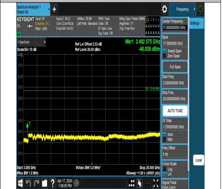
66-66-15MHz-20MHz-QPSK-QPSK-132401-132572-1RB#0-0RB#0-0-3000~20000MHz-PASS
