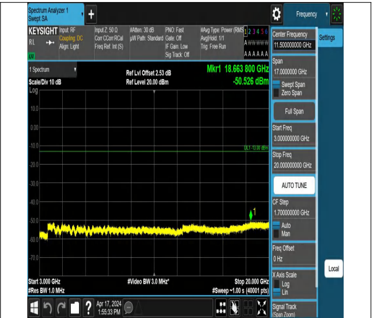
66-66-20MHz-5MHz-QPSK-QPSK-132397-132514-100RB#0-25R B#0-3000~20000MHz-PASS
