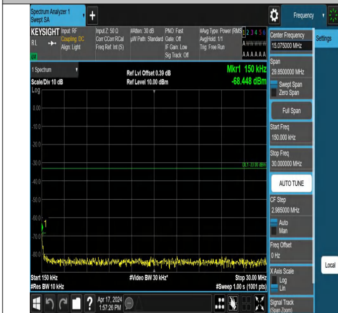
66-66-20MHz-5MHz-QPSK-QPSK-132522-132639-100RB#0-25R B#0-0.15~30MHz-PASS
