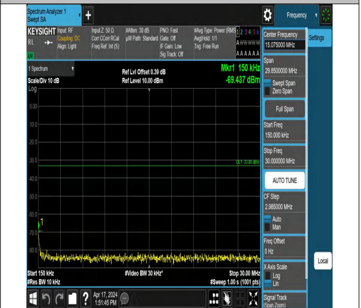
66-66-20MHz-5MHz-QPSK-QPSK-132072-132189-1RB#0-0RB# 0-0.15~30MHz-PASS
