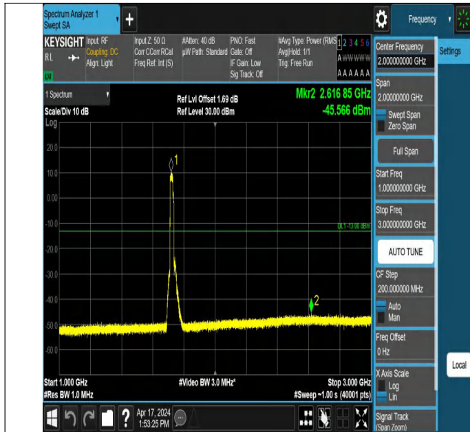
66-66-20MHz-5MHz-QPSK-QPSK-132072-132189-100RB#0-25R B#0-1000~3000MHz-PASS
