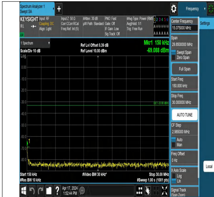
66-66-20MHz-5MHz-QPSK-QPSK-132072-132189-1RB#0-1RB#2 4-0.15~30MHz-PASS
