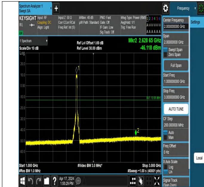
66-66-20MHz-5MHz-QPSK-QPSK-132397-132514-100RB#0-25R B#0-1000~3000MHz-PASS
