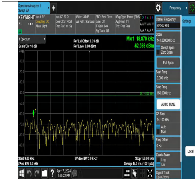
66-66-20MHz-5MHz-QPSK-QPSK-132522-132639-1RB#99-0RB# 0-0.009~0.15MHz-PASS
