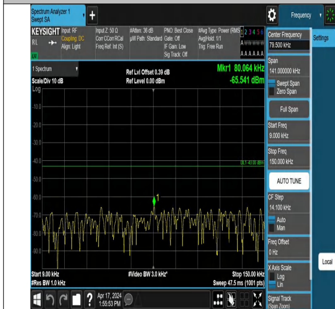
66-66-20MHz-5MHz-QPSK-QPSK-132522-132639-1RB#0-0RB#0 -0.009~0.15MHz-PASS
