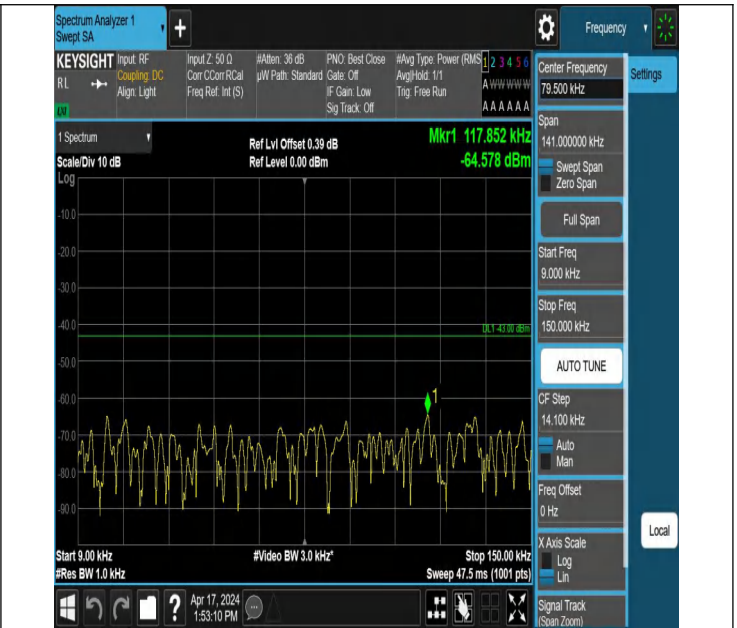
66-66-20MHz-5MHz-QPSK-QPSK-132072-132189-100RB#0-25R B#0-0.009~0.15MHz-PASS
