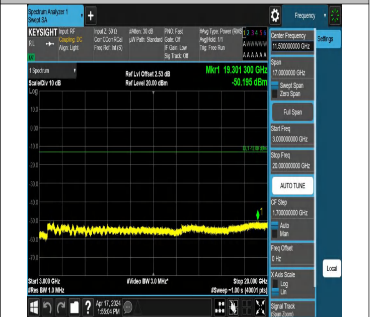
66-66-20MHz-5MHz-QPSK-QPSK-132397-132514-1RB#0-1RB# 24-3000~20000MHz-PASS
