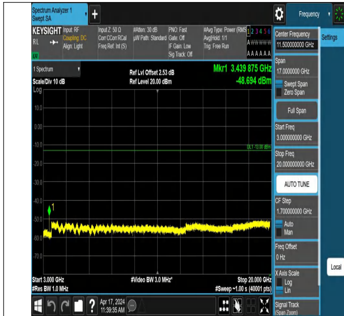
66-66-10MHz-20MHz-QPSK-QPSK-132027-132171-1RB#49-0RB #0-3000~20000MHz-PASS
