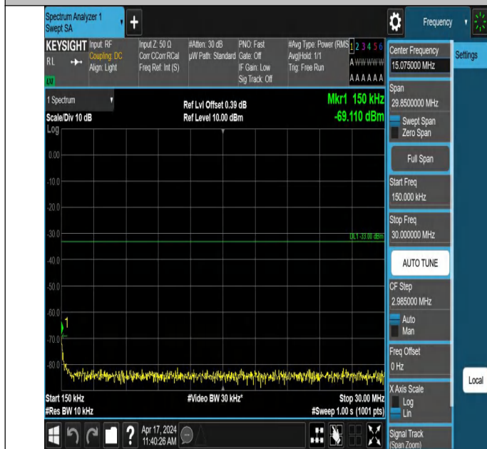
66-66-10MHz-20MHz-QPSK-QPSK-132328-132472-1RB#0-0RB# 0-0.15~30MHz-PASS
