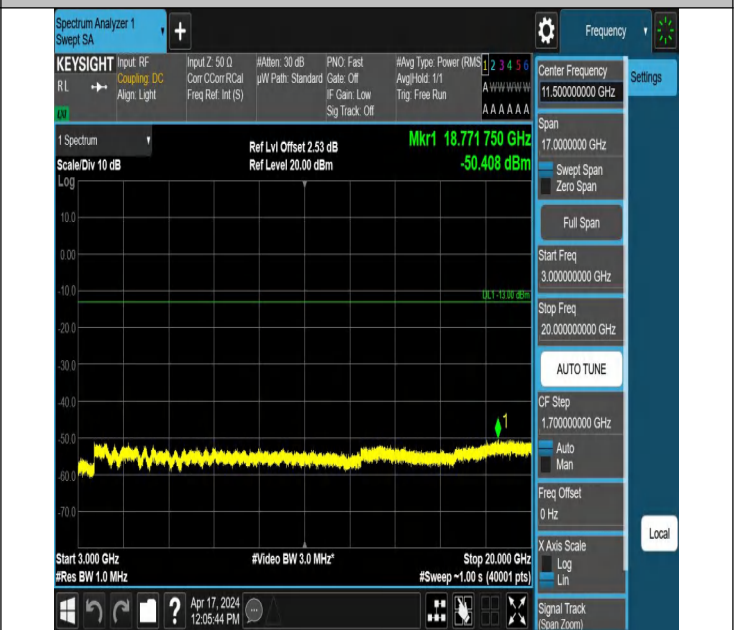
66-66-15MHz-10MHz-QPSK-QPSK-132373-132493-1RB#0-1RB #49-3000~20000MHz-PASS
