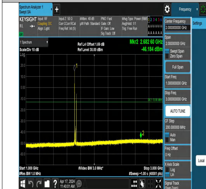
66-66-10MHz-20MHz-QPSK-QPSK-132027-132171-1RB#0-1RB# 99-1000~3000MHz-PASS
