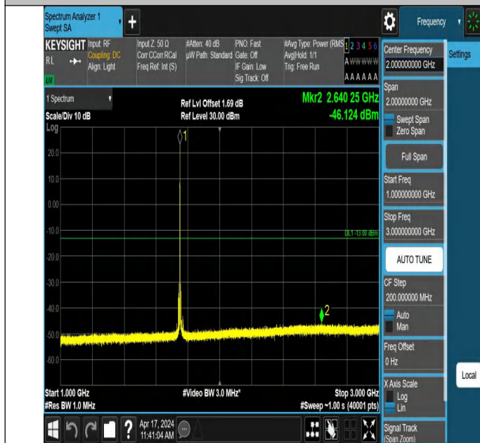
66-66-10MHz-20MHz-QPSK-QPSK-132328-132472-1RB#49-0RB #0-1000~3000MHz-PASS
