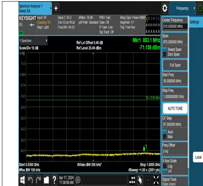
66-66-10MHz-20MHz-QPSK-QPSK-132027-132171-1RB#0-0RB# 0-30~1000MHz-PASS
