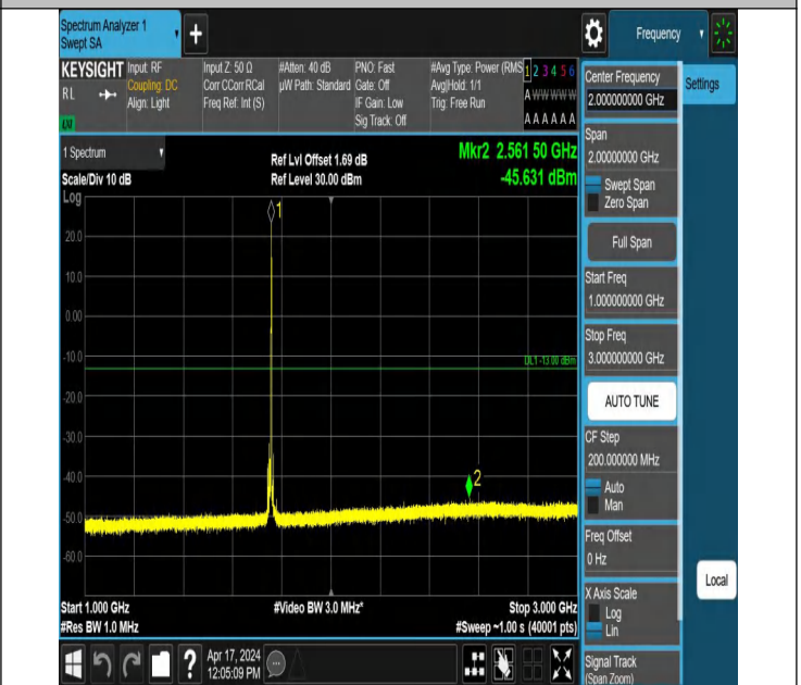
66-66-15MHz-10MHz-QPSK-QPSK-132373-132493-1RB#74-0R B#0-1000~3000MHz-PASS
