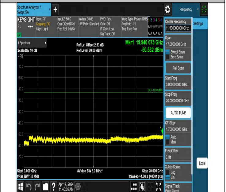
66-66-10MHz-20MHz-QPSK-QPSK-132027-132171-1RB#0-1RB# #99-3000~20000MHz-PASS
