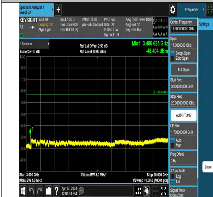
66-66-15MHz-10MHz-QPSK-QPSK-132373-132493-1RB#0-0RB# 0-3000~20000MHz-PASS
