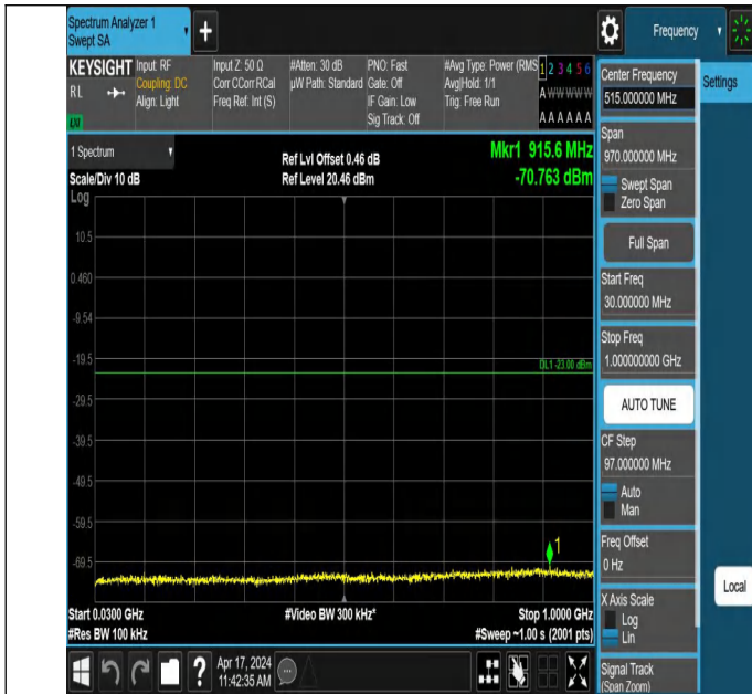
66-66-10MHz-20MHz-QPSK-QPSK-132428-132572-1RB#49-0RB #0-30~1000MHz-PASS
