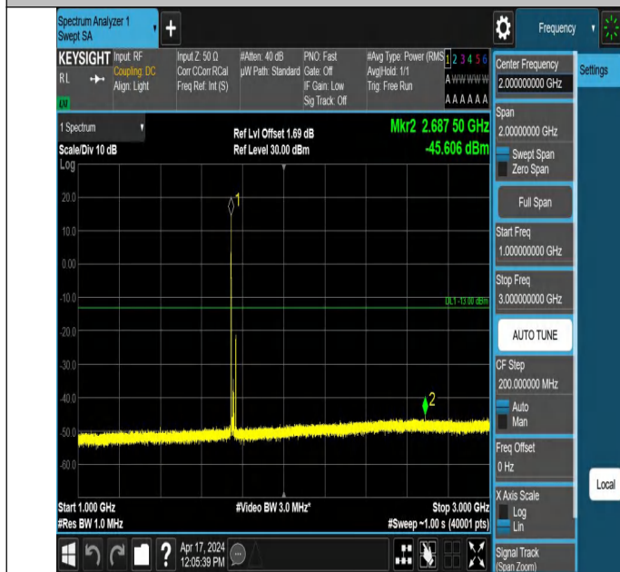
66-66-15MHz-10MHz-QPSK-QPSK-132373-132493-1RB#0-1RB# 49-1000~3000MHz-PASS
