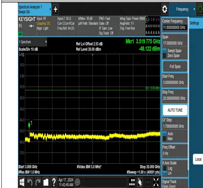
66-66-10MHz-20MHz-QPSK-QPSK-132428-132572-1RB#49-0RB #0-3000~20000MHz-PASS
