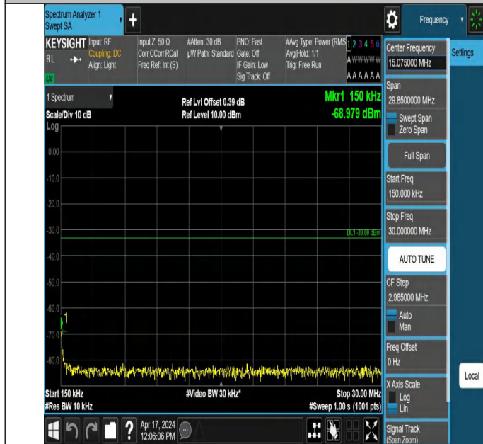
66-66-15MHz-10MHz-QPSK-QPSK-132499-132619-1RB#0-0RB# 0-0.15~30MHz-PASS
