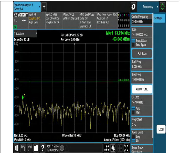
66-66-15MHz-10MHz-QPSK-QPSK-132499-132619-1RB#0-0RB #0-0.009~0.15MHz-PASS
