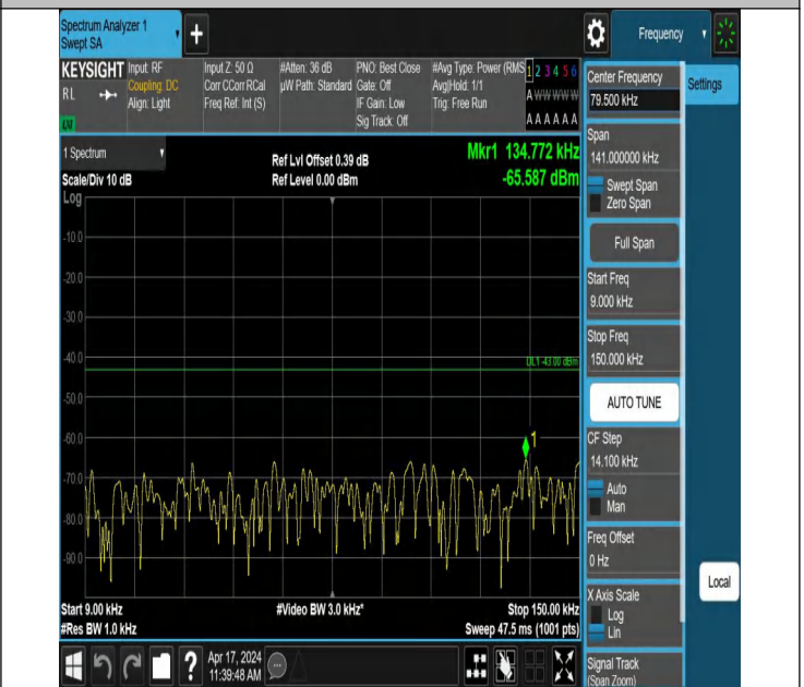
66-66-10MHz-20MHz-QPSK-QPSK-132027-132171-1RB#0-0-1RB #99-0.009~0.15MHz-PASS
