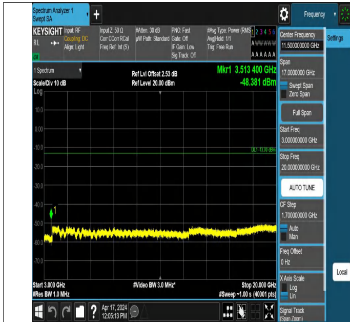
66-66-15MHz-10MHz-QPSK-QPSK-132373-132493-1RB#74-0RB #0-3000~20000MHz-PASS
