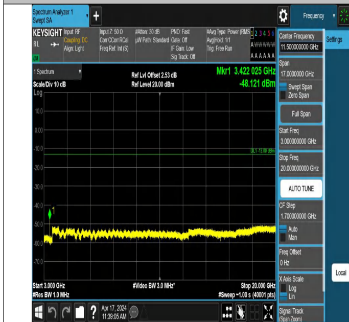
66-66-10MHz-20MHz-QPSK-QPSK-132027-132171-1RB#0-0RB# 0-3000~20000MHz-PASS
