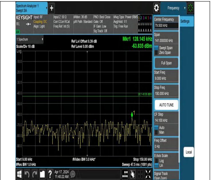
66-66-10MHz-20MHz-QPSK-QPSK-132328-132472-1RB#0-0RB #0-0.009~0.15MHz-PASS
