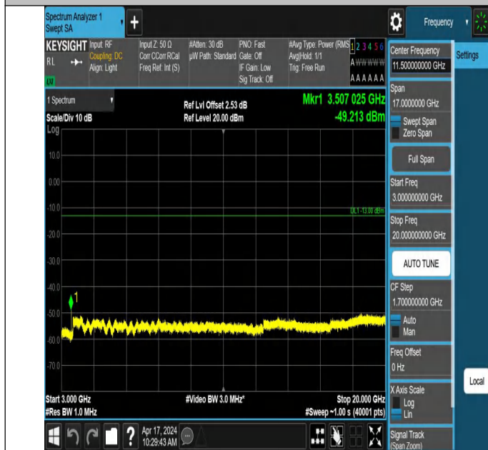
66-66-5MHz-20MHz-QPSK-QPSK-132428-132572-1RB#0-0RB#0 -3000~20000MHz-PASS
