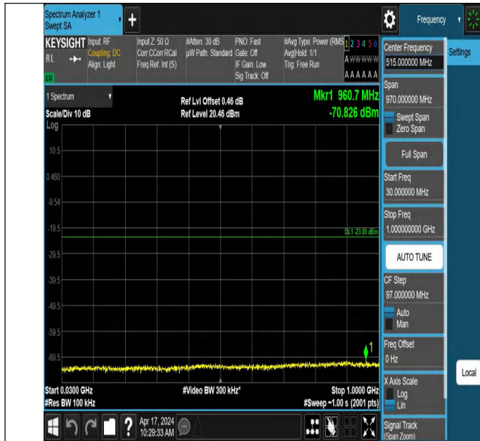
66-66-5MHz-20MHz-QPSK-QPSK-132428-132572-1RB#0-0RB#0 -30~1000MHz-PASS
