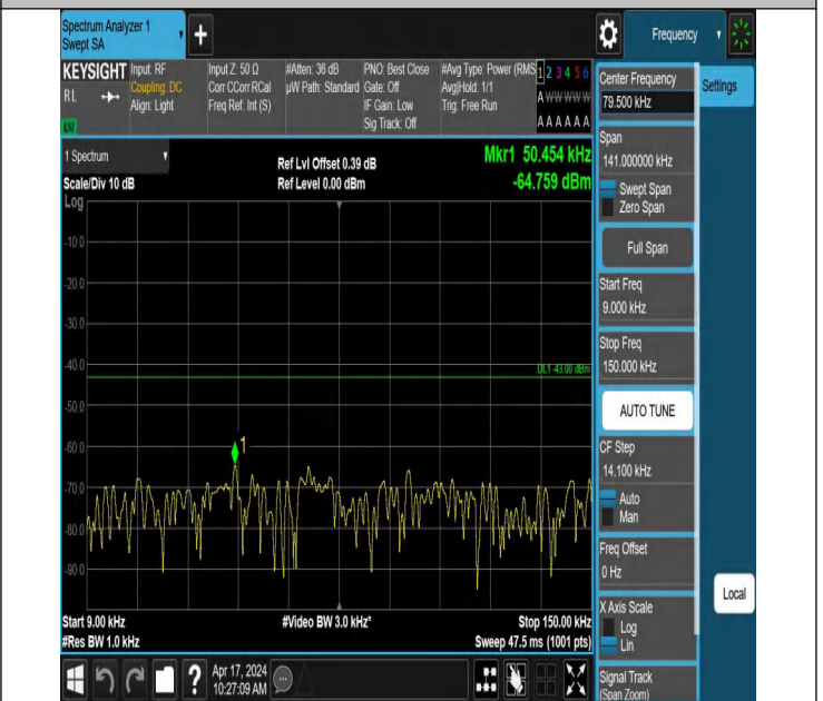
66-66-5MHz-20MHz-QPSK-QPSK-132328-132472-1RB#0-0RB# 0-0.009~0.15MHz-PASS
