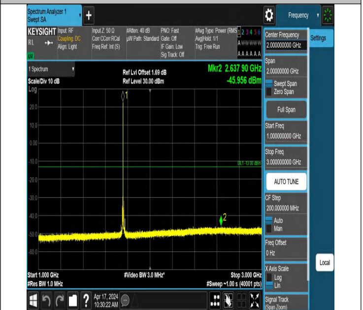
66-66-5MHz-20MHz-QPSK-QPSK-132428-132572-1RB#24-0RB #0-1000~3000MHz-PASS
