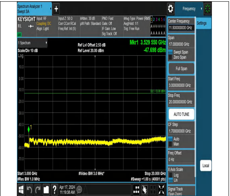
66-66-10MHz-15MHz-QPSK-QPSK-132477-132597-1RB#49-0RB B#0-3000~20000MHz-PASS
