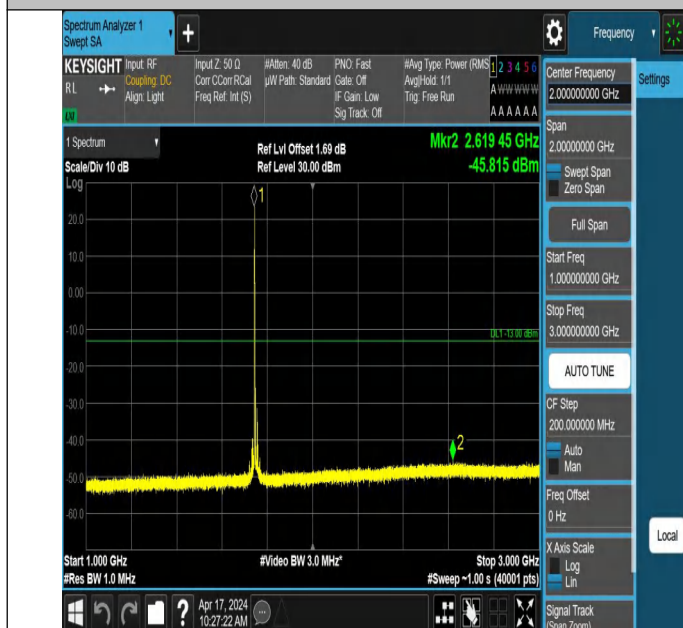
66-66-5MHz-20MHz-QPSK-QPSK-132328-132472-1RB#0-0RB#0 -1000~3000MHz-PASS
