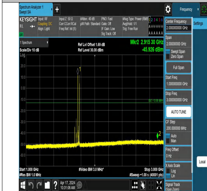
66-66-5MHz-20MHz-QPSK-QPSK-132428-132572-1RB#0-1RB#9 9-1000~3000MHz-PASS
