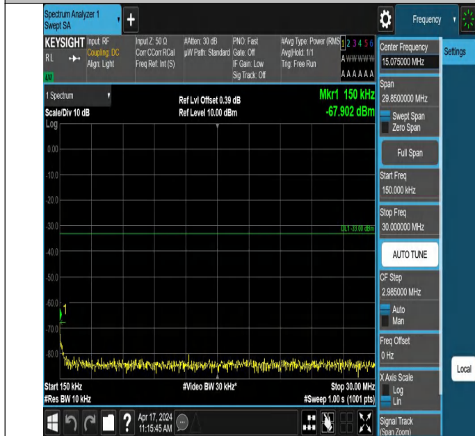
66-66-10MHz-15MHz-QPSK-QPSK-132025-132145-1RB#0-0RB# 0-0.15~30MHz-PASS
