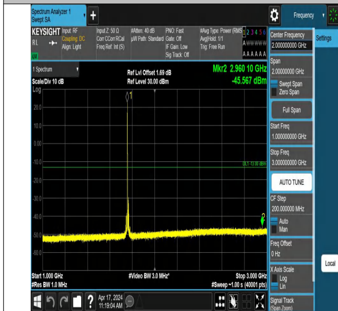
66-66-10MHz-15MHz-QPSK-QPSK-132477-132597-1RB#0-0RB# 0-1000~3000MHz-PASS
