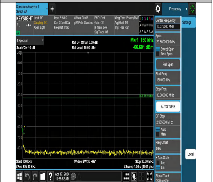
66-66-10MHz-20MHz-QPSK-QPSK-132027-132171-1RB#0-0RB# #0-0.15~30MHz-PASS
