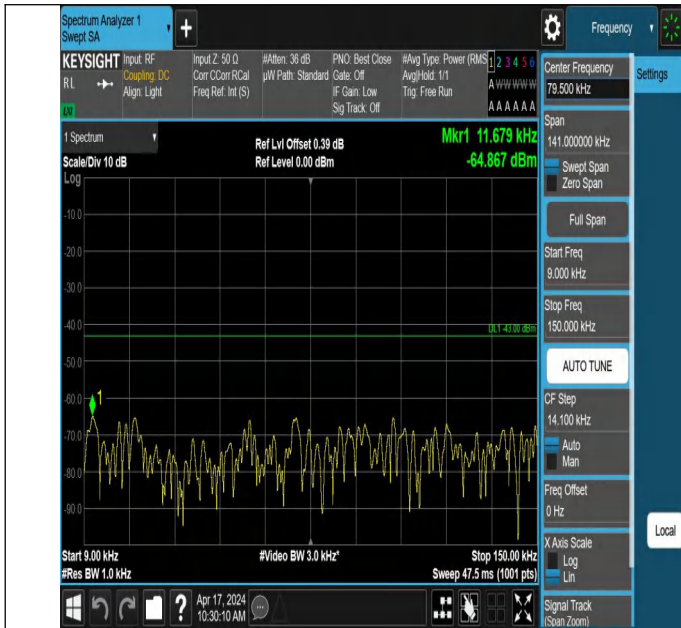
66-66-5MHz-20MHz-QPSK-QPSK-132428-132572-1RB#24-0RB# 0-0.009~0.15MHz-PASS
