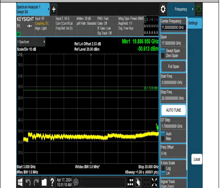
66-66-5MHz-20MHz-QPSK-QPSK-132428-132572-1RB#0-1RB# 99-3000~20000MHz-PASS
