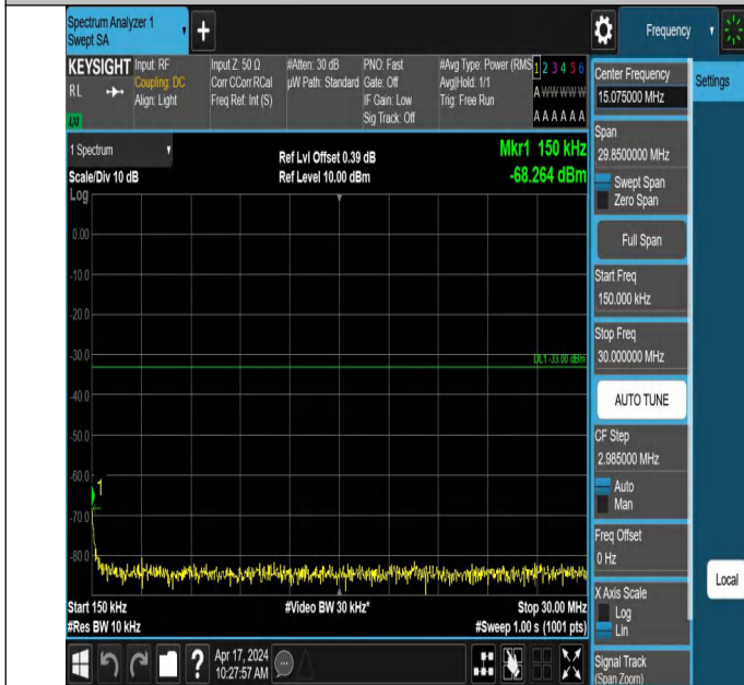
66-66-5MHz-20MHz-QPSK-QPSK-132328-132472-1RB#24-0RB# 0-0.15~30MHz-PASS
