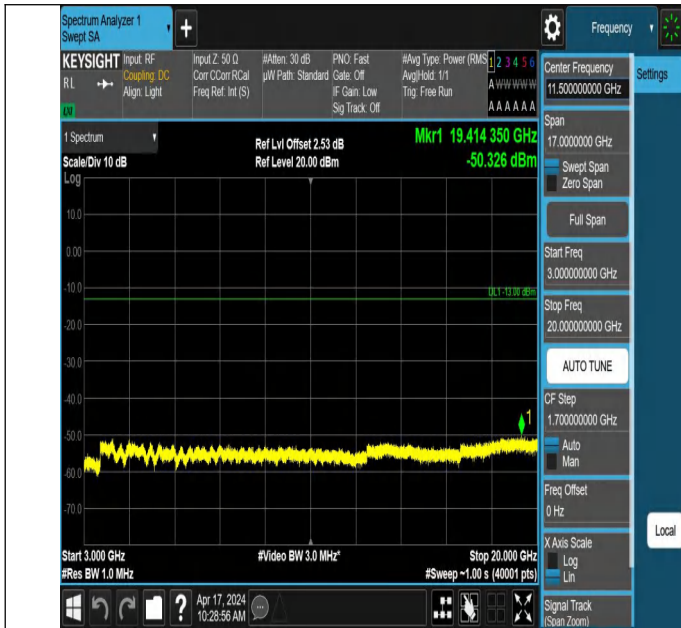
66-66-5MHz-20MHz-QPSK-QPSK-132328-132472-1RB#0-1RB#9 9-3000~20000MHz-PASS
