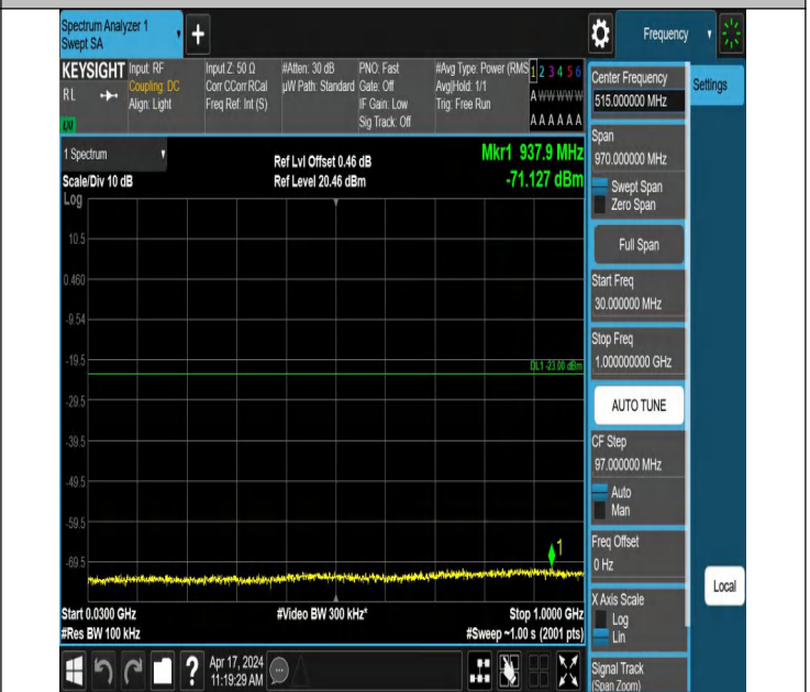
66-66-10MHz-15MHz-QPSK-QPSK-132477-132597-1RB#49-0RB#0-30~1000MHz-PASS
