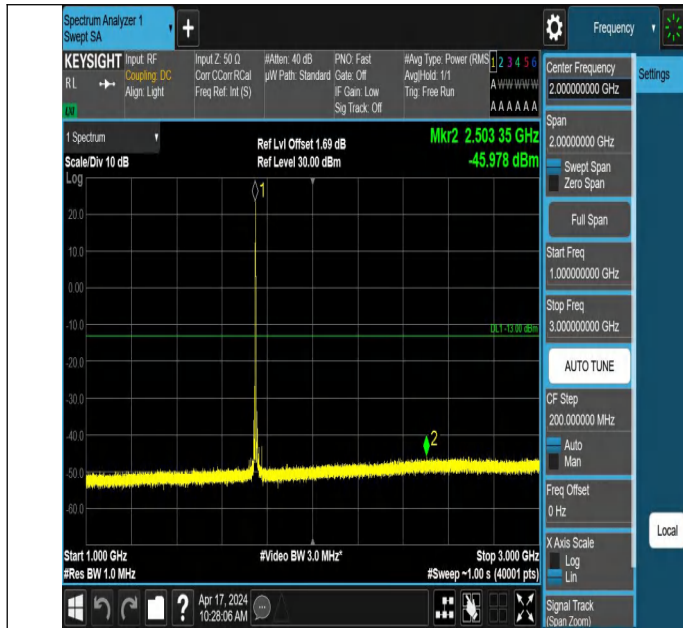
66-66-5MHz-20MHz-QPSK-QPSK-132328-132472-1RB#24-0RB# 0-1000~3000MHz-PASS
