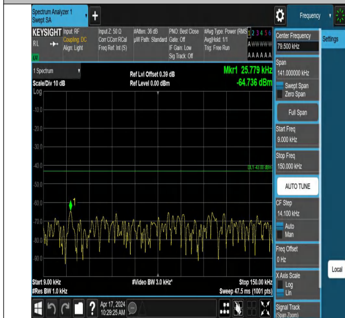
66-66-5MHz-20MHz-QPSK-QPSK-132428-132572-1RB#0-0RB#0 -0.009~0.15MHz-PASS
