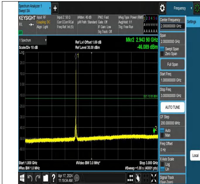
66-66-10MHz-15MHz-QPSK-QPSK-132477-132597-1RB#49-0RB #0-1000~3000MHz-PASS
