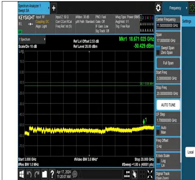
66-66-10MHz-15MHz-QPSK-QPSK-132477-132597-1RB#0-1RB#74-3000~20000MHz-PASS
