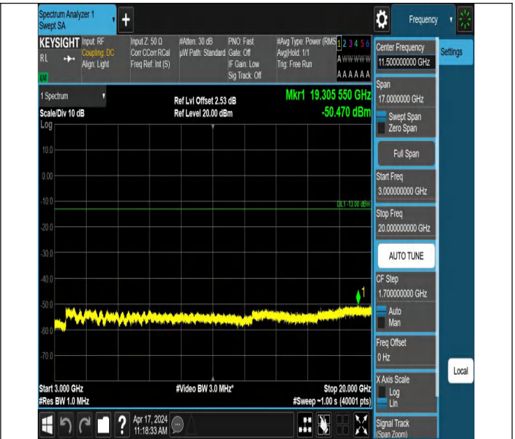
66-66-10MHz-15MHz-QPSK-QPSK-132351-132471-1RB#0-1RB #74-3000~20000MHz-PASS
