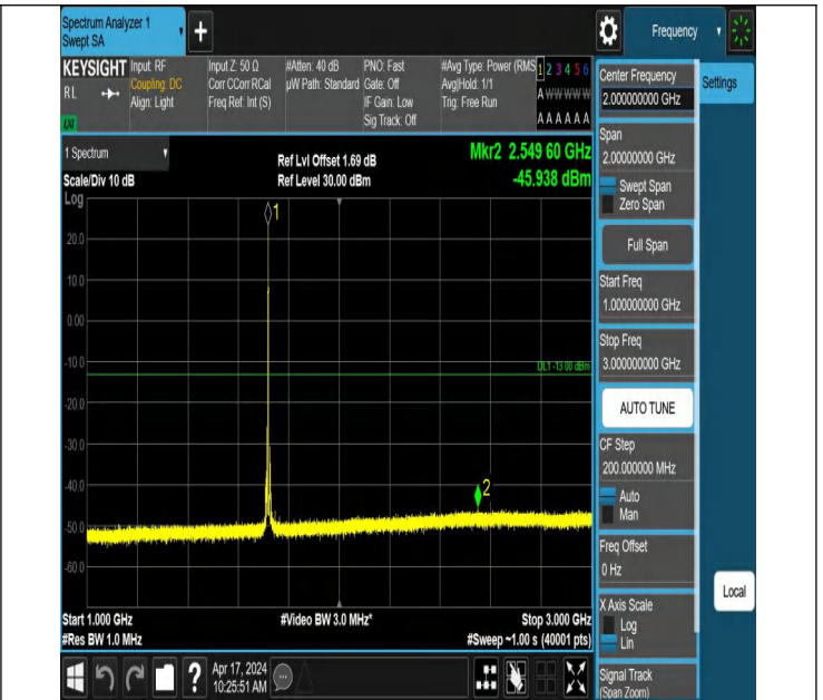
66-66-5MHz-20MHz-QPSK-QPSK-132027-132171-1RB#24-0RB# #0-1000~3000MHz-PASS
