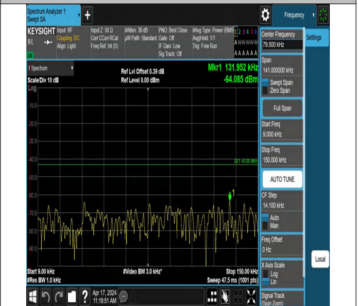
66-66-10MHz-15MHz-QPSK-QPSK-132477-132597-1RB#0-0RB #0-0.009~0.15MHz-PASS
