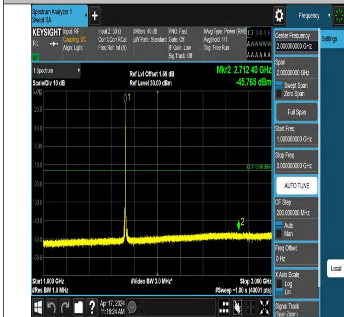
66-66-10MHz-15MHz-QPSK-QPSK-132025-132145-1RB#49-0RB #0-1000~3000MHz-PASS
