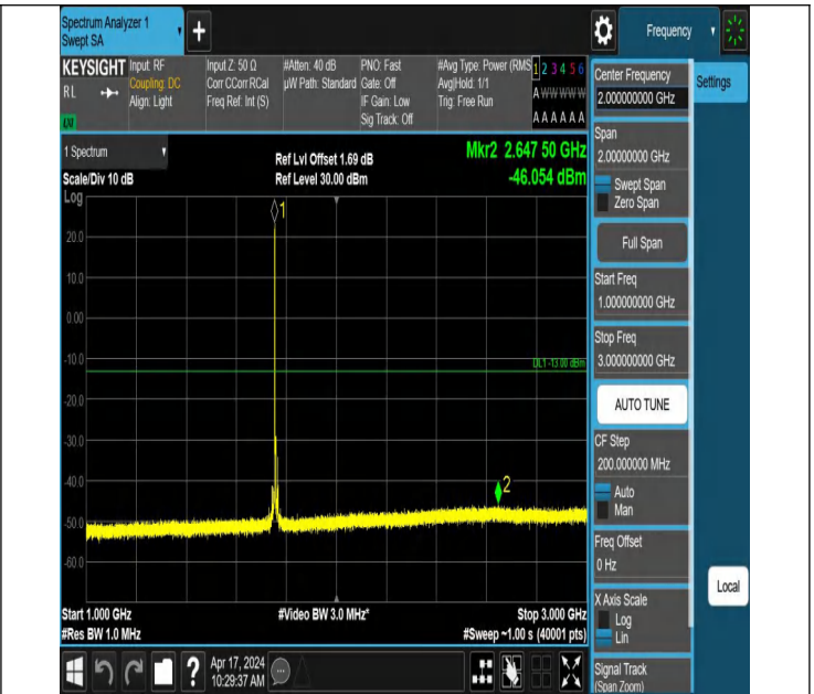
66-66-5MHz-20MHz-QPSK-QPSK-132428-132572-1RB#0-0RB#0 0-1000~3000MHz-PASS
