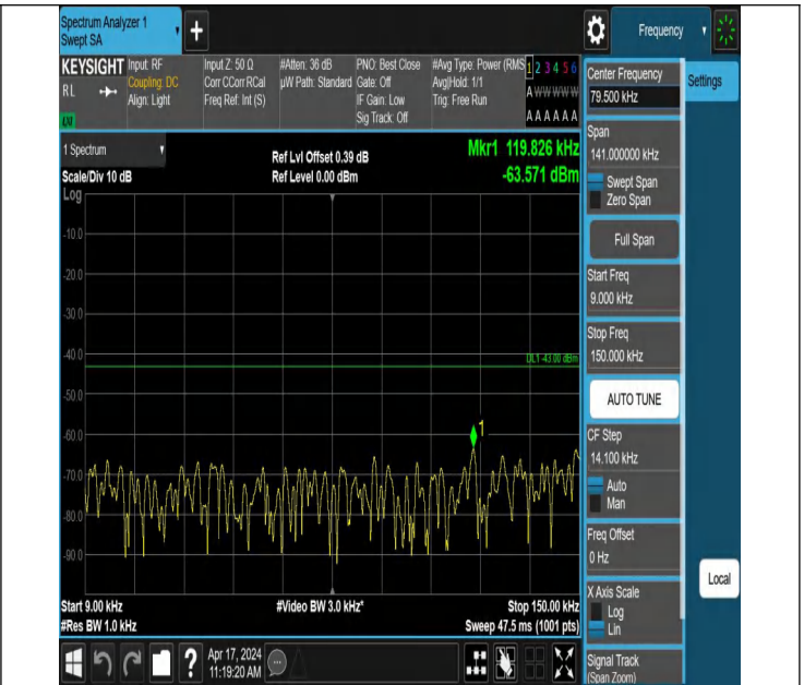
66-66-10MHz-15MHz-QPSK-QPSK-132477-132597-1RB#49-0RB#0-0.009~0.15MHz-PASS
