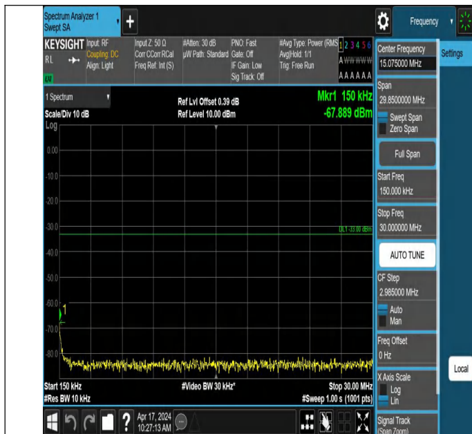
66-66-5MHz-20MHz-QPSK-QPSK-132328-132472-1RB#0-0RB#0 -0.15~30MHz-PASS
