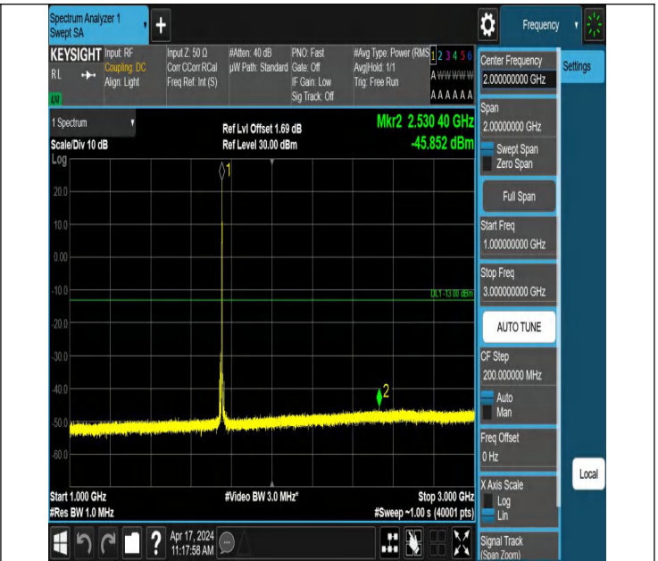
66-66-10MHz-15MHz-QPSK-QPSK-132351-132471-1RB#49-0R B#0-1000~3000MHz-PASS
