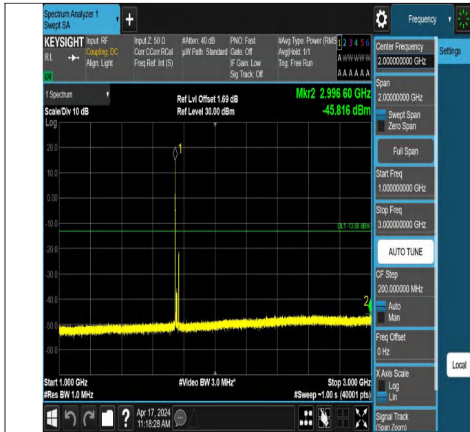
66-66-10MHz-15MHz-QPSK-QPSK-132351-132471-1RB#0-1RB# 74-1000~3000MHz-PASS
