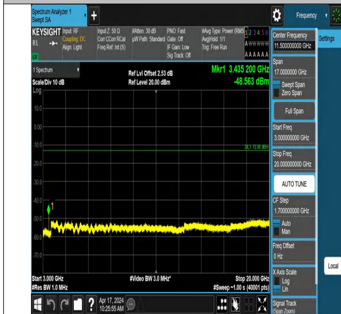
66-66-5MHz-20MHz-QPSK-QPSK-132027-132171-1RB#24-0RB# 0-3000~20000MHz-PASS
