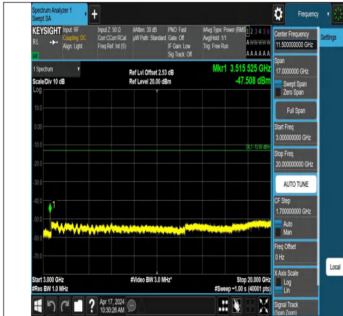
66-66-5MHz-20MHz-QPSK-QPSK-132428-132572-1RB#24-0RB# 0-3000~20000MHz-PASS
