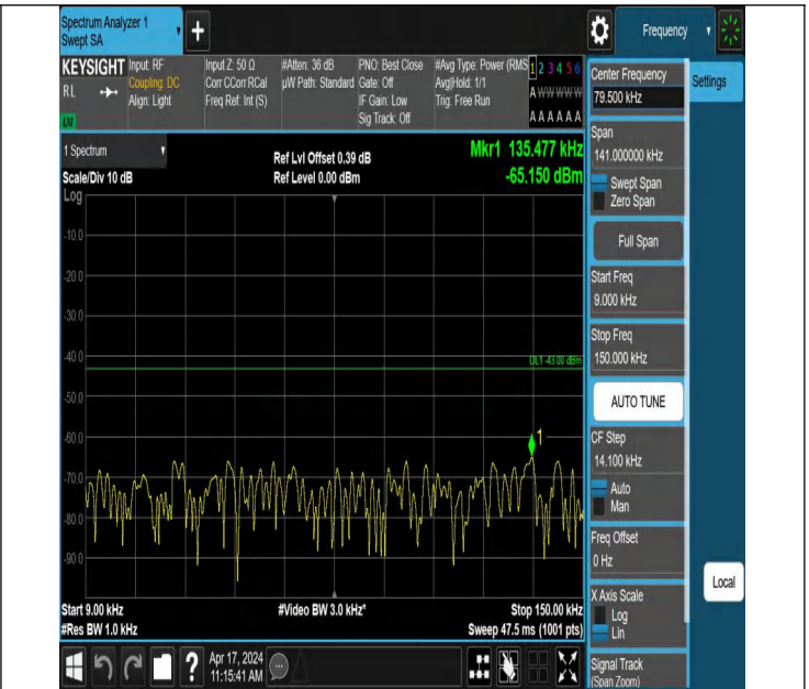
66-66-10MHz-15MHz-QPSK-QPSK-132025-132145-1RB#0-0RB #0-0.009~0.15MHz-PASS
