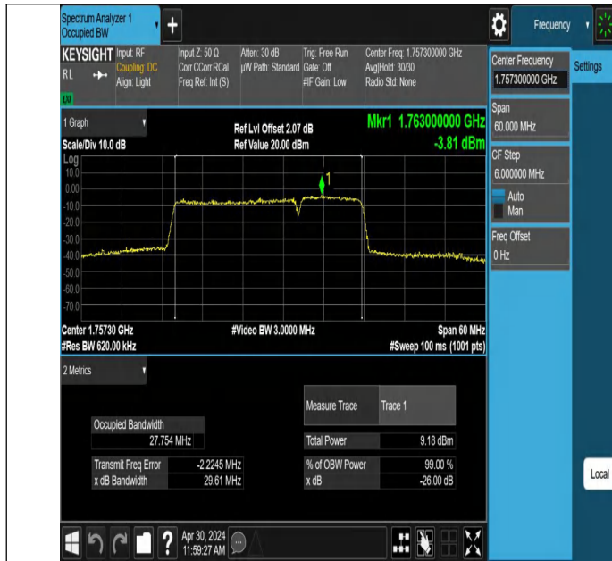
66-66-20MHz-10MHz-QPSK-QPSK-132373-132517-100RB#0-50 RB#0-PASS
