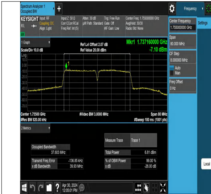
66-66-20MHz-20MHz-QPSK-QPSK-132323-132521-100RB#0-100RB#0-PASS
