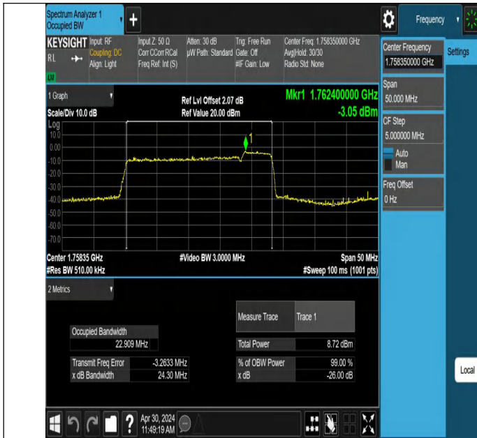
66-66-20MHz-5MHz-QPSK-QPSK-132397-132514-100RB#0-25R B#0-PASS
