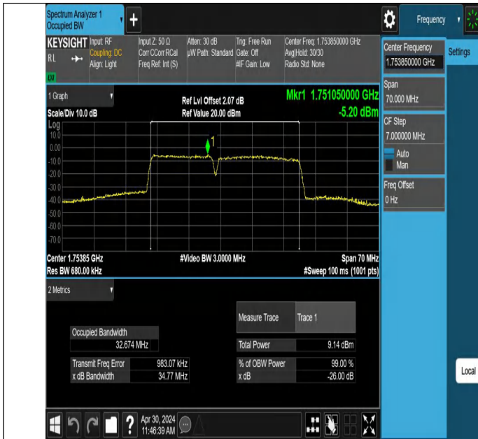
66-66-15MHz-20MHz-QPSK-QPSK-132325-132496-75RB#0-100 RB#0-PASS
