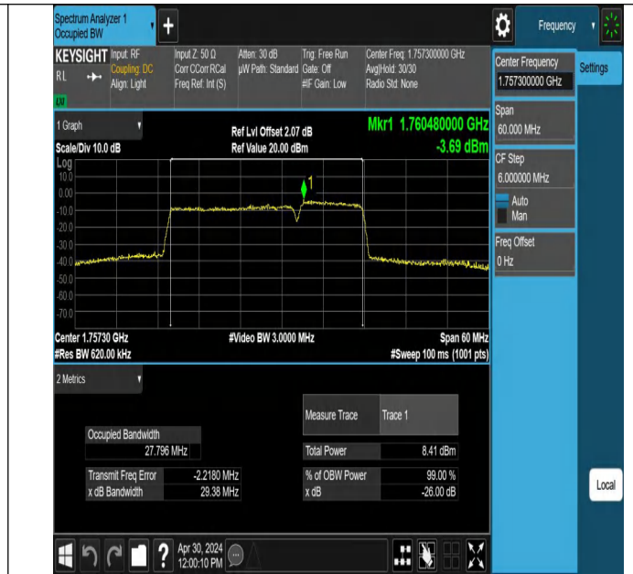
66-66-20MHz-10MHz-64QAM-64QAM-132373-132517-100RB#0 -50RB#0-PASS
