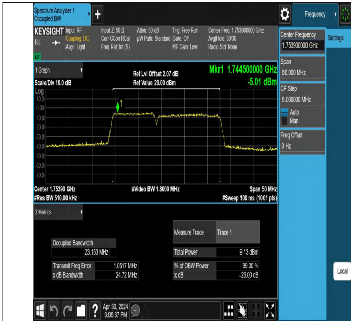
66-66-10MHz-15MHz-QPSK-QPSK-132351-132471-50RB#0-75R B#0-PASS
