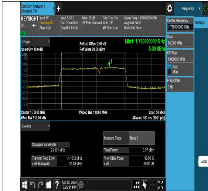
66-66-15MHz-10MHz-QPSK-QPSK-132373-132493-75RB#0-50RB#0-PASS
