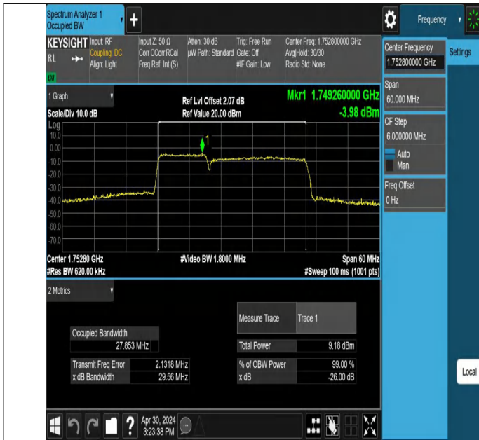
66-66-10MHz-20MHz-QPSK-QPSK-132328-132472-50RB#0-100 RB#0-PASS
