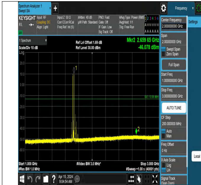
66-66-10MHz-10MHz-QPSK-QPSK-132022-132121-1RB#0-1RB #49-1000~3000MHz-PASS
