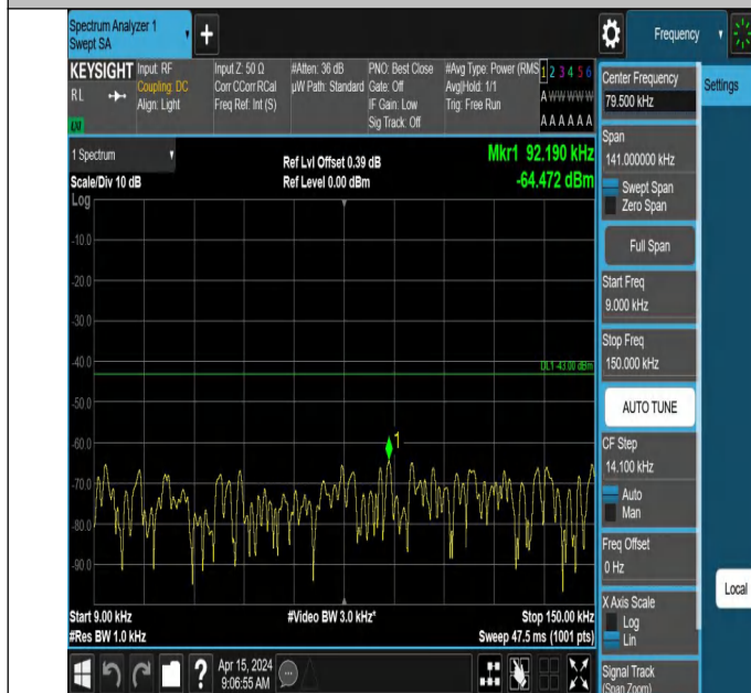
66-66-10MHz-10MHz-QPSK-QPSK-132523-132622-1RB#0-0RB #0-0.009~0.15MHz-PASS
