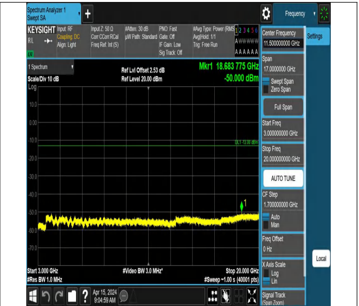
66-66-10MHz-10MHz-QPSK-QPSK-132022-132121-1RB#0-1RB #49-3000~20000MHz-PASS
