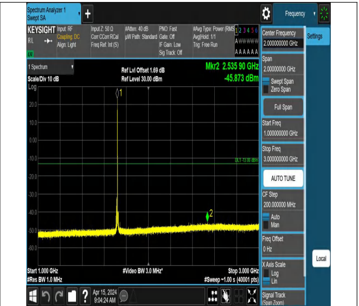
66-66-10MHz-10MHz-QPSK-QPSK-132022-132121-1RB#49-0R B#0-1000~3000MHz-PASS
