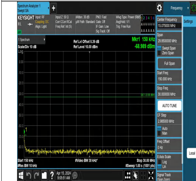
66-66-10MHz-10MHz-QPSK-QPSK-132373-132472-1RB#49-0R B#0-0.15~30MHz-PASS
