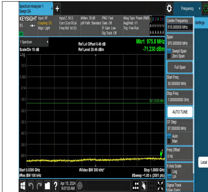
66-66-10MHz-10MHz-QPSK-QPSK-132523-132622-1RB#0-0RB #0-30~1000MHz-PASS
