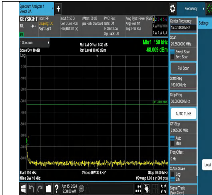
66-66-10MHz-10MHz-QPSK-QPSK-132523-132622-1RB#0-1RB #49-0.15~30MHz-PASS
