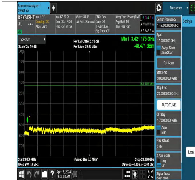
66-66-10MHz-10MHz-QPSK-QPSK-132022-132121-1RB#0-0RB #0-3000~20000MHz-PASS
