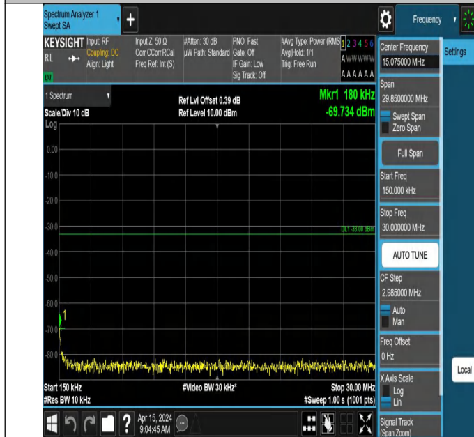
66-66-10MHz-10MHz-QPSK-QPSK-132022-132121-1RB#0-0RB #49-0.15~30MHz-PASS
