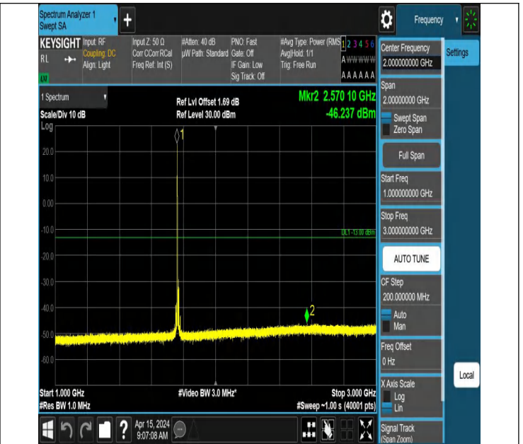
66-66-10MHz-10MHz-QPSK-QPSK-132523-132622-1RB#0-0RB #0-1000~3000MHz-PASS
