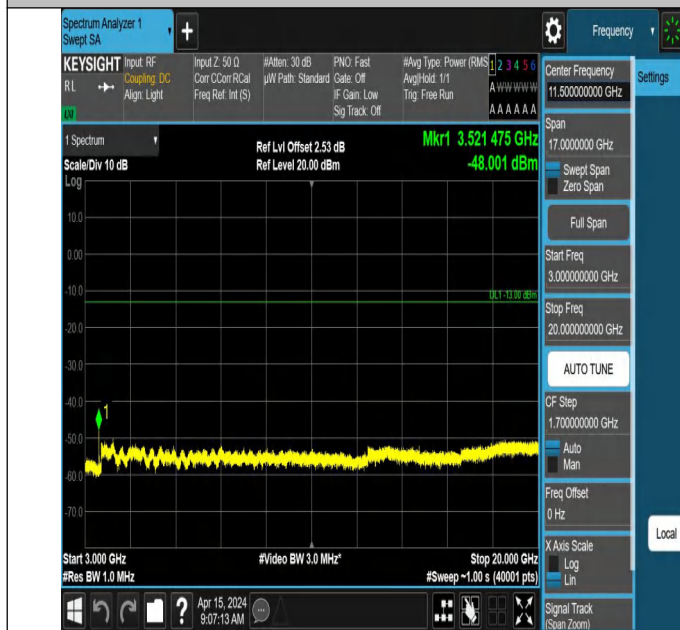
66-66-10MHz-10MHz-QPSK-QPSK-132523-132622-1RB#0-0RB #0-3000~20000MHz-PASS
