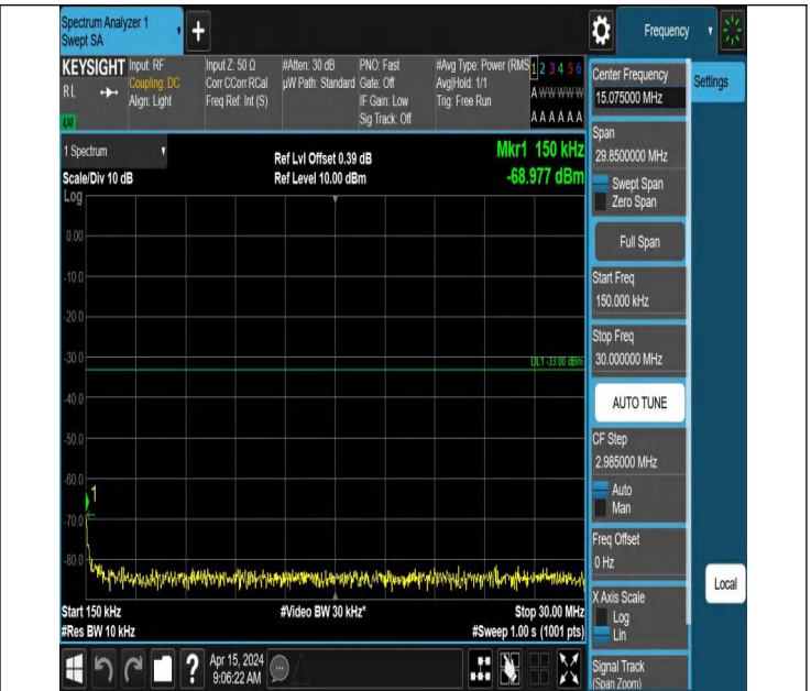
66-66-10MHz-10MHz-QPSK-QPSK-132373-132472-1RB#0-1RB #49-0.15~30MHz-PASS
