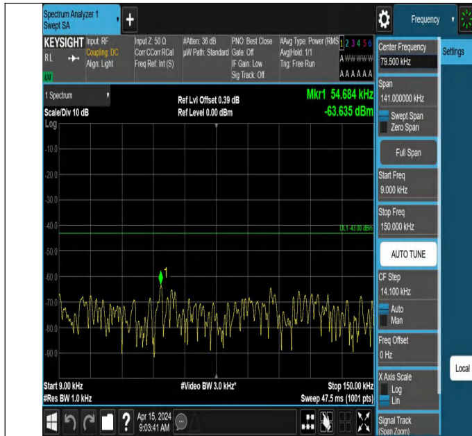
66-66-10MHz-10MHz-QPSK-QPSK-132022-132121-1RB#0-0RB #0-0.009~0.15MHz-PASS
