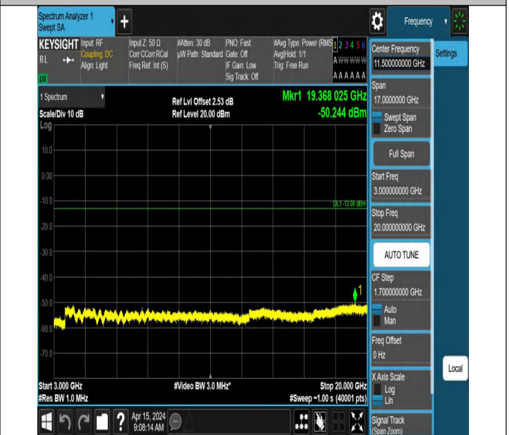
66-66-10MHz-10MHz-QPSK-QPSK-132523-132622-1RB#0-1RB #49-3000~20000MHz-PASS
