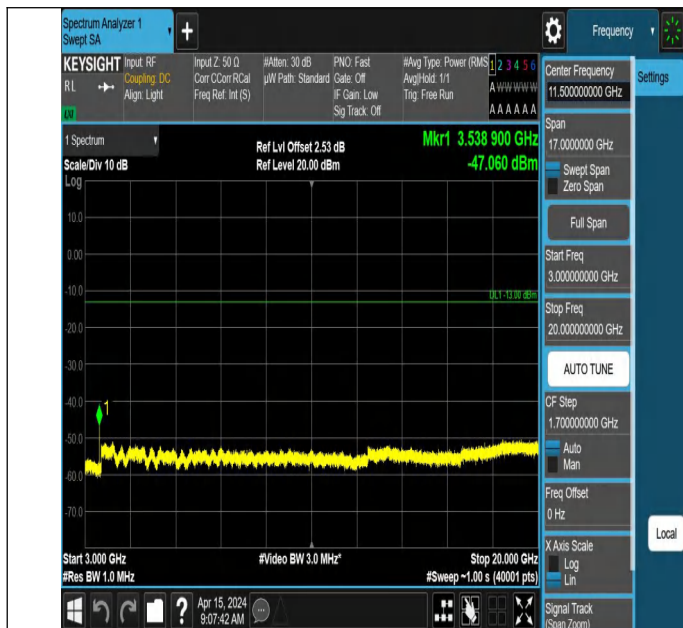
66-66-10MHz-10MHz-QPSK-QPSK-132523-132622-1RB#49-0R B#0-3000~20000MHz-PASS
