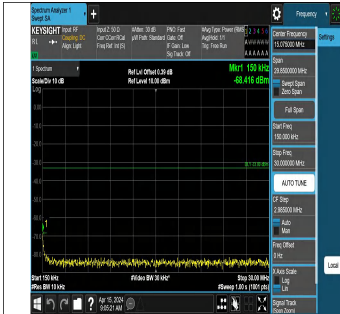
66-66-10MHz-10MHz-QPSK-QPSK-132373-132472-1RB#0-0RB #0-0.15~30MHz-PASS
