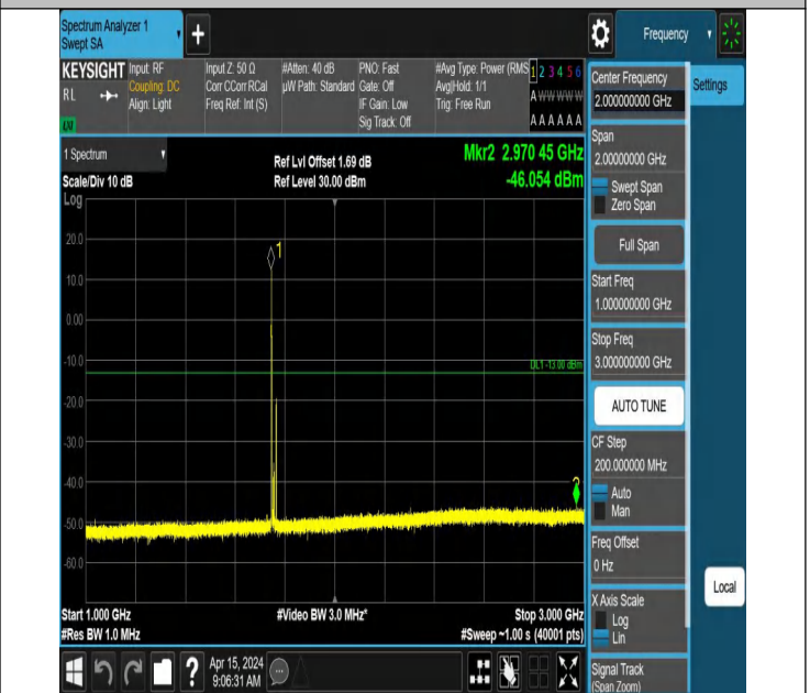
66-66-10MHz-10MHz-QPSK-QPSK-132373-132472-1RB#0-1RB #49-1000~3000MHz-PASS
