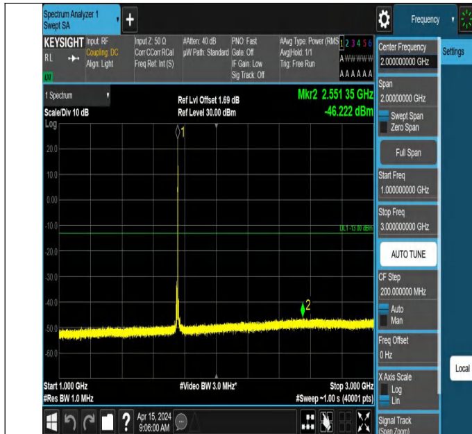
66-66-10MHz-10MHz-QPSK-QPSK-132373-132472-1RB#49-0R B#0-1000~3000MHz-PASS
