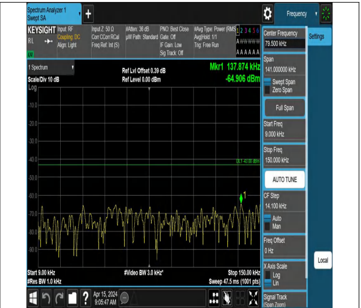
66-66-10MHz-10MHz-QPSK-QPSK-132373-132472-1RB#49-0R B#0-0.009~0.15MHz-PASS
