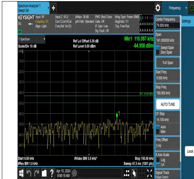
66-66-10MHz-10MHz-QPSK-QPSK-132373-132472-1RB#0-1RB #49-0.009~0.15MHz-PASS
