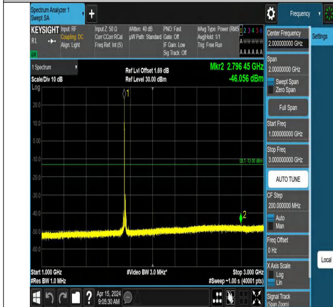
66-66-10MHz-10MHz-QPSK-QPSK-132373-132472-1RB#0-0RB #0-1000~3000MHz-PASS
