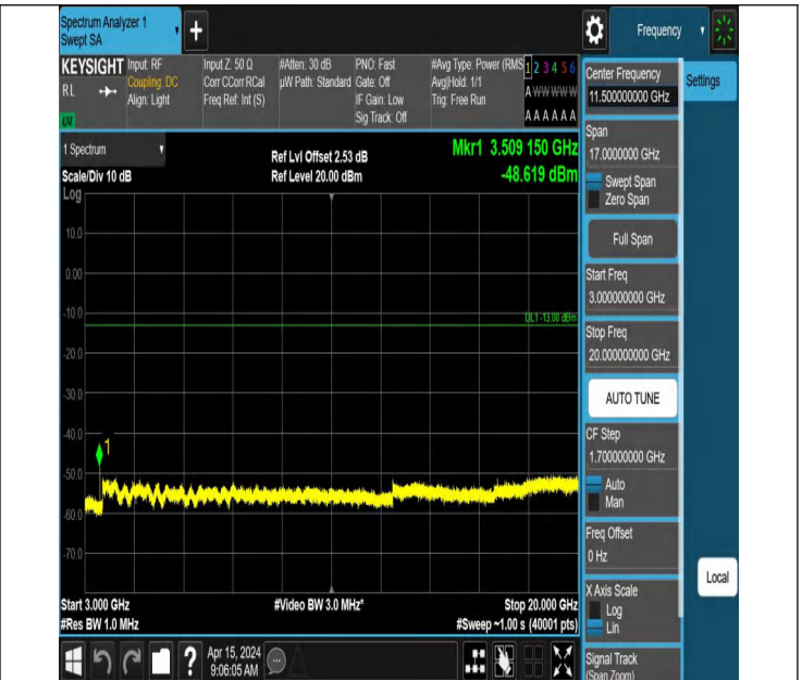
66-66-10MHz-10MHz-QPSK-QPSK-132373-132472-1RB#49-0R B#0-3000~20000MHz-PASS
