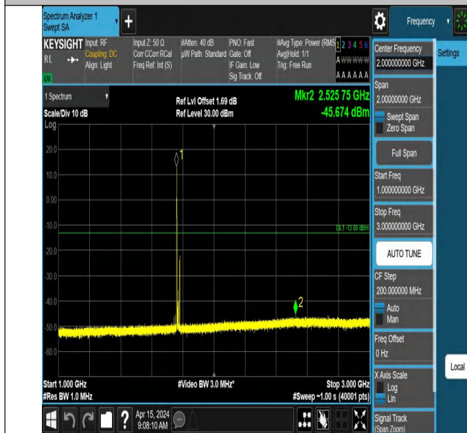
66-66-10MHz-10MHz-QPSK-QPSK-132523-132622-1RB#0-1RB #49-1000~3000MHz-PASS
