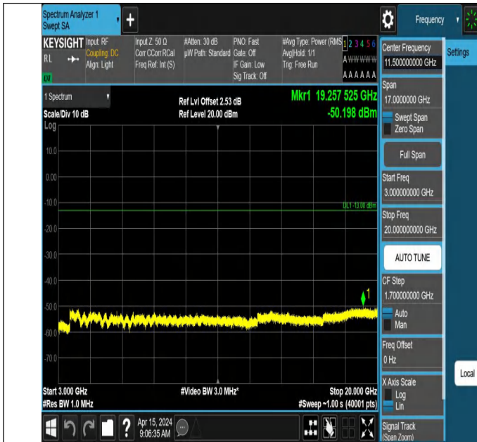
66-66-10MHz-10MHz-QPSK-QPSK-132373-132472-1RB#0-1RB #49-3000~20000MHz-PASS
