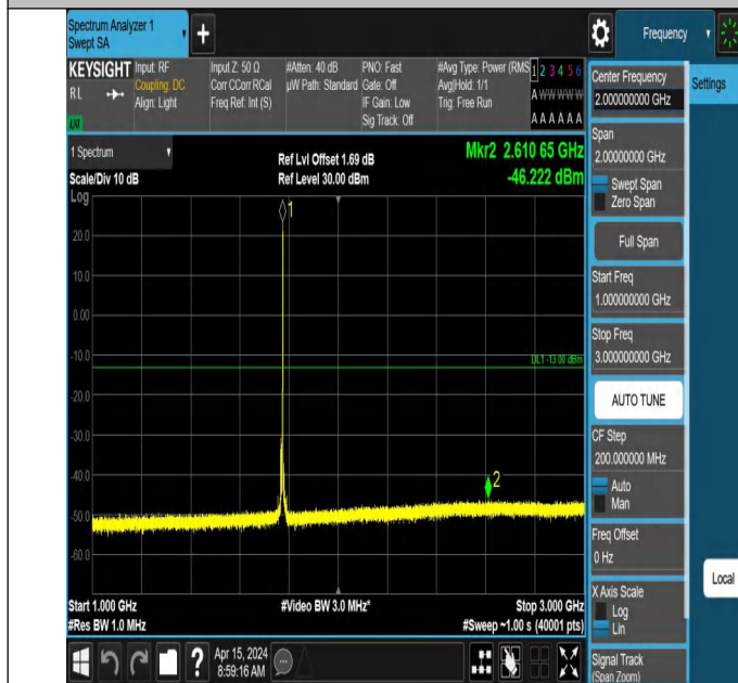
66-66-10MHz-5MHz-QPSK-QPSK-132572-132644-1RB#49-0RB #0-1000~3000MHz-PASS
