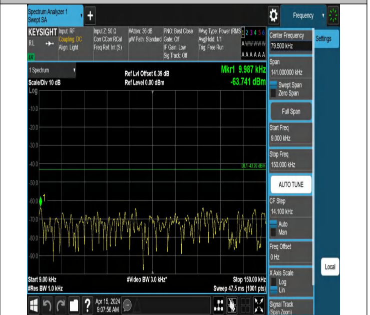
66-66-10MHz-10MHz-QPSK-QPSK-132523-132622-1RB#0-1RB #49-0.009~0.15MHz-PASS
