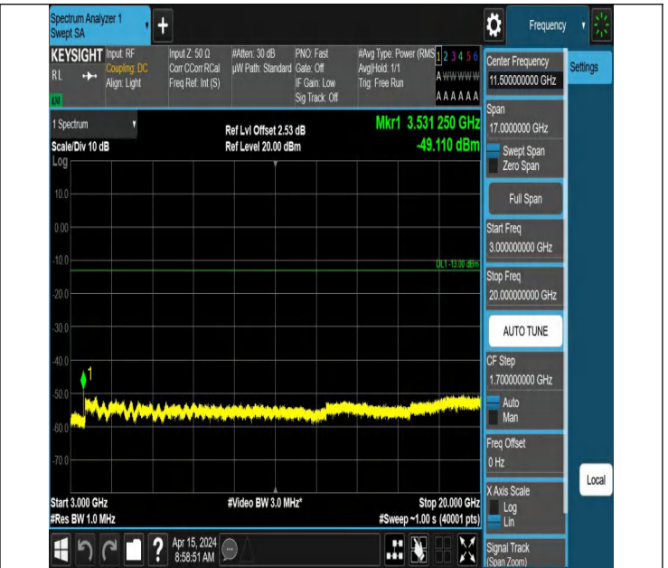
66-66-10MHz-5MHz-QPSK-QPSK-132572-132644-1RB#0-0RB# 0-3000~20000MHz-PASS
