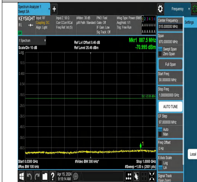
66-66-5MHz-15MHz-QPSK-QPSK-132504-132597-1RB#0-0RB# 0-30~1000MHz-PASS
