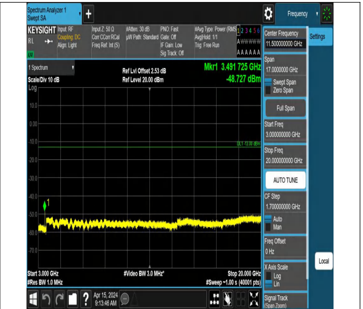
66-66-5MHz-15MHz-QPSK-QPSK-132353-132446-1RB#0-0RB# 0-3000~20000MHz-PASS
