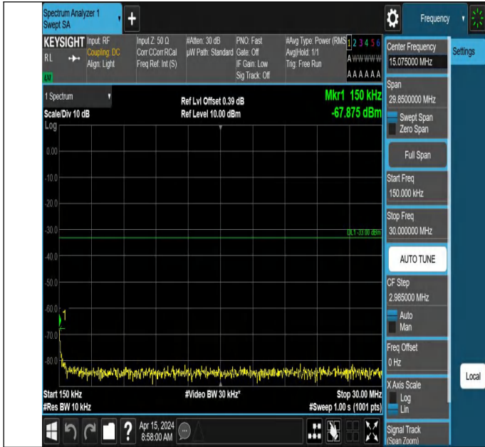
66-66-10MHz-5MHz-QPSK-QPSK-132397-132469-1RB#0-1RB# 24-0.15~30MHz-PASS
