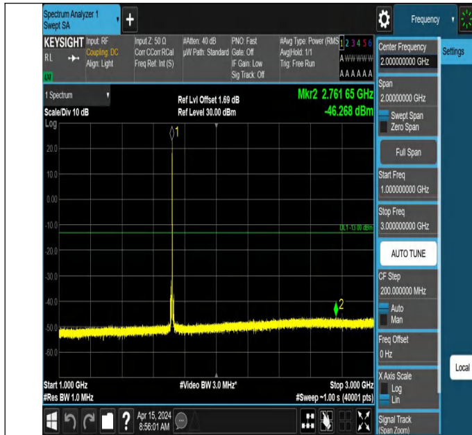
66-66-10MHz-5MHz-QPSK-QPSK-132022-132094-1RB#49-0RB #0-1000~3000MHz-PASS
