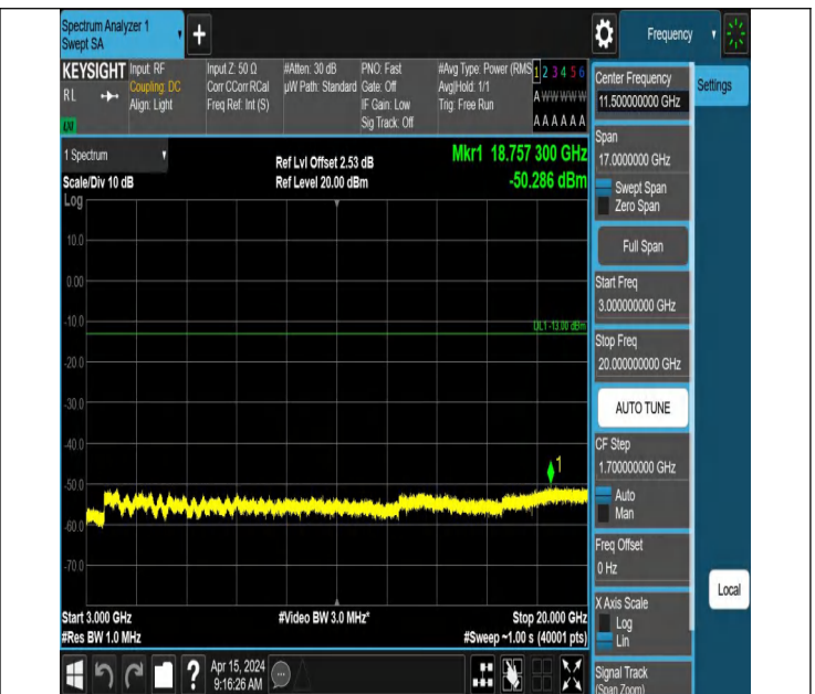
66-66-5MHz-15MHz-QPSK-QPSK-132504-132597-1RB#0-1RB# 74-3000~20000MHz-PASS
