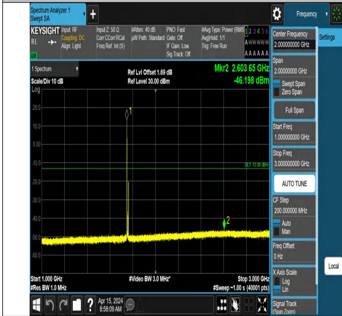
66-66-10MHz-5MHz-QPSK-QPSK-132397-132469-1RB#0-1RB# 24-1000~3000MHz-PASS
