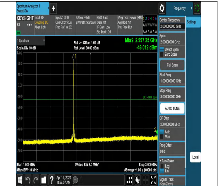
66-66-10MHz-5MHz-QPSK-QPSK-132397-132469-1RB#0-0RB# 0-1000~3000MHz-PASS
