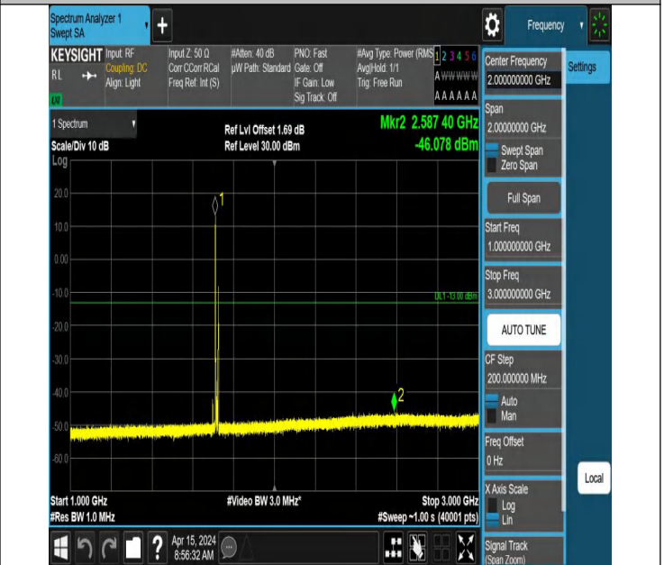
66-66-10MHz-5MHz-QPSK-QPSK-132022-132094-1RB#0-1RB# 24-1000~3000MHz-PASS
