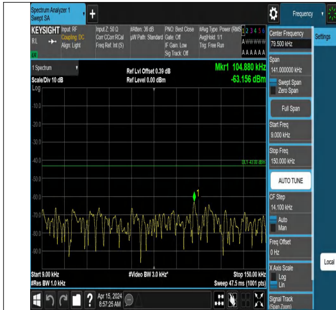
66-66-10MHz-5MHz-QPSK-QPSK-132397-132469-1RB#49-0RB #0-0.009~0.15MHz-PASS
