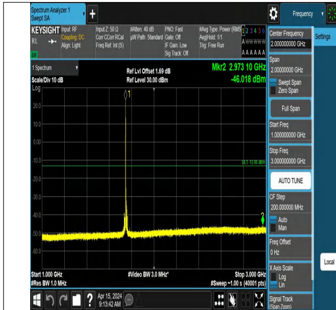
66-66-5MHz-15MHz-QPSK-QPSK-132353-132446-1RB#0-0RB# 0-1000~3000MHz-PASS
