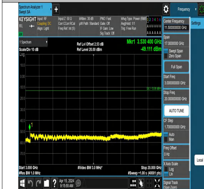
66-66-5MHz-15MHz-QPSK-QPSK-132504-132597-1RB#24-0RB #0-3000~20000MHz-PASS
