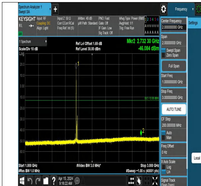
66-66-5MHz-15MHz-QPSK-QPSK-132504-132597-1RB#0-1RB# 74-1000~3000MHz-PASS
