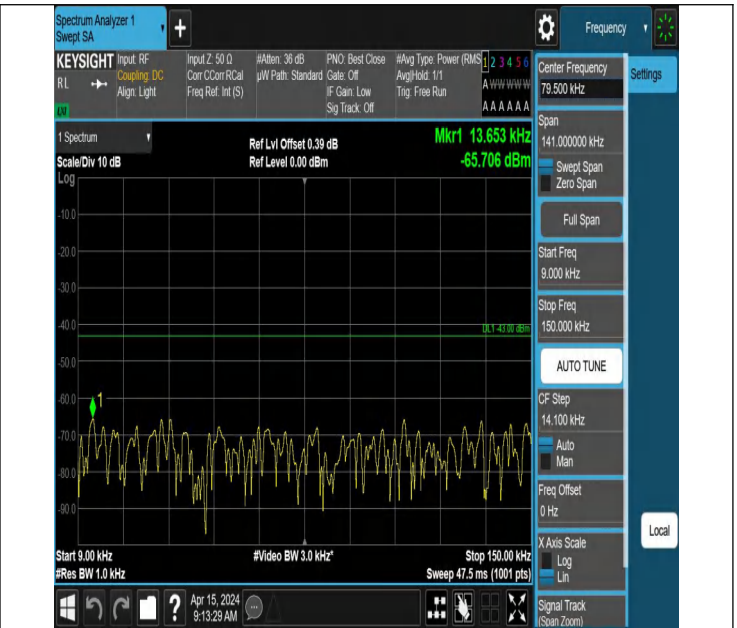
66-66-5MHz-15MHz-QPSK-QPSK-132353-132446-1RB#0-0RB# 0-0.009~0.15MHz-PASS
