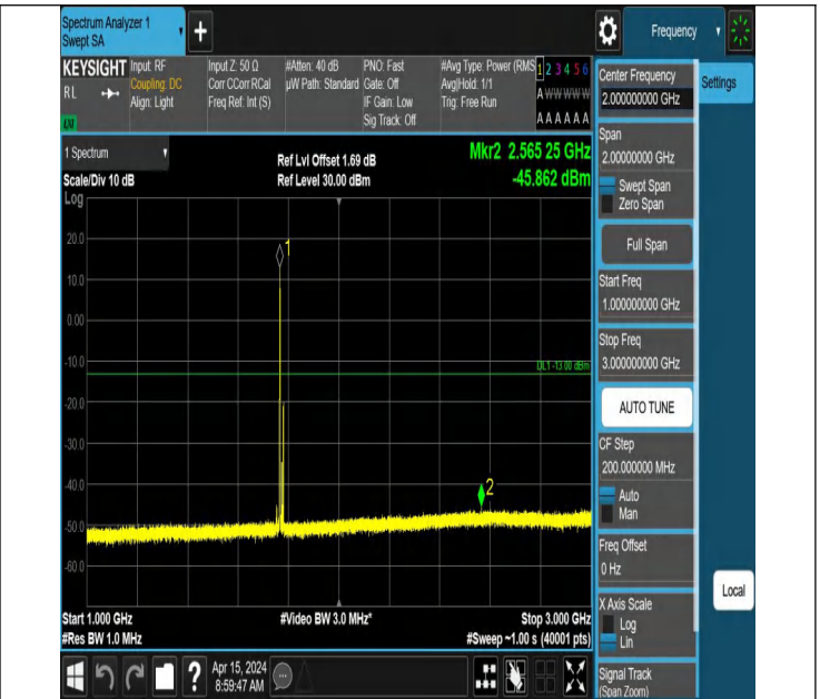
66-66-10MHz-5MHz-QPSK-QPSK-132572-132644-1RB#0-1RB# 24-1000~3000MHz-PASS
