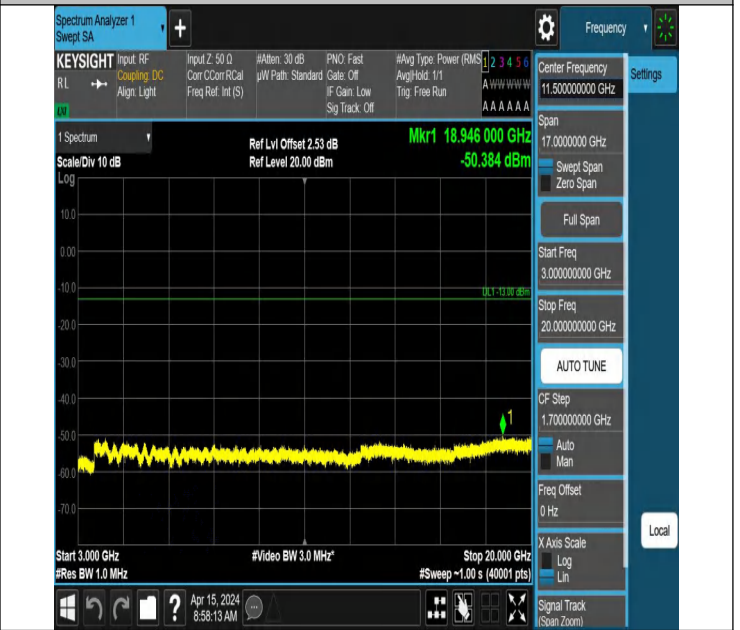
66-66-10MHz-5MHz-QPSK-QPSK-132397-132469-1RB#0-1RB# 24-3000~20000MHz-PASS
