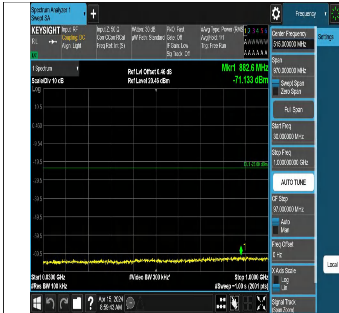
66-66-10MHz-5MHz-QPSK-QPSK-132572-132644-1RB#0-1RB# 24-30~1000MHz-PASS
