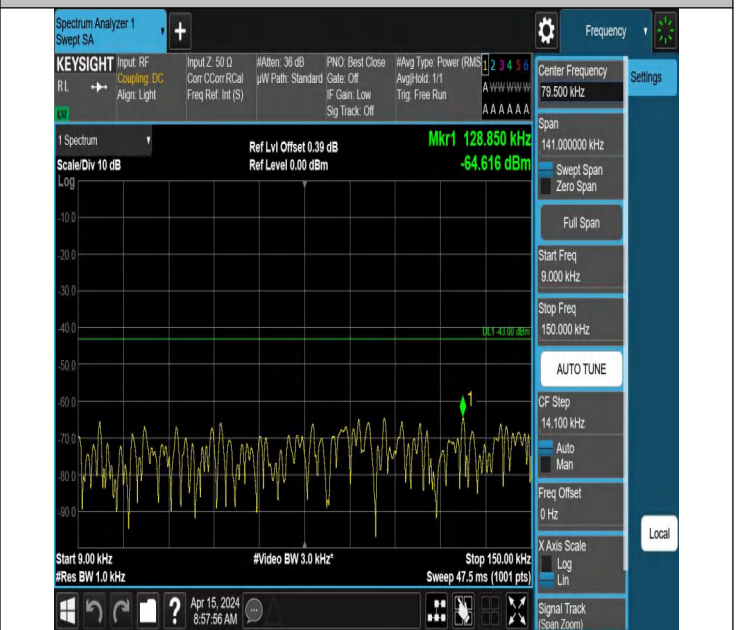
66-66-10MHz-5MHz-QPSK-QPSK-132397-132469-1RB#0-1RB# 24-0.009~0.15MHz-PASS
