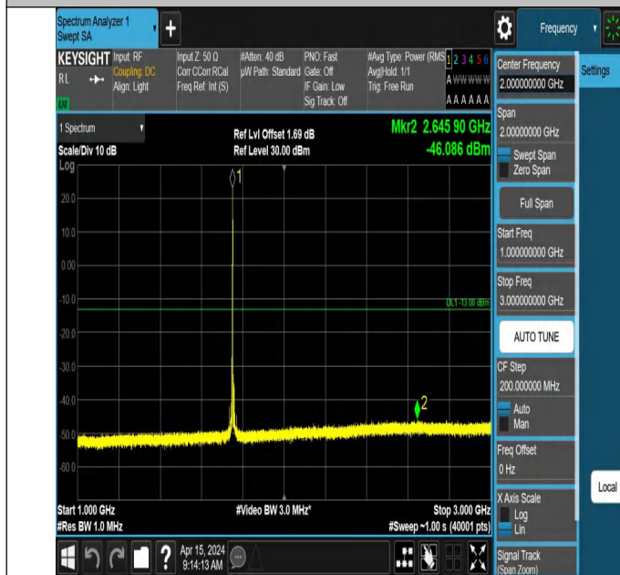
66-66-5MHz-15MHz-QPSK-QPSK-132353-132446-1RB#24-0RB #0-1000~3000MHz-PASS
