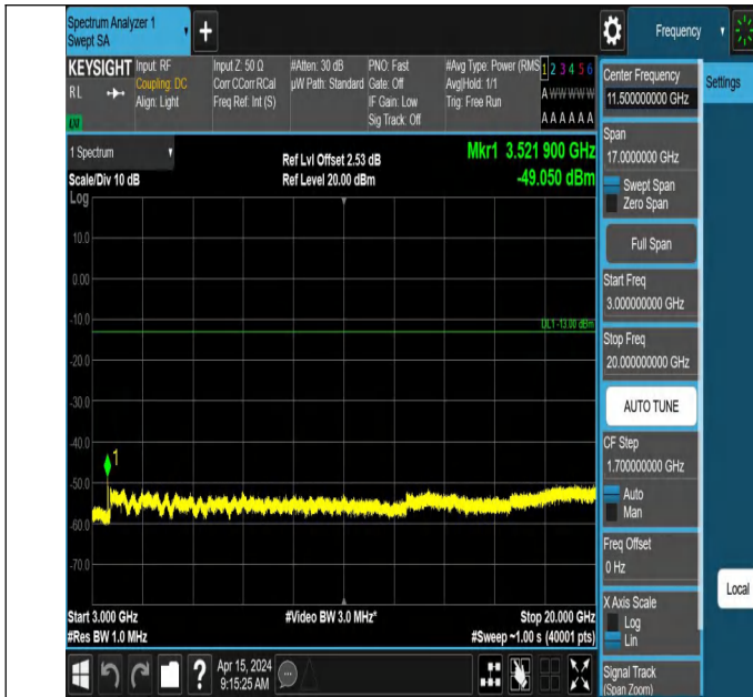
66-66-5MHz-15MHz-QPSK-QPSK-132504-132597-1RB#0-0RB# 0-3000~20000MHz-PASS
