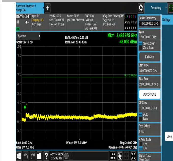
66-66-10MHz-5MHz-QPSK-QPSK-132397-132469-1RB#0-0RB# 0-3000~20000MHz-PASS
