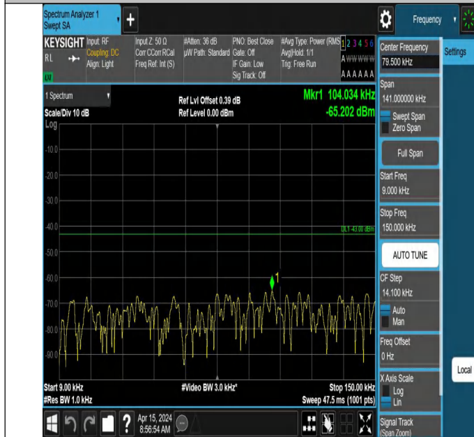
66-66-10MHz-5MHz-QPSK-QPSK-132397-132469-1RB#0-0RB# 0-0.009~0.15MHz-PASS
