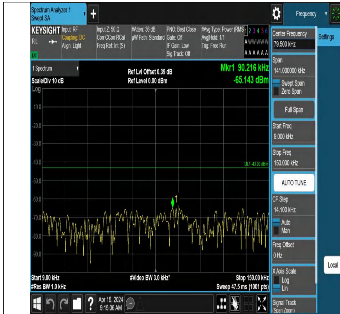
66-66-5MHz-15MHz-QPSK-QPSK-132504-132597-1RB#0-0RB# 0-0.009~0.15MHz-PASS
