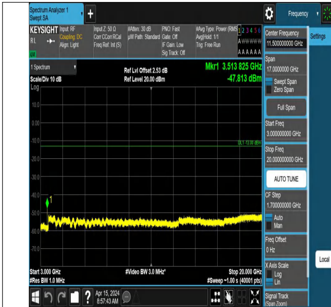
66-66-10MHz-5MHz-QPSK-QPSK-132397-132469-1RB#49-0RB# #0-3000~20000MHz-PASS
