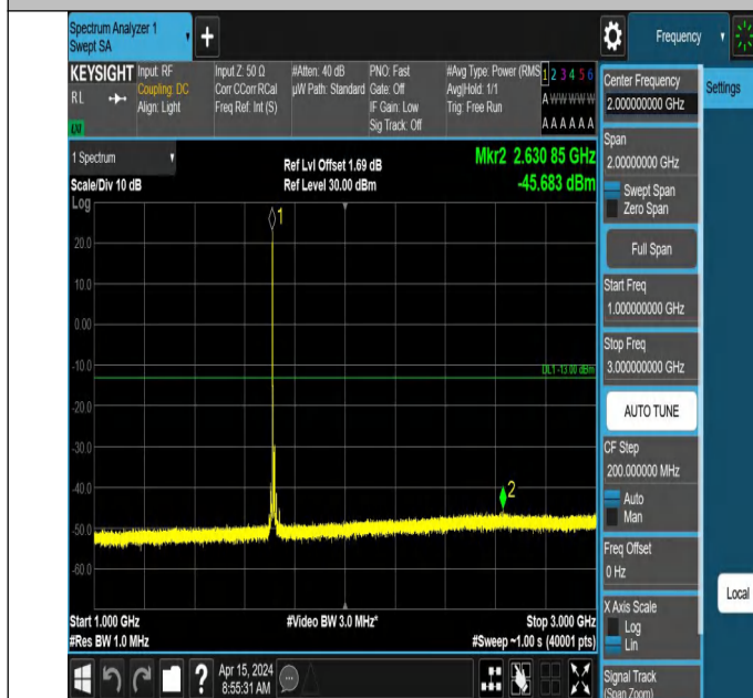
66-66-10MHz-5MHz-QPSK-QPSK-132022-132094-1RB#0-0RB# 0-1000~3000MHz-PASS
