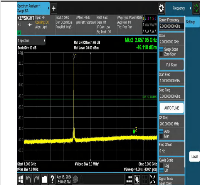
66-66-5MHz-5MHz-QPSK-QPSK-132398-132446-1RB#0-0RB#0-1000~3000MHz-PASS
