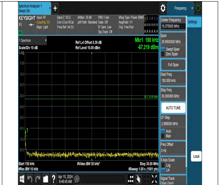
66-66-5MHz-10MHz-QPSK-QPSK-132375-132447-1RB#0-0RB# 0-0.15~30MHz-PASS
