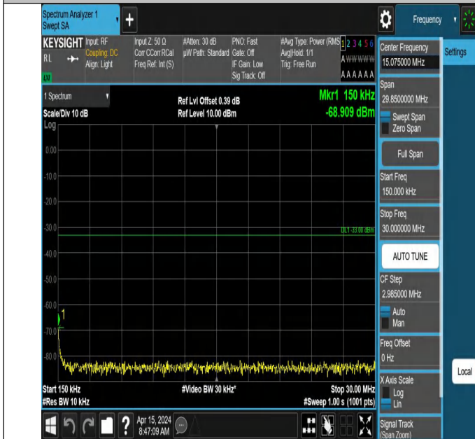
66-66-5MHz-10MHz-QPSK-QPSK-132000-132072-1RB#0-0RB# 0-0.15~30MHz-PASS
