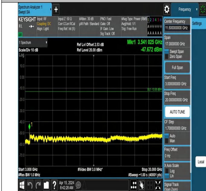
66-66-5MHz-5MHz-QPSK-QPSK-132599-132647-1RB#0-0RB#0-3000~20000MHz-PASS
