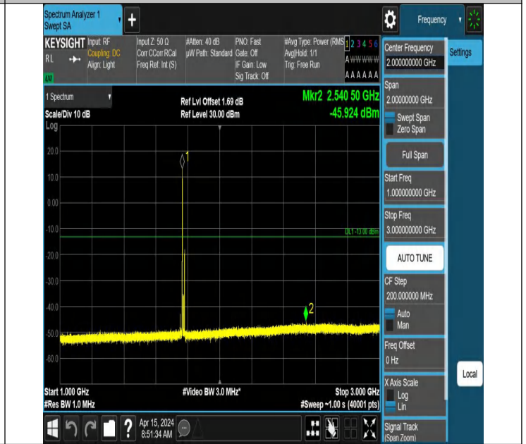
66-66-5MHz-10MHz-QPSK-QPSK-132550-132622-1RB#0-1RB# 49-1000~3000MHz-PASS
