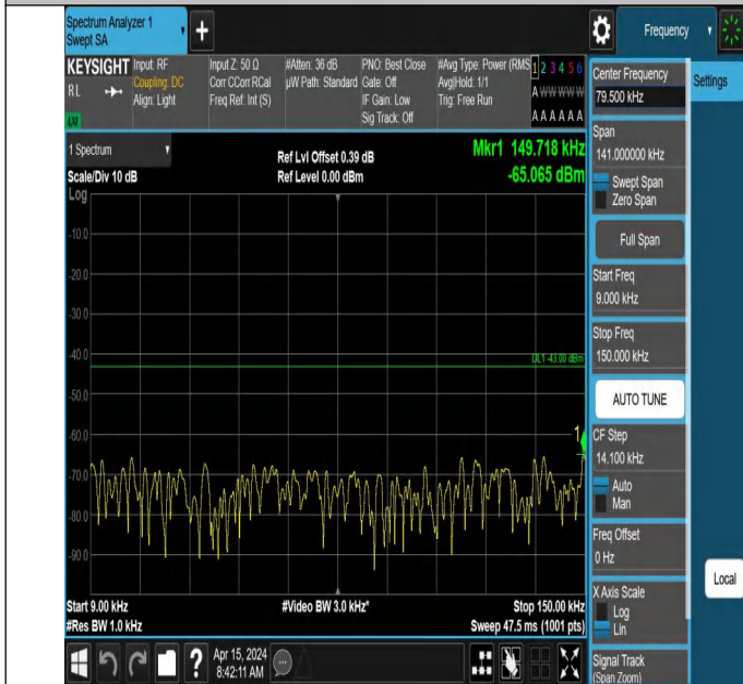
66-66-5MHz-5MHz-QPSK-QPSK-132599-132647-1RB#0-0RB#0- 0.009~0.15MHz-PASS
