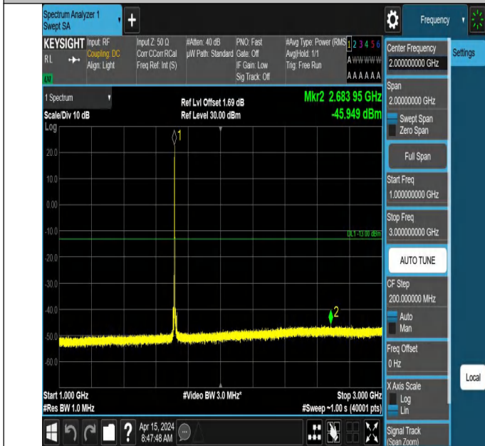
66-66-5MHz-10MHz-QPSK-QPSK-132000-132072-1RB#24-0RB #0-1000~3000MHz-PASS
