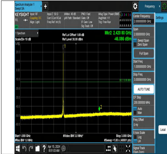
66-66-5MHz-10MHz-QPSK-QPSK-132550-132622-1RB#24-0RB #0-1000~3000MHz-PASS
