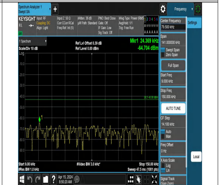
66-66-5MHz-10MHz-QPSK-QPSK-132550-132622-1RB#0-0RB# 0-0.009~0.15MHz-PASS
