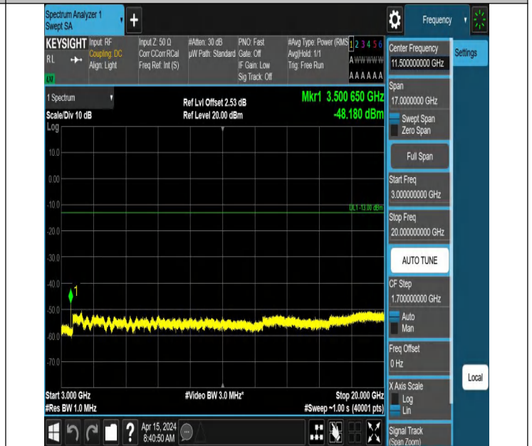
66-66-5MHz-5MHz-QPSK-QPSK-132398-132446-1RB#0-0RB#0-3000~20000MHz-PASS
