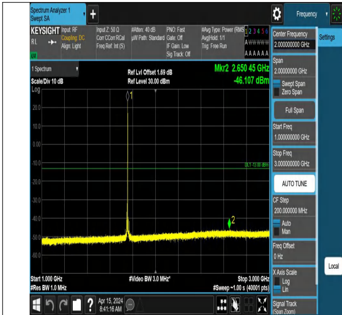
66-66-5MHz-5MHz-QPSK-QPSK-132398-132446-1RB#24-0RB# 0-1000~3000MHz-PASS
