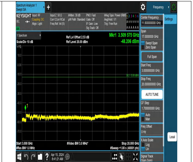
66-66-5MHz-5MHz-QPSK-QPSK-132398-132446-1RB#24-0RB# 0-3000~20000MHz-PASS
