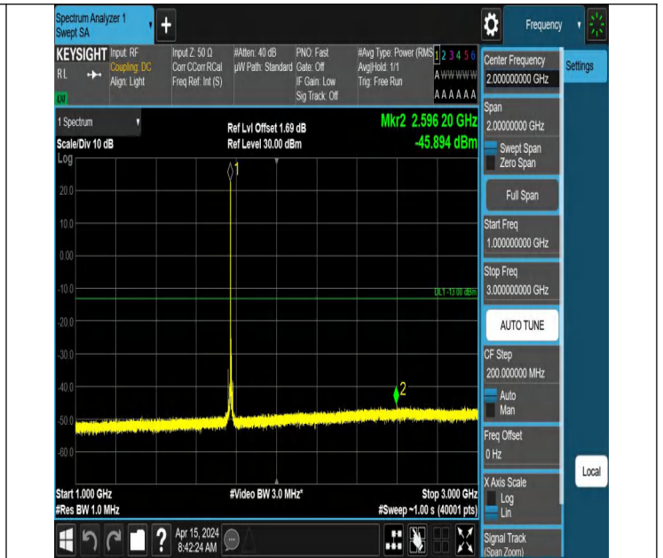
66-66-5MHz-5MHz-QPSK-QPSK-132599-132647-1RB#0-0RB#0-1000~3000MHz-PASS
