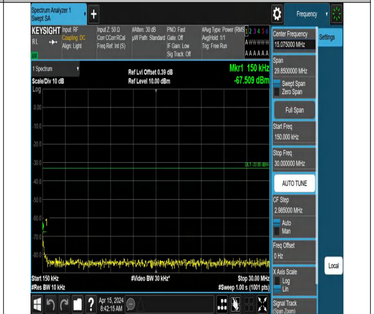
66-66-5MHz-5MHz-QPSK-QPSK-132599-132647-1RB#0-0RB#0- 0.15~30MHz-PASS
