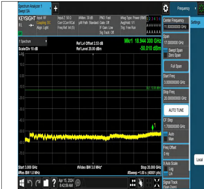
66-66-5MHz-5MHz-QPSK-QPSK-132599-132647-1RB#24-0RB# 0-3000~20000MHz-PASS
