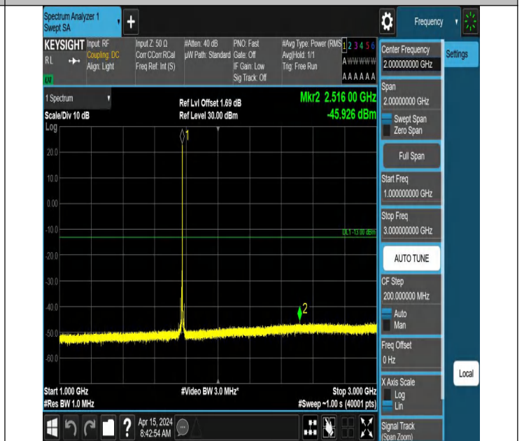
66-66-5MHz-5MHz-QPSK-QPSK-132599-132647-1RB#24-0RB# 0-1000~3000MHz-PASS
