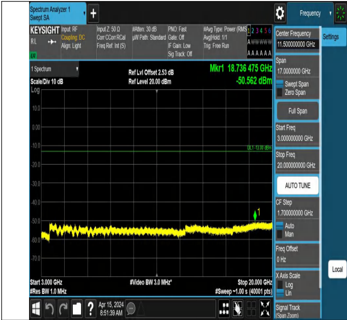
66-66-5MHz-10MHz-QPSK-QPSK-132550-132622-1RB#0-1RB# 49-3000~20000MHz-PASS
