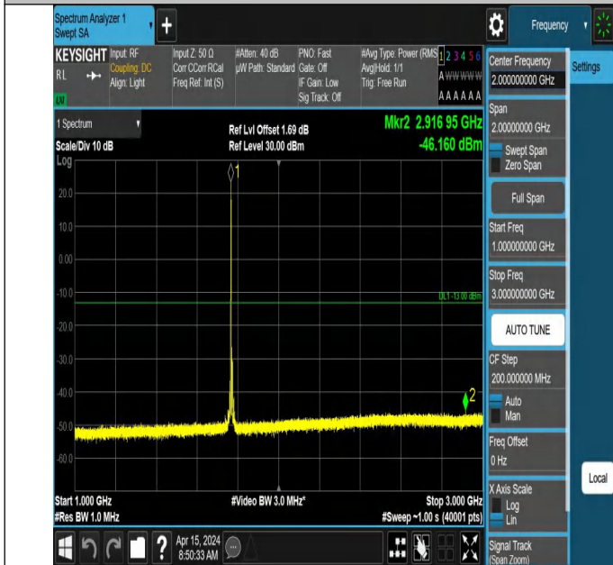
66-66-5MHz-10MHz-QPSK-QPSK-132550-132622-1RB#0-0RB# 0-1000~3000MHz-PASS
