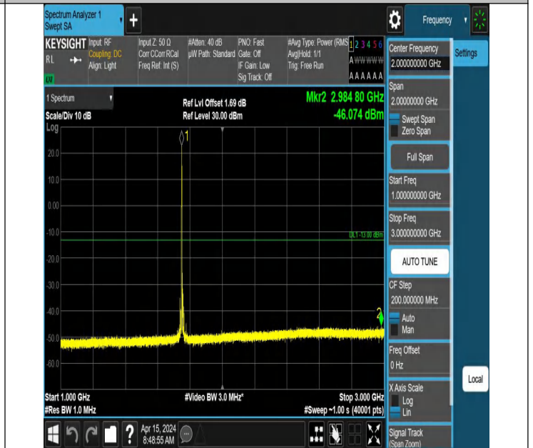
66-66-5MHz-10MHz-QPSK-QPSK-132375-132447-1RB#0-0RB# 0-1000~3000MHz-PASS
