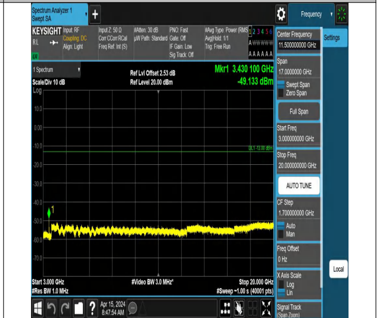
66-66-5MHz-10MHz-QPSK-QPSK-132000-132072-1RB#24-0RB #0-3000~20000MHz-PASS
