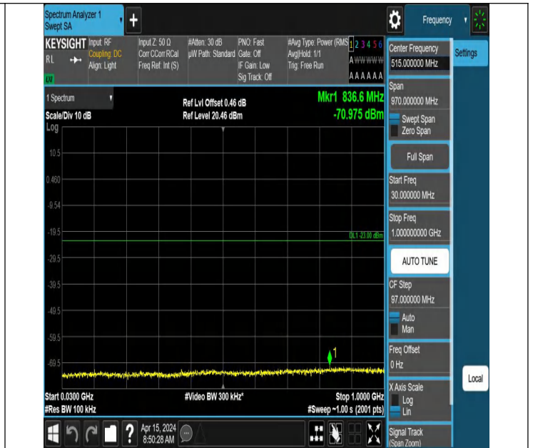
66-66-5MHz-10MHz-QPSK-QPSK-132550-132622-1RB#0-0RB# 0-30~1000MHz-PASS
