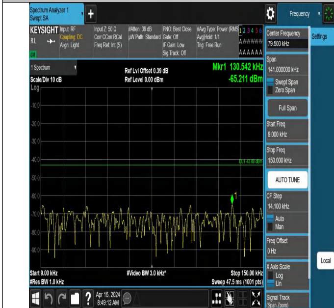
66-66-5MHz-10MHz-QPSK-QPSK-132375-132447-1RB#24-0RB #0-0.009~0.15MHz-PASS
