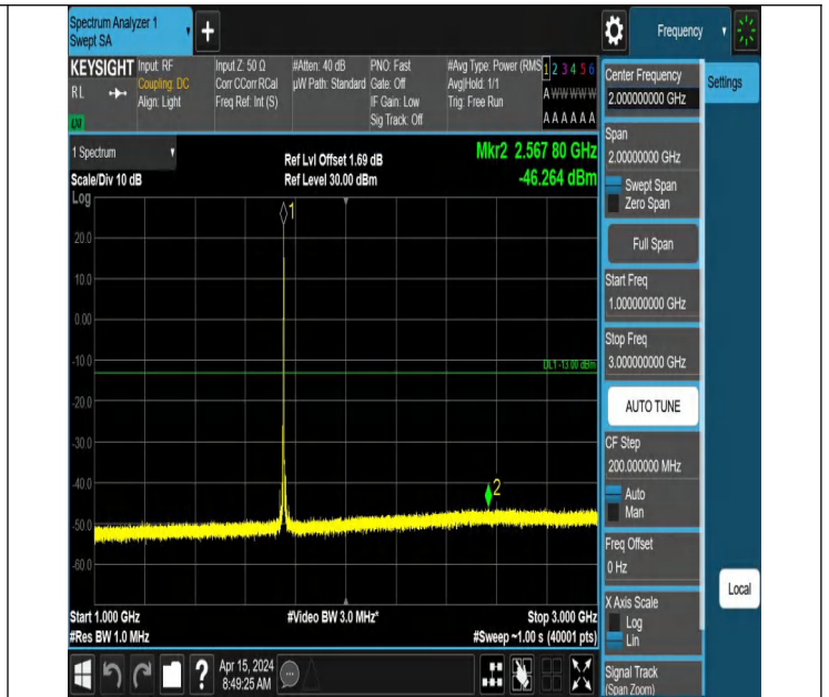
66-66-5MHz-10MHz-QPSK-QPSK-132375-132447-1RB#24-0RB #0-1000~3000MHz-PASS
