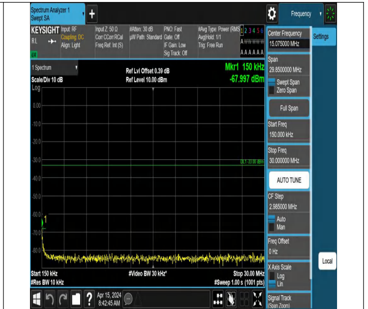
66-66-5MHz-5MHz-QPSK-QPSK-132599-132647-1RB#24-0RB# 0-0.15~30MHz-PASS
