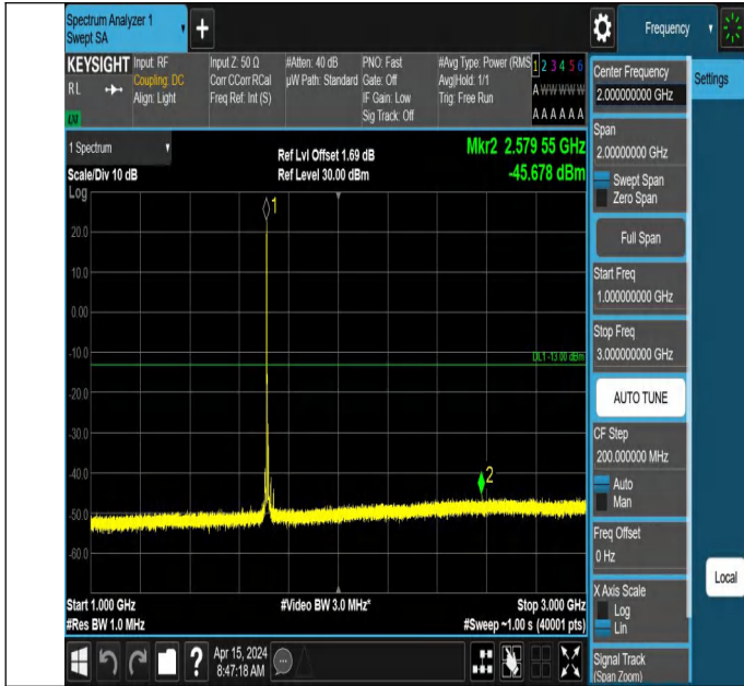
66-66-5MHz-10MHz-QPSK-QPSK-132000-132072-1RB#0-0RB#
