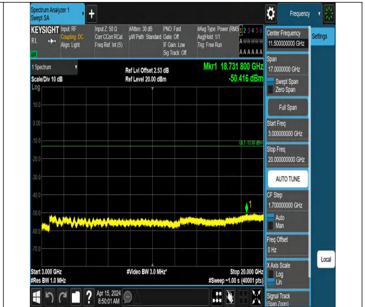
66-66-5MHz-10MHz-QPSK-QPSK-132375-132447-1RB#0-1RB# 49-3000~20000MHz-PASS
