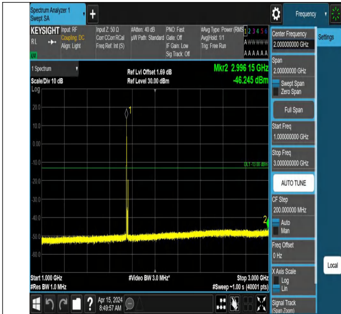
66-66-5MHz-10MHz-QPSK-QPSK-132375-132447-1RB#0-1RB# 49-1000~3000MHz-PASS
