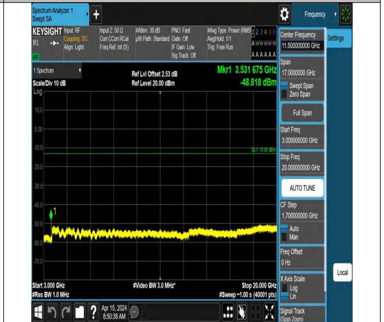
66-66-5MHz-10MHz-QPSK-QPSK-132550-132622-1RB#0-0RB# 0-3000~20000MHz-PASS
