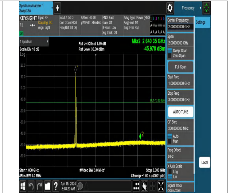
66-66-5MHz-10MHz-QPSK-QPSK-132000-132072-1RB#0-1RB#
