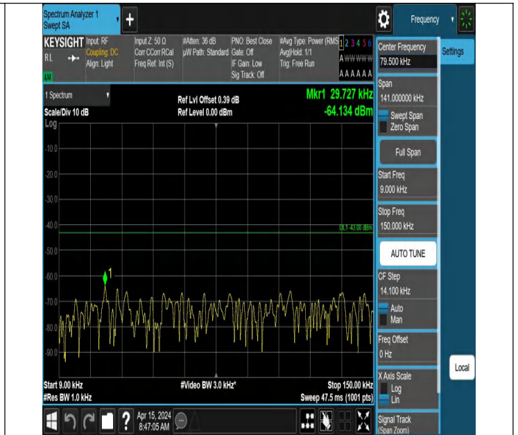
66-66-5MHz-10MHz-QPSK-QPSK-132000-132072-1RB#0-0RB# 0-0.009~0.15MHz-PASS
