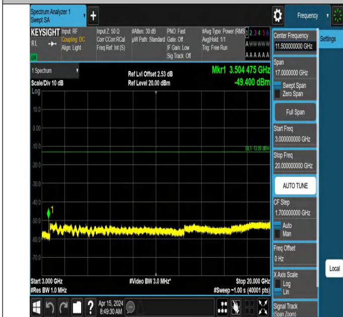
66-66-5MHz-10MHz-QPSK-QPSK-132375-132447-1RB#24-0RB #0-3000~20000MHz-PASS
