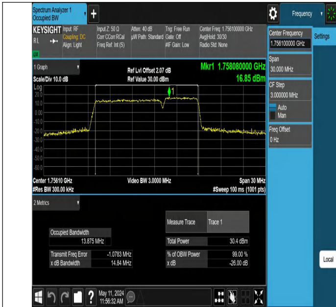
66-66-10MHz-5MHz-QPSK-QPSK-132397-132469-50RB#0-25RB #0-PASS
