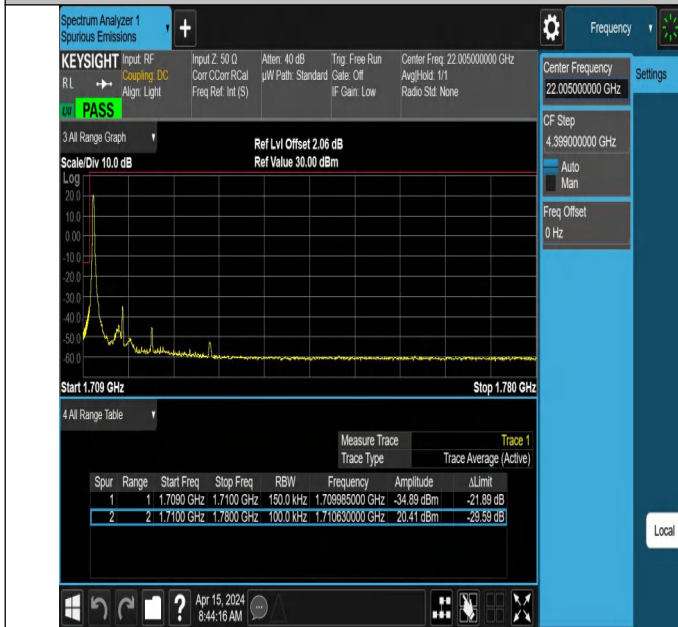
5MHz-10MHz_QPSK@QPSK-QPSK@QPSK_132000-132072_1 RB#0@25RB#0-0RB#0@50RB#0
