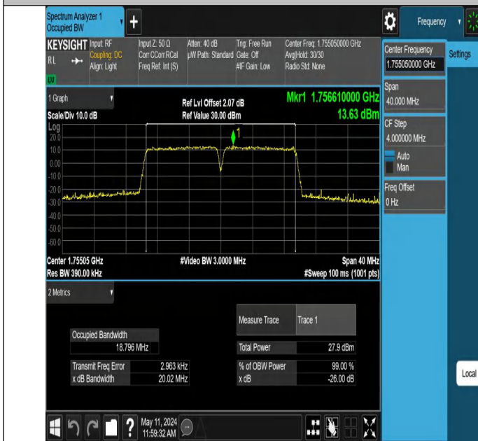
66-66-10MHz-10MHz-256QAM-256QAM-132373-132472-50RB#0-50R B#0-PASS
