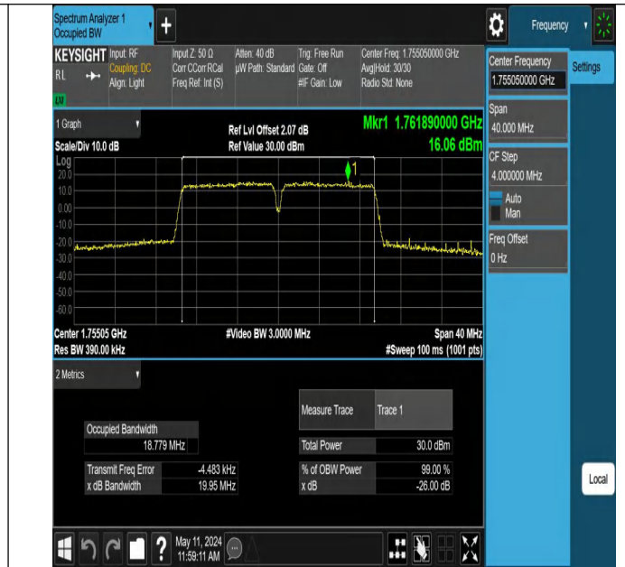
66-66-10MHz-10MHz-64QAM-64QAM-132373-132472-50RB#0-50R B#0-PASS
