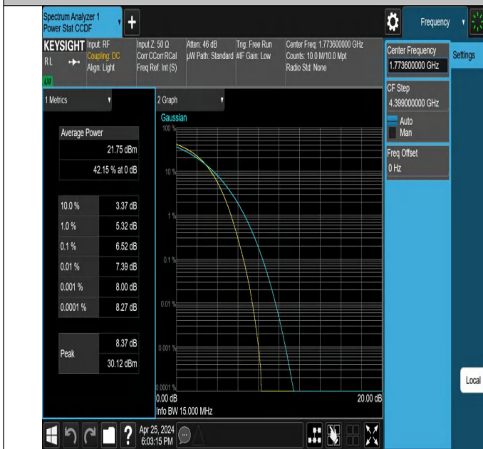
66-66-10MHz-5MHz-QPSK-QPSK-132572-132644-50RB#0-25R
