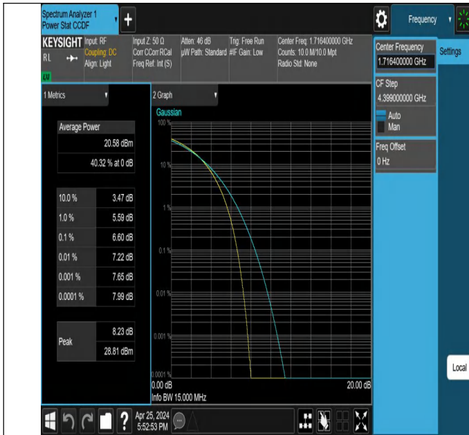
66-66-5MHz-10MHz-QPSK-QPSK-132000-132072-25RB#0-50R
