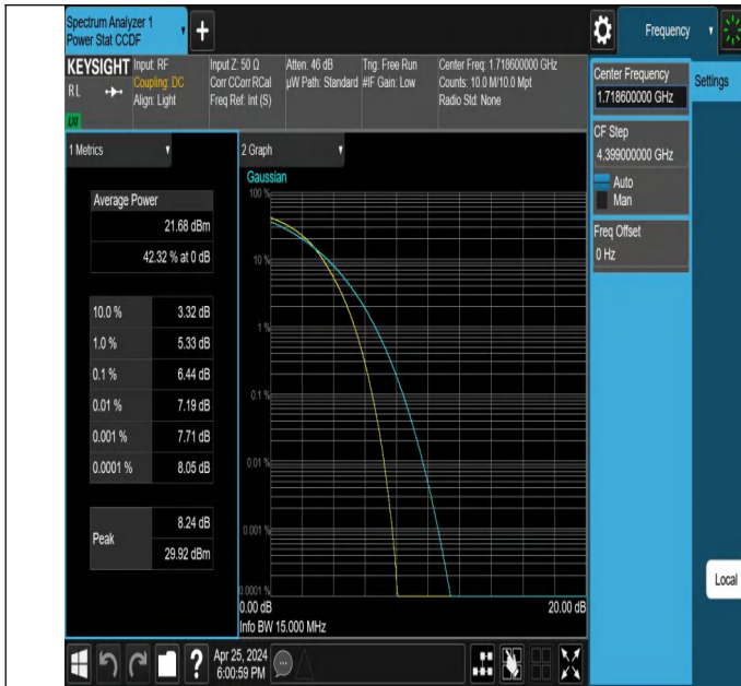
66-66-10MHz-5MHz-QPSK-QPSK-132022-132094-50RB#0-25R
