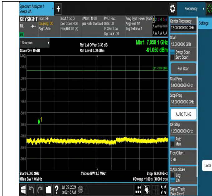
42-42(3450-3550)-20MHz-20MHz-QPSK-QPSK-42792-42990-1R B#99-0RB#0-6000~18000MHz-PASS
