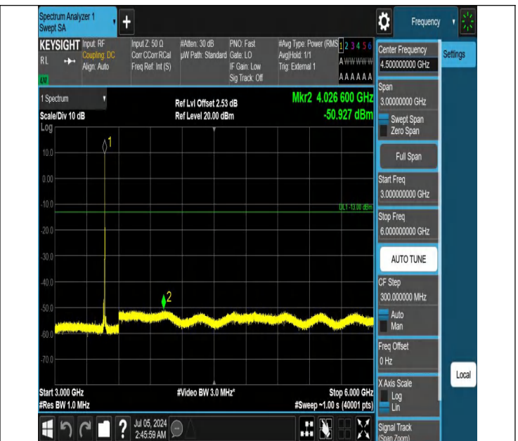
42-42(3450-3550)-20MHz-20MHz-QPSK-QPSK-42190-42388-1R B#99-0RB#0-3000~6000MHz-PASS
