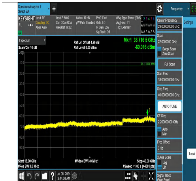
42-42(3450-3550)-20MHz-20MHz-QPSK-QPSK-42190-42388-1R B#0-0RB#0-18000~40000MHz-PASS
