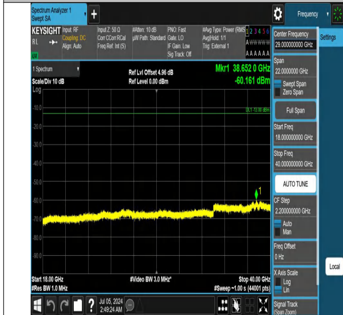
42-42(3450-3550)-20MHz-20MHz-QPSK-QPSK-42190-42388-1R B#0-1RB#99-18000~40000MHz-PASS
