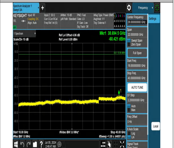
42-42(3450-3550)-20MHz-20MHz-QPSK-QPSK-42190-42388-1R B#99-0RB#0-18000~40000MHz-PASS
