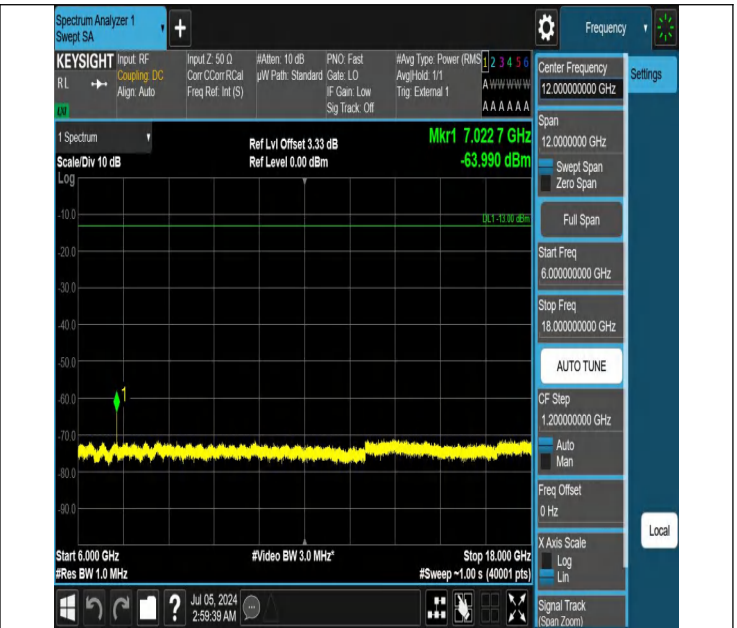
42-42(3450-3550)-20MHz-20MHz-QPSK-QPSK-42792-42990-1R B#0-ORB#0-6000~18000MHz-PASS
