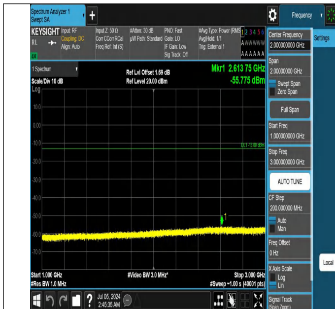
42-42(3450-3550)-20MHz-20MHz-QPSK-QPSK-42190-42388-1R B#99-0RB#0-1000~3000MHz-PASS
