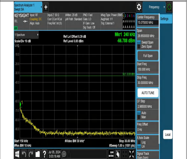
42-42(3450-3550)-20MHz-20MHz-QPSK-QPSK-42792-42990-1R B#0-1RB#99-0.15~30MHz-PASS
