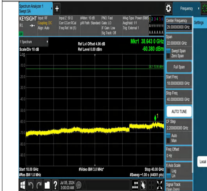
42-42(3450-3550)-20MHz-20MHz-QPSK-QPSK-42792-42990-1R B#0-ORB#0-18000~40000MHz-PASS
