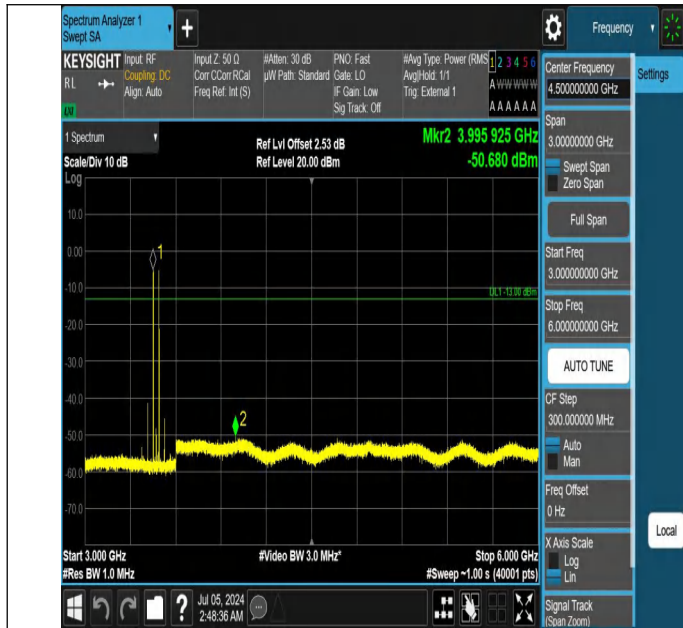
42-42(3450-3550)-20MHz-20MHz-QPSK-QPSK-42190-42388-1R B#0-1RB#99-3000~6000MHz-PASS
