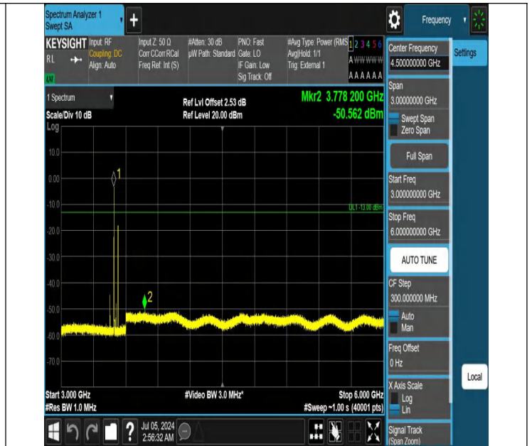
42-42(3450-3550)-20MHz-20MHz-QPSK-QPSK-42590-42788-1R B#0-1RB#99-3000~6000MHz-PASS
