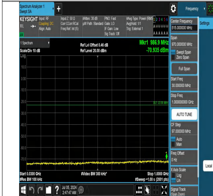
42-42(3450-3550)-20MHz-20MHz-QPSK-QPSK-42190-42388-1R B#0-1RB#99-30~1000MHz-PASS
