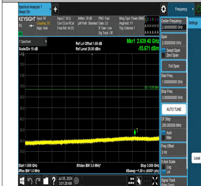
42-42(3450-3550)-20MHz-20MHz-QPSK-QPSK-42792-42990-1R B#99-ORB#0-1000~3000MHz-PASS
