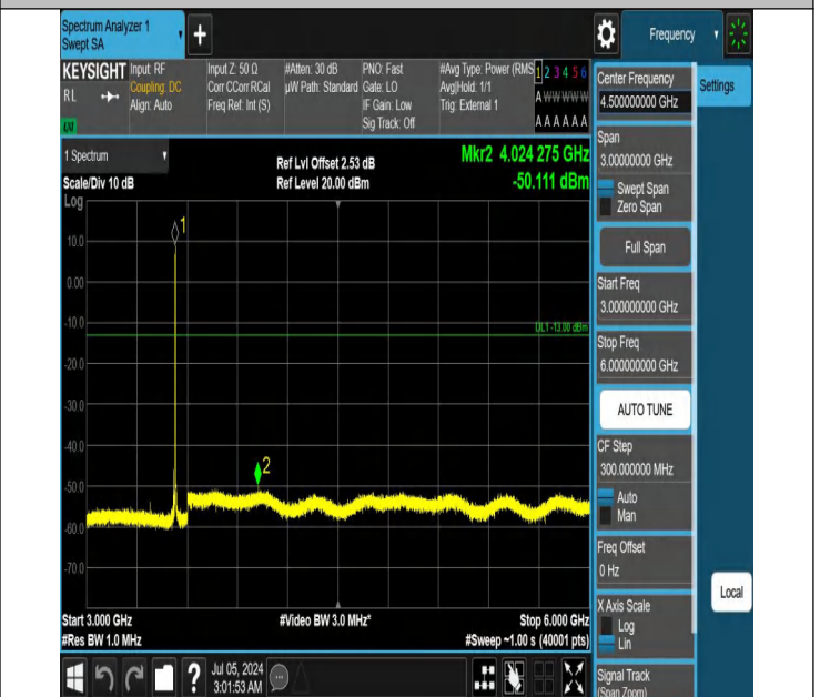
42-42(3450-3550)-20MHz-20MHz-QPSK-QPSK-42792-42990-1R B#99-ORB#0-3000~6000MHz-PASS
