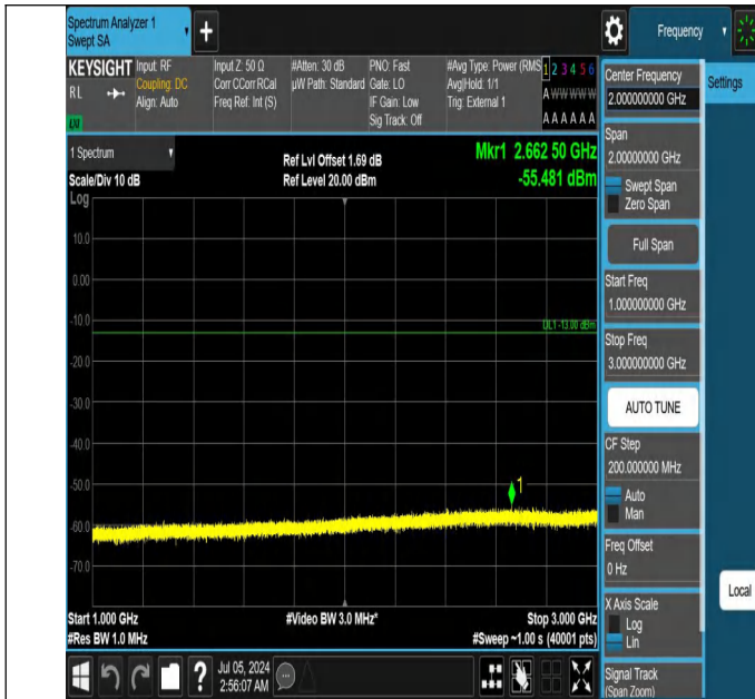
42-42(3450-3550)-20MHz-20MHz-QPSK-QPSK-42590-42788-1R B#0-1RB#99-1000~3000MHz-PASS
