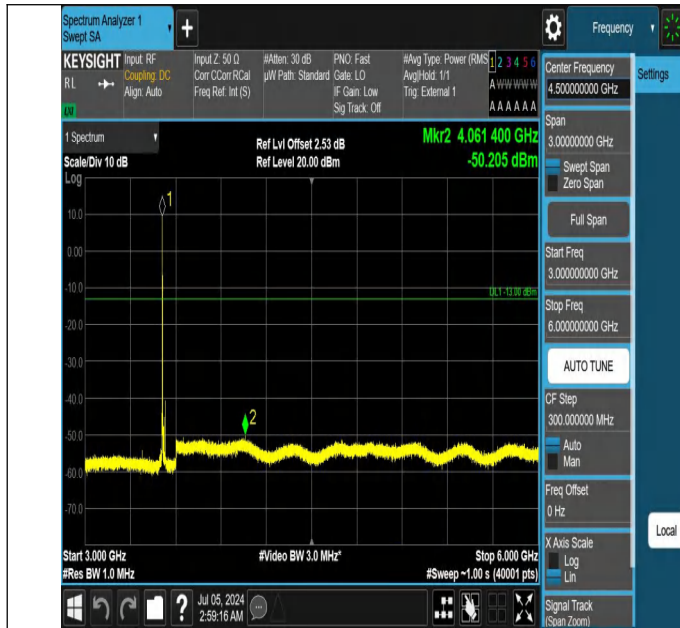
42-42(3450-3550)-20MHz-20MHz-QPSK-QPSK-42792-42990-1R B#0-ORB#0-3000~6000MHz-PASS
