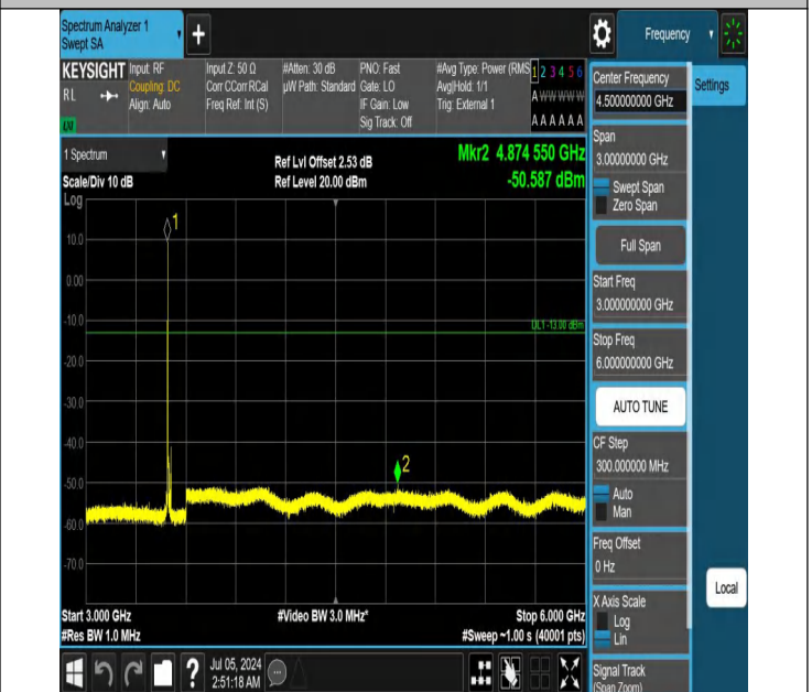
42-42(3450-3550)-20MHz-20MHz-QPSK-QPSK-42590-42788-1R B#0-ORB#0-3000~6000MHz-PASS
