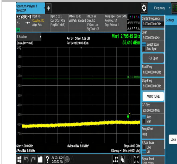
42-42(3450-3550)-20MHz-20MHz-QPSK-QPSK-42590-42788-1R B#0-ORB#0-1000~3000MHz-PASS
