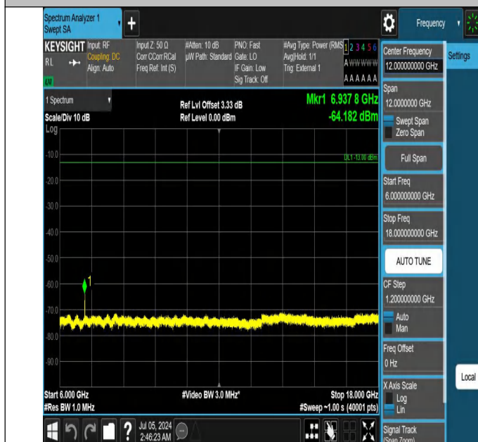
42-42(3450-3550)-20MHz-20MHz-QPSK-QPSK-42190-42388-1R B#99-0RB#0-6000~18000MHz-PASS
