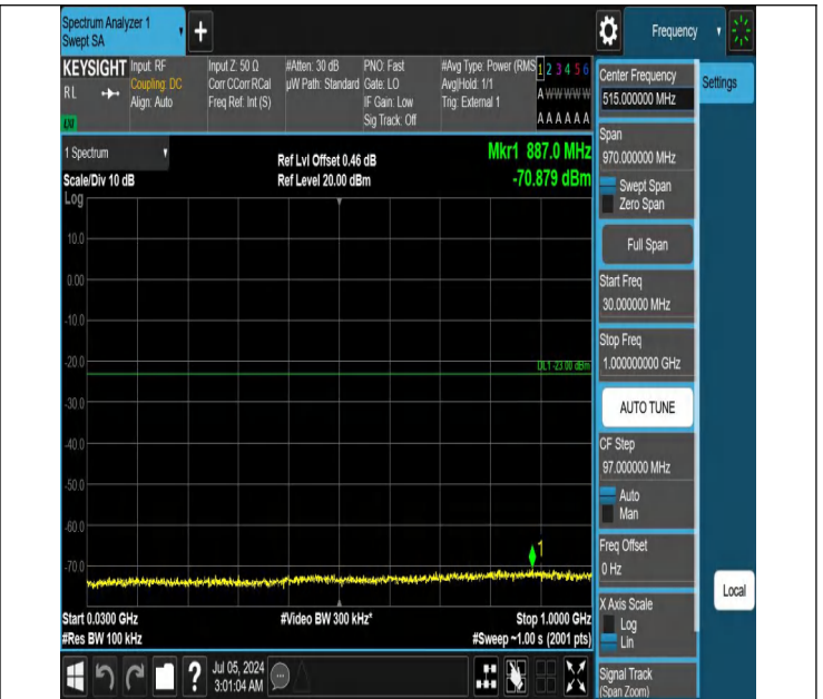
42-42(3450-3550)-20MHz-20MHz-QPSK-QPSK-42792-42990-1R B#99-ORB#0-30~1000MHz-PASS
