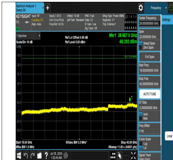
42-42(3450-3550)-10MHz-20MHz-QPSK-QPSK-42140-42284-1R B#0-1RB#99-18000~40000MHz-PASS
