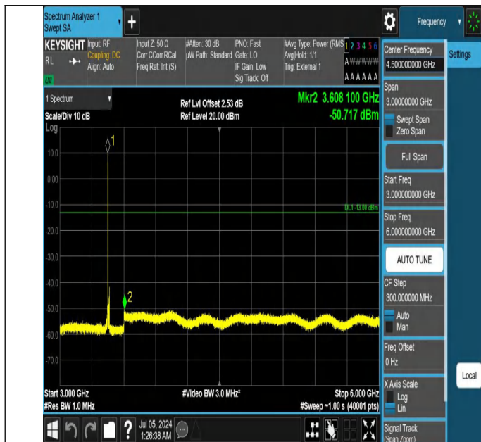
42-42(3450-3550)-10MHz-20MHz-QPSK-QPSK-42140-42284-1R B#0-0RB#0-3000~6000MHz-PASS
