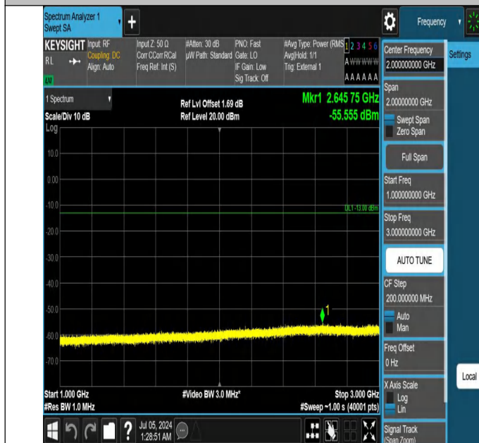
42-42(3450-3550)-10MHz-20MHz-QPSK-QPSK-42140-42284-1R B#49-ORB#0-1000~3000MHz-PASS
