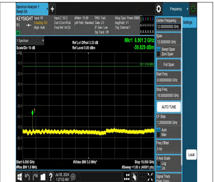
42-42(3450-3550)-10MHz-20MHz-QPSK-QPSK-42140-42284-1R B#0-0RB#0-6000~18000MHz-PASS
