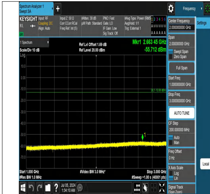
42-42(3450-3550)-10MHz-20MHz-QPSK-QPSK-42590-42734-1R B#0-ORB#0-1000~3000MHz-PASS
