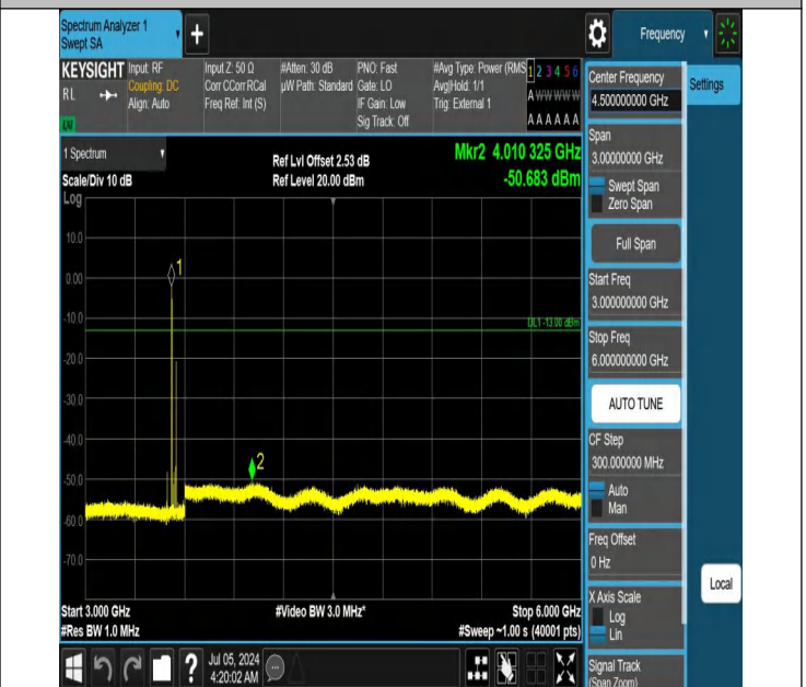
42-42(3450-3550)-20MHz-10MHz-QPSK-QPSK-42896-43040-1R B#0-1RB#49-3000~6000MHz-PASS
