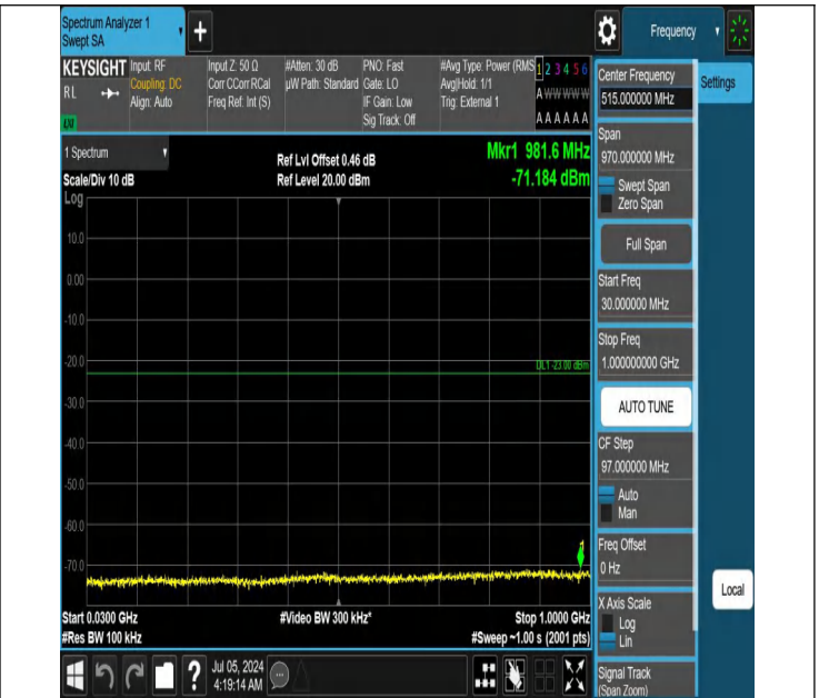
42-42(3450-3550)-20MHz-10MHz-QPSK-QPSK-42896-43040-1R B#0-1RB#49-30~1000MHz-PASS
