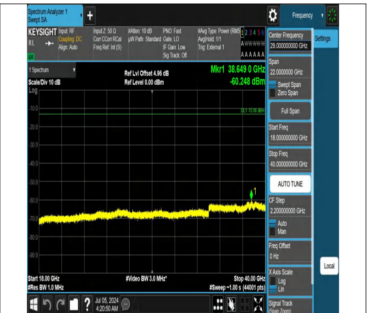
42-42(3450-3550)-20MHz-10MHz-QPSK-QPSK-42896-43040-1R B#0-1RB#49-18000~40000MHz-PASS
