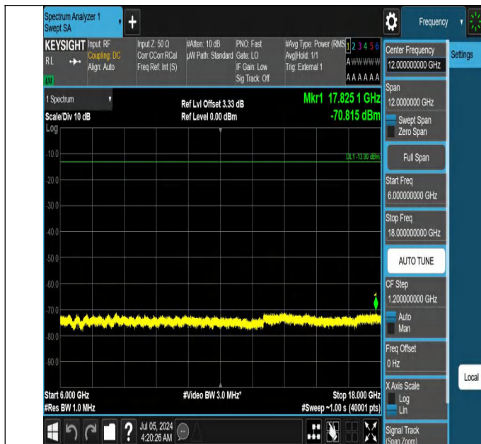
42-42(3450-3550)-20MHz-10MHz-QPSK-QPSK-42896-43040-1R B#0-1RB#49-6000~18000MHz-PASS
