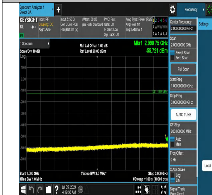
42-42(3450-3550)-20MHz-10MHz-QPSK-QPSK-42896-43040-1R B#0-1RB#49-1000~3000MHz-PASS
