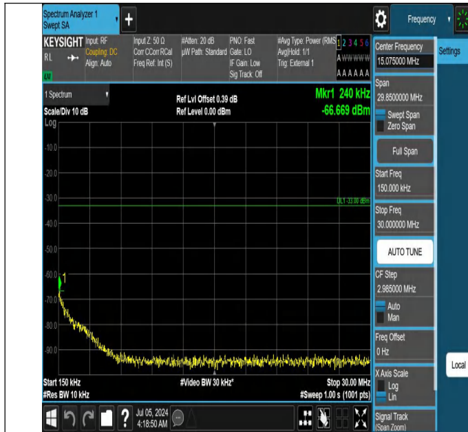
42-42(3450-3550)-20MHz-10MHz-QPSK-QPSK-42896-43040-1R B#0-1RB#49-0.15~30MHz-PASS
