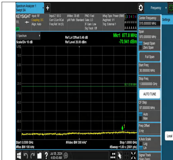
42-42(3450-3550)-20MHz-10MHz-QPSK-QPSK-42190-42334-1R B#99-0RB#0-30~1000MHz-PASS
