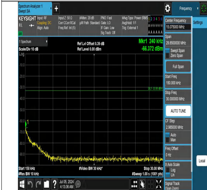
42-42(3450-3550)-20MHz-10MHz-QPSK-QPSK-42896-43040-1R B#0-0RB#0-0.15~30MHz-PASS
