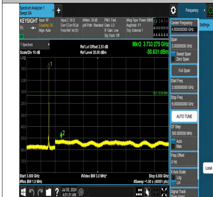
42-42(3450-3550)-20MHz-10MHz-QPSK-QPSK-42190-42334-1R B#99-0RB#0-3000~6000MHz-PASS
