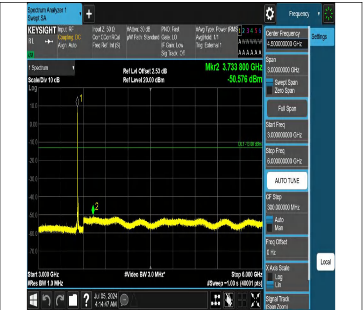
42-42(3450-3550)-20MHz-10MHz-QPSK-QPSK-42896-43040-1R B#0-ORB#0-3000~6000MHz-PASS
