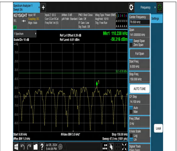
42-42(3450-3550)-20MHz-5MHz-QPSK-QPSK-42948-43065-1RB #99-0RB#0-0.009~0.15MHz-PASS
