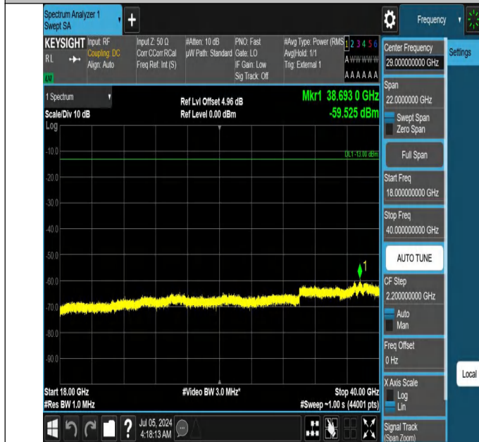
42-42(3450-3550)-20MHz-10MHz-QPSK-QPSK-42896-43040-1R B#99-ORB#0-18000~40000MHz-PASS
