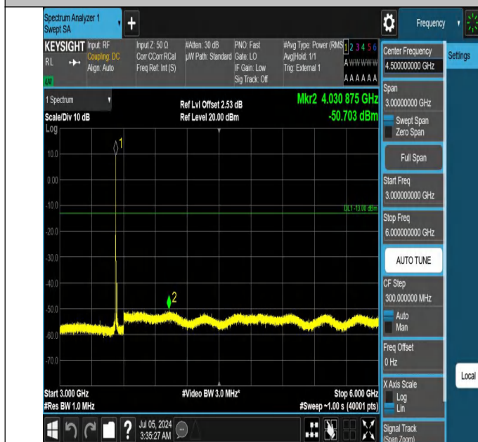
42-42(3450-3550)-20MHz-5MHz-QPSK-QPSK-42948-43065-1RB #0-0RB#0-3000~6000MHz-PASS
