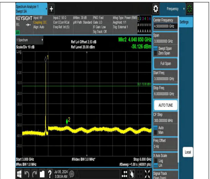
42-42(3450-3550)-20MHz-5MHz-QPSK-QPSK-42948-43065-1RB #99-0RB#0-3000~6000MHz-PASS
