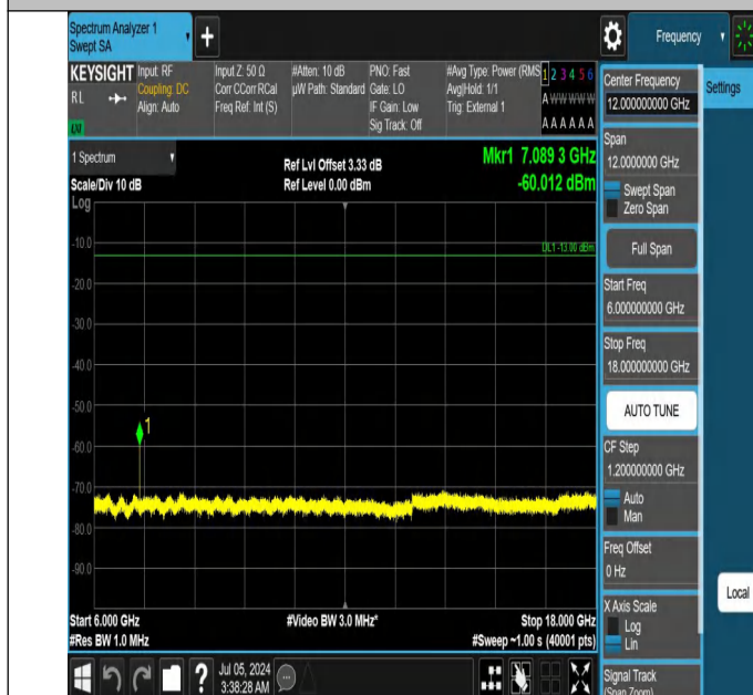
42-42(3450-3550)-20MHz-5MHz-QPSK-QPSK-42948-43065-1RB #99-0RB#0-6000~18000MHz-PASS
