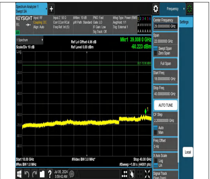
42-42(3450-3550)-20MHz-10MHz-QPSK-QPSK-42190-42334-1R B#0-0RB#0-18000~40000MHz-PASS
