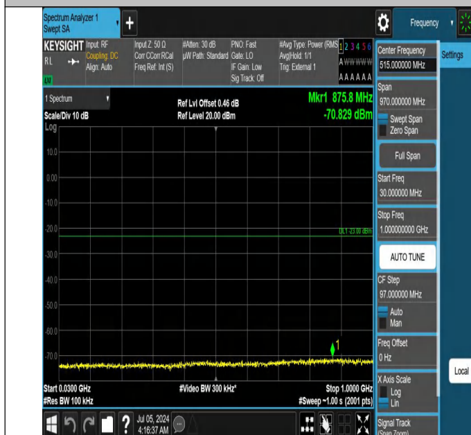
42-42(3450-3550)-20MHz-10MHz-QPSK-QPSK-42896-43040-1R B#99-0RB#0-30~1000MHz-PASS
