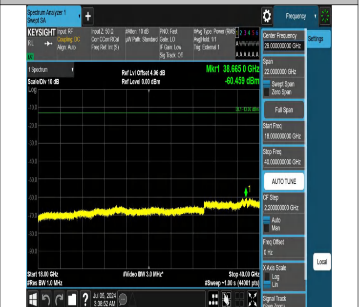
42-42(3450-3550)-20MHz-5MHz-QPSK-QPSK-42948-43065-1RB #99-0RB#0-18000~40000MHz-PASS
