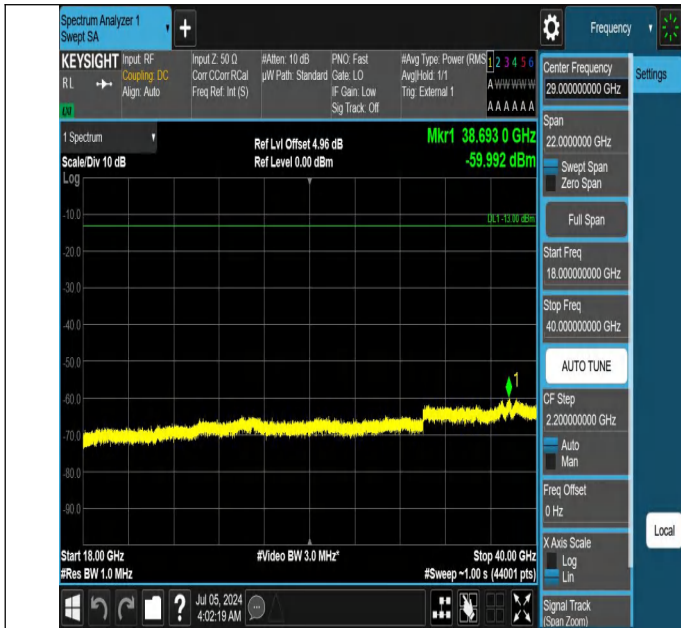
42-42(3450-3550)-20MHz-10MHz-QPSK-QPSK-42190-42334-1R B#99-0RB#0-18000~40000MHz-PASS
