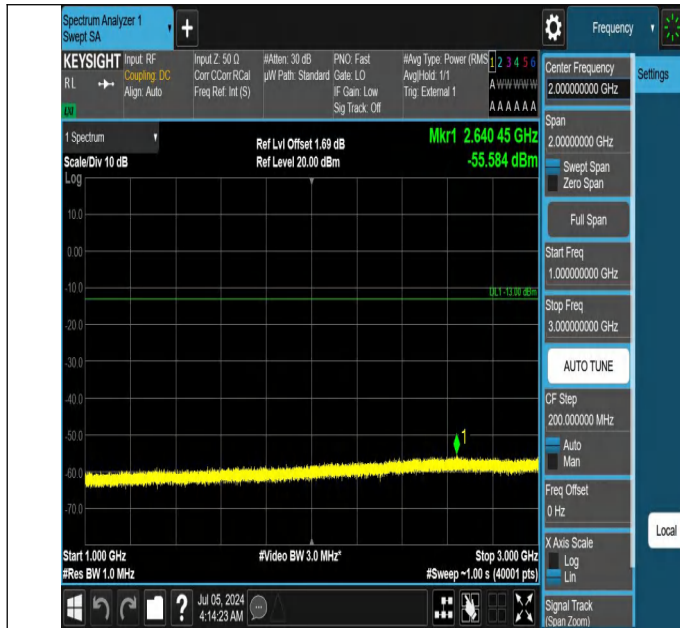
42-42(3450-3550)-20MHz-10MHz-QPSK-QPSK-42896-43040-1R B#0-ORB#0-1000~3000MHz-PASS
