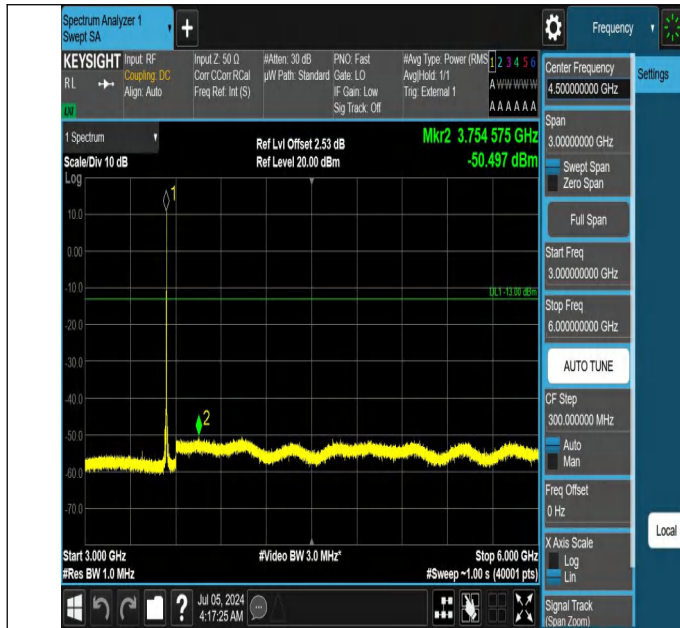
42-42(3450-3550)-20MHz-10MHz-QPSK-QPSK-42896-43040-1R B#99-ORB#0-3000~6000MHz-PASS
