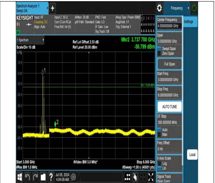
42-42(3450-3550)-20MHz-10MHz-QPSK-QPSK-42190-42334-1R B#0-1RB#49-3000~6000MHz-PASS
