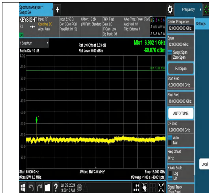
42-42(3450-3550)-20MHz-10MHz-QPSK-QPSK-42190-42334-1R B#0-0RB#0-6000~18000MHz-PASS
