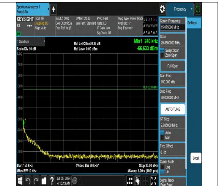
42-42(3450-3550)-20MHz-10MHz-QPSK-QPSK-42896-43040-1R B#99-0RB#0-0.15~30MHz-PASS
