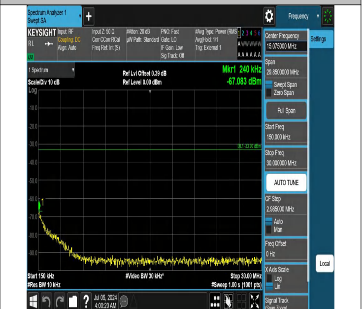
42-42(3450-3550)-20MHz-10MHz-QPSK-QPSK-42190-42334-1R B#99-0RB#0-0.15~30MHz-PASS
