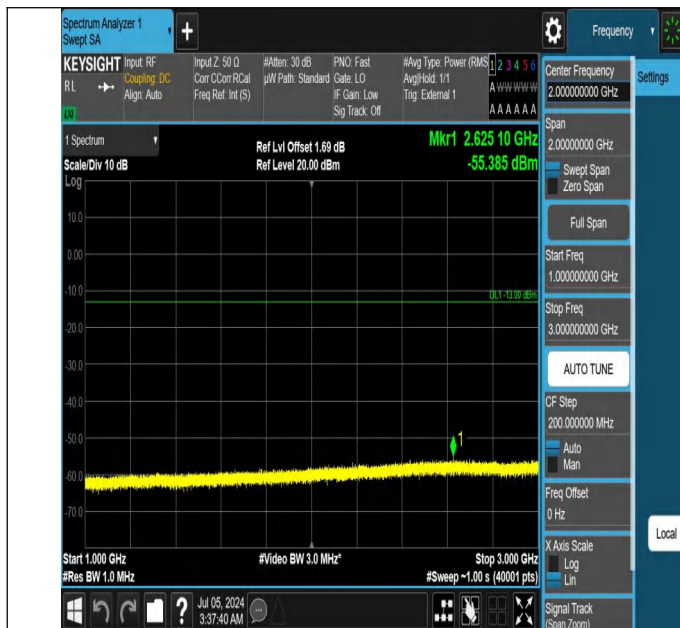
42-42(3450-3550)-20MHz-5MHz-QPSK-QPSK-42948-43065-1RB #99-0RB#0-1000~3000MHz-PASS
