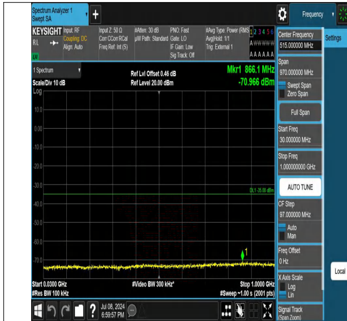
41-41-10MHz-20MHz-QPSK-QPSK-40526-40670-1RB#0-0RB#0-30~1000MHz-PASS
