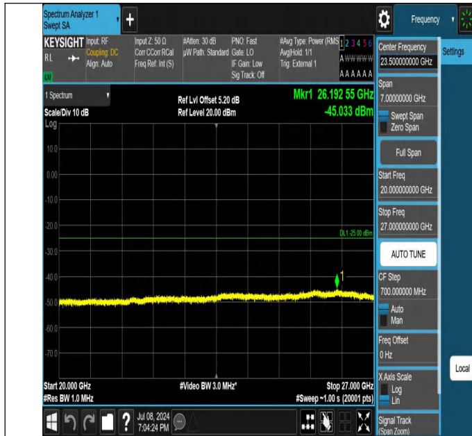
41-41-10MHz-20MHz-QPSK-QPSK-40526-40670-1RB#0-1RB#9 9-20000~27000MHz-PASS
