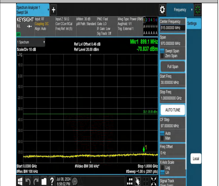
41-41-10MHz-20MHz-QPSK-QPSK-39705-39849-1RB#0-1RB#9 9-30~1000MHz-PASS
