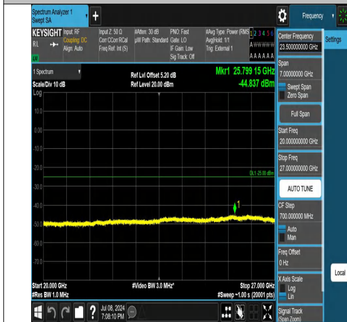
41-41-10MHz-20MHz-QPSK-QPSK-41346-41490-1RB#49-0RB# 0-20000~27000MHz-PASS
