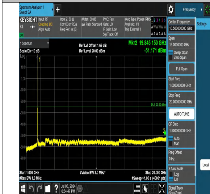
41-41-10MHz-20MHz-QPSK-QPSK-39705-39849-1RB#0-0RB#0-1000~20000MHz-PASS
