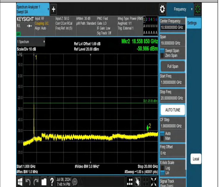
41-41-15MHz-20MHz-QPSK-QPSK-39728-39899-1RB#0-0RB#0- 1000~20000MHz-PASS
