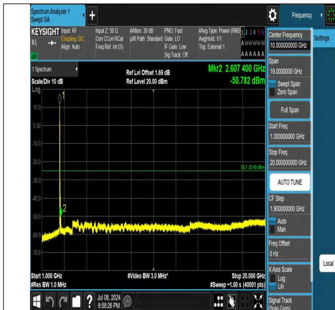
41-41-10MHz-20MHz-QPSK-QPSK-39705-39849-1RB#0-1RB#9 9-1000~20000MHz-PASS
