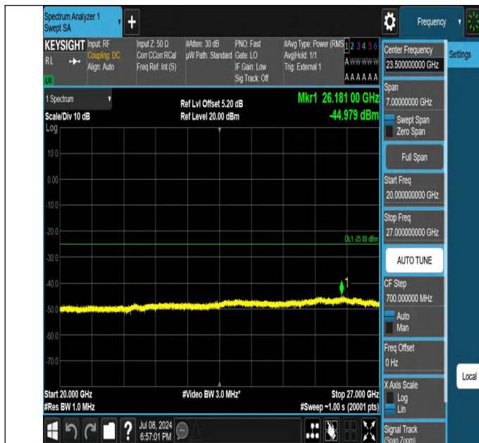
41-41-10MHz-20MHz-QPSK-QPSK-39705-39849-1RB#49-0RB# 0-20000~27000MHz-PASS
