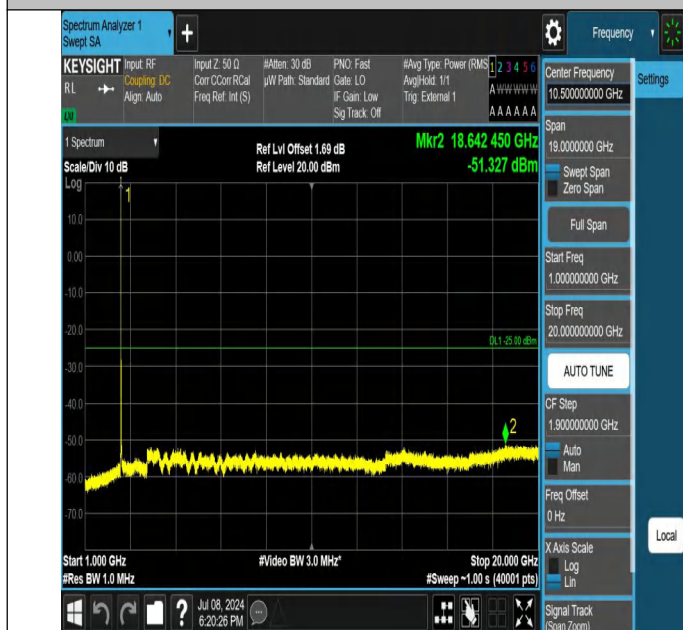
41-41-5MHz-20MHz-QPSK-QPSK-39683-39800-1RB#24-0RB#0- 1000~20000MHz-PASS
