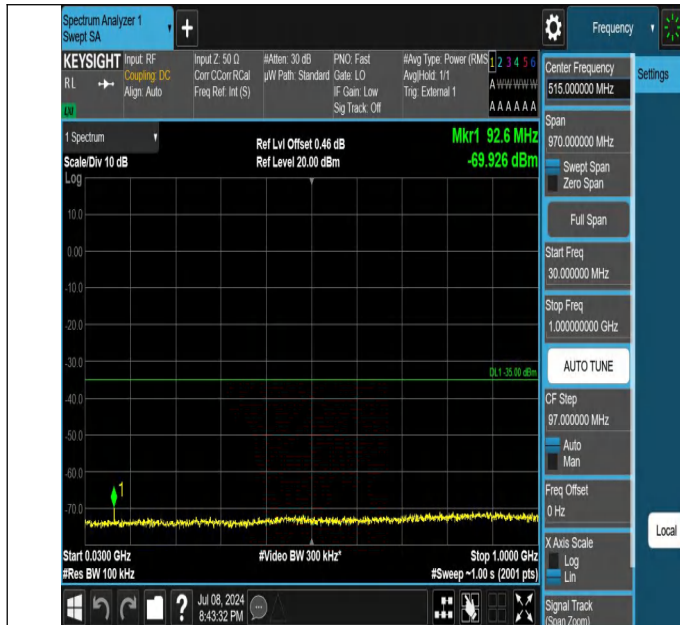
41-41-20MHz-15MHz-QPSK-QPSK-39750-39921-1RB#99-0RB# 0-30~1000MHz-PASS
