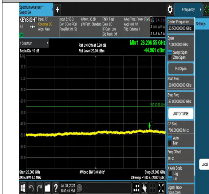
41-41-20MHz-15MHz-QPSK-QPSK-40546-40717-1RB#0-1RB#7 4-20000~27000MHz-PASS
