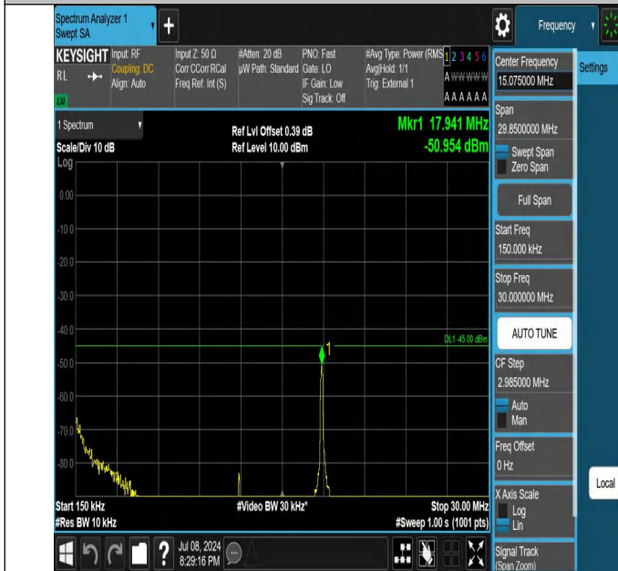
41-41-20MHz-10MHz-QPSK-QPSK-40571-40715-1RB#0-0RB#0- 0.15~30MHz-PASS
