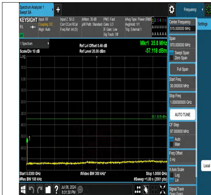
41-41-20MHz-10MHz-QPSK-QPSK-40571-40715-1RB#99-0RB# 0-30~1000MHz-PASS
