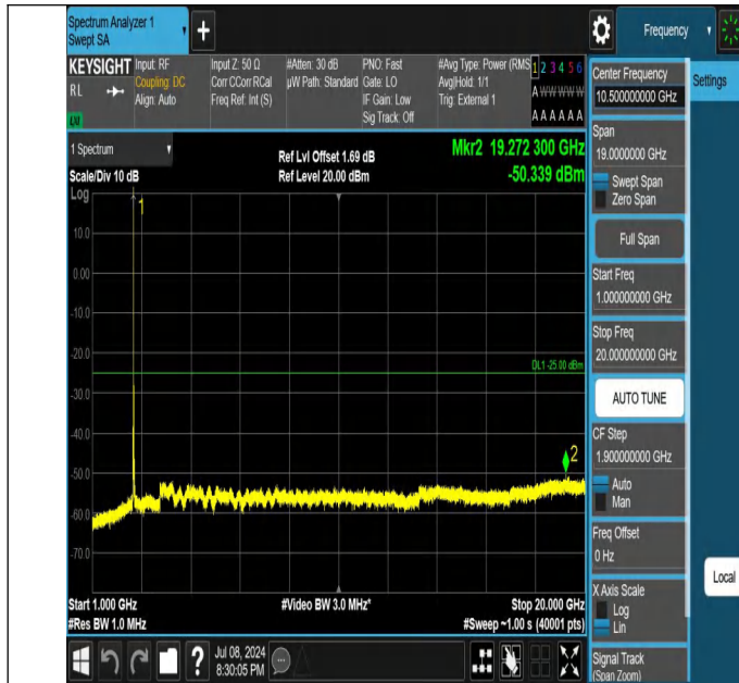
41-41-20MHz-10MHz-QPSK-QPSK-40571-40715-1RB#0-0RB#0-1000~20000MHz-PASS
