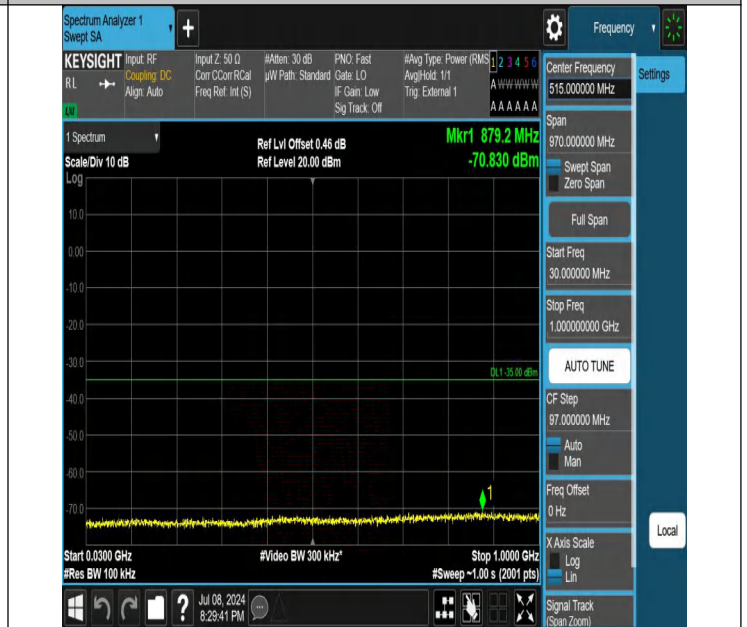
41-41-20MHz-10MHz-QPSK-QPSK-40571-40715-1RB#0-0RB#0- 30~1000MHz-PASS
