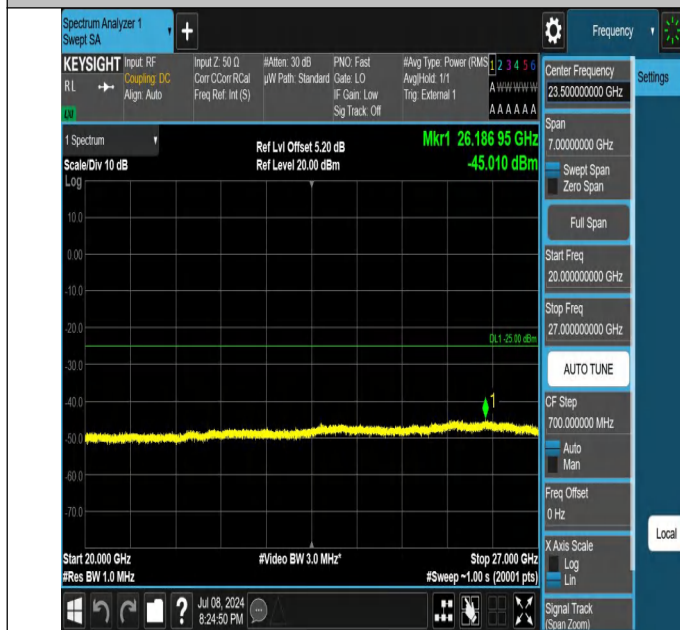
41-41-20MHz-10MHz-QPSK-QPSK-39750-39894-1RB#0-0RB#0-20000~27000MHz-PASS
