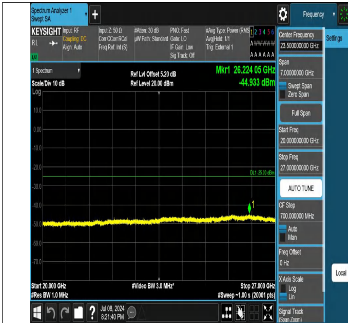
41-41-20MHz-5MHz-QPSK-QPSK-41440-41557-1RB#0-1RB#24-20000~27000MHz-PASS
