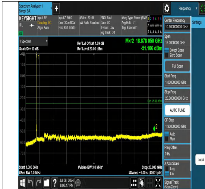
41-41-20MHz-5MHz-QPSK-QPSK-39750-39867-1RB#99-0RB#0- 1000~20000MHz-PASS
