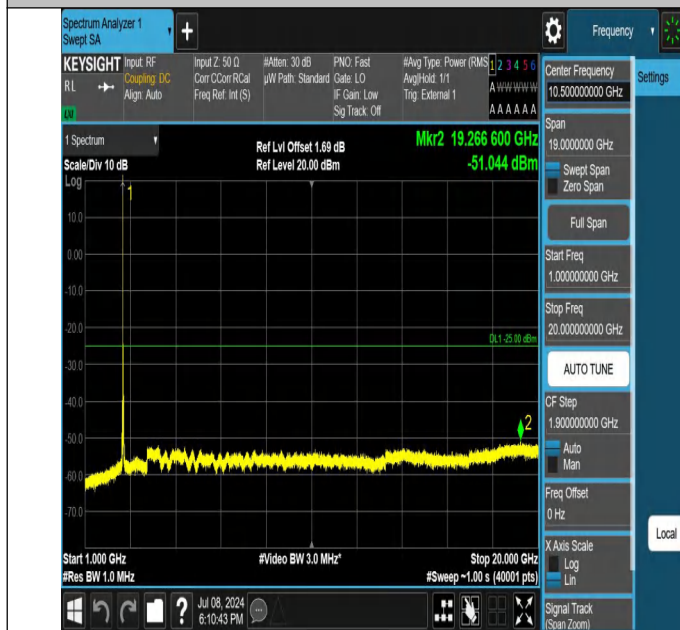
38-38-20MHz-20MHz-QPSK-QPSK-37952-38150-1RB#0-0RB#0- 1000~20000MHz-PASS
