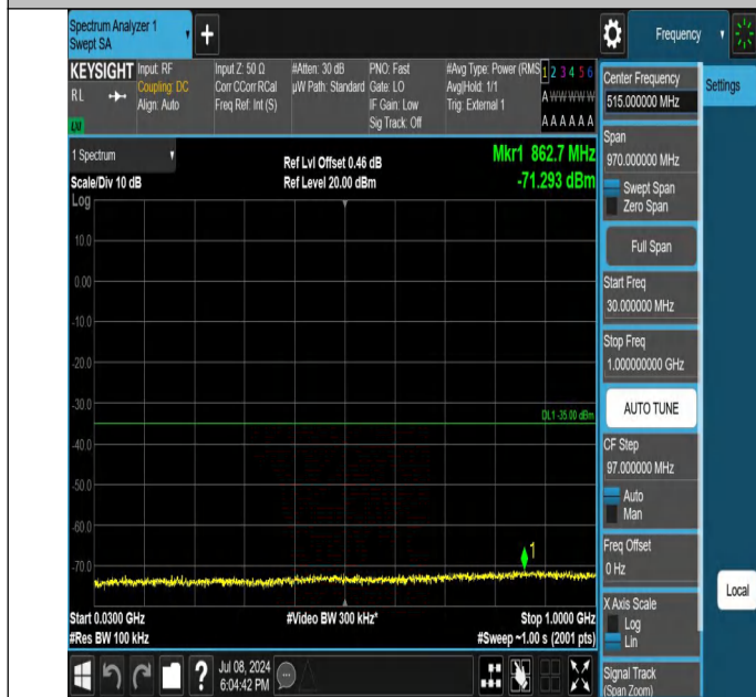
38-38-20MHz-20MHz-QPSK-QPSK-37901-38099-1RB#0-0RB#0-30~1000MHz-PASS
