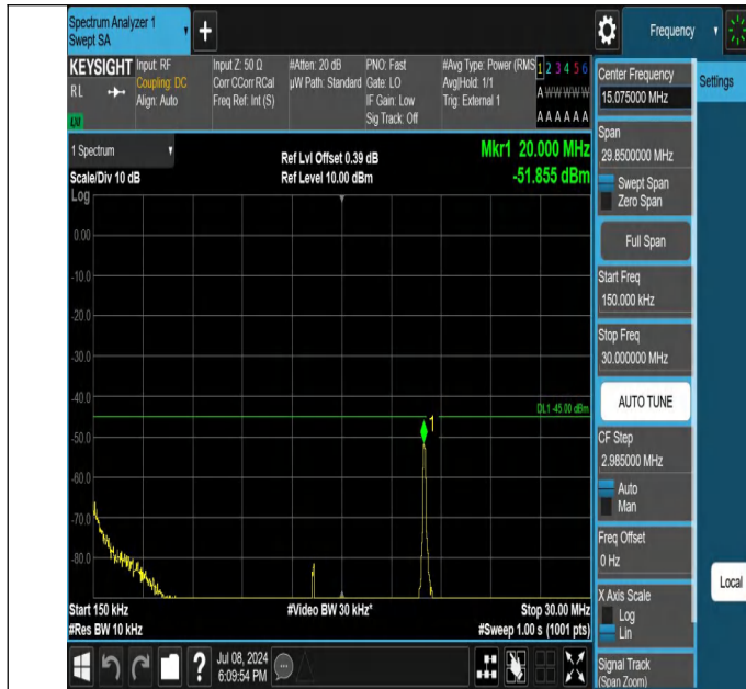
38-38-20MHz-20MHz-QPSK-QPSK-37952-38150-1RB#0-0RB#0- 0.15~30MHz-PASS
