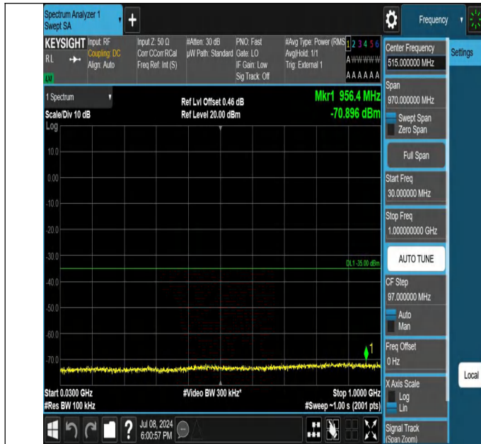
38-38-20MHz-20MHz-QPSK-QPSK-37850-38048-1RB#99-0RB# 0-30~1000MHz-PASS
