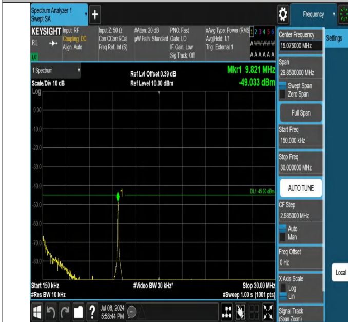
38-38-20MHz-20MHz-QPSK-QPSK-37850-38048-1RB#0-0RB#0- 0.15~30MHz-PASS
