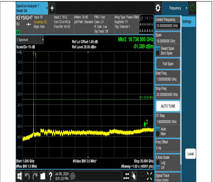
38-38-20MHz-20MHz-QPSK-QPSK-37850-38048-1RB#99-0RB# 0-1000~20000MHz-PASS
