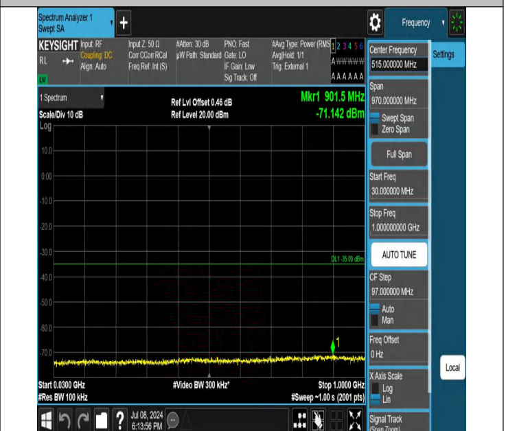
38-38-20MHz-20MHz-QPSK-QPSK-37952-38150-1RB#0-1RB#9 9-30~1000MHz-PASS
