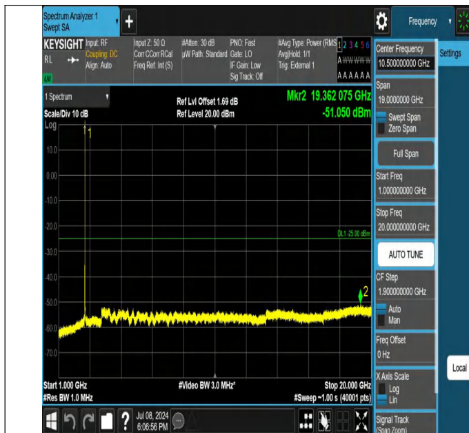
38-38-20MHz-20MHz-QPSK-QPSK-37901-38099-1RB#99-0RB# 0-1000~20000MHz-PASS
