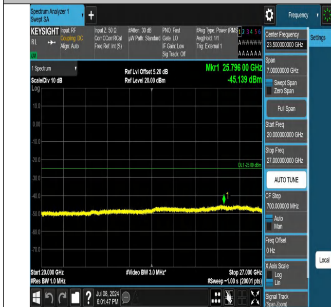
38-38-20MHz-20MHz-QPSK-QPSK-37850-38048-1RB#99-0RB# 0-20000~27000MHz-PASS
