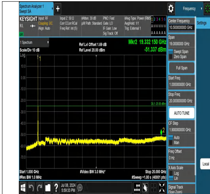
38-38-20MHz-20MHz-QPSK-QPSK-37850-38048-1RB#0-0RB#0-1000~20000MHz-PASS
