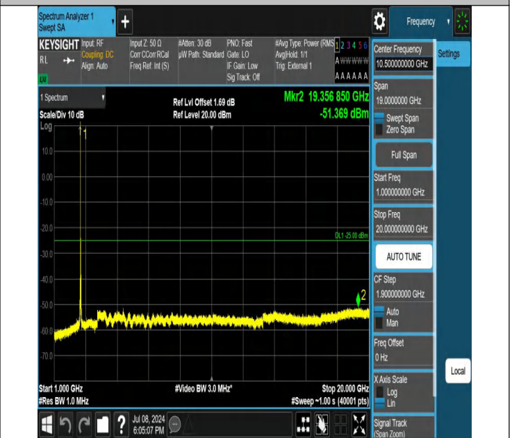
38-38-20MHz-20MHz-QPSK-QPSK-37901-38099-1RB#0-0RB#0-1000~20000MHz-PASS
