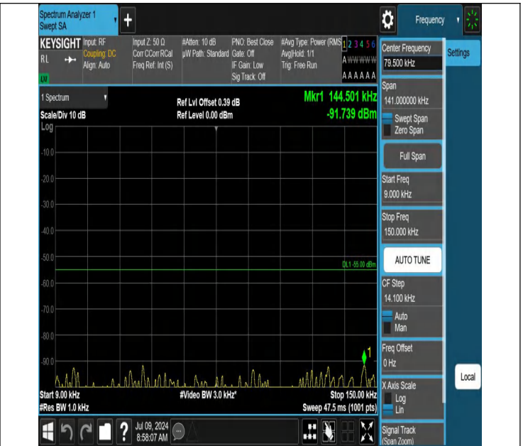
38-38-20MHz-20MHz-QPSK-QPSK-37850-38048-1RB#0-0RB#0- 0.009~0.15MHz-PASS
