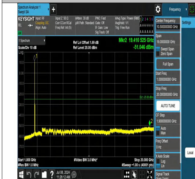
7-7-15MHz-20MHz-QPSK-QPSK-20828-20999-1RB#0-1RB#99-1 000~20000MHz-PASS
