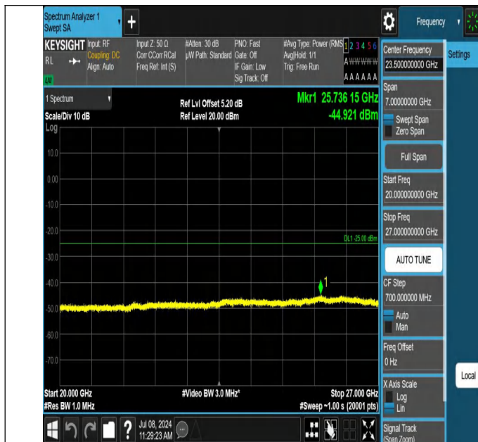
7-7-15MHz-20MHz-QPSK-QPSK-21179-21350-1RB#74-0RB#0-2 0000~27000MHz-PASS
