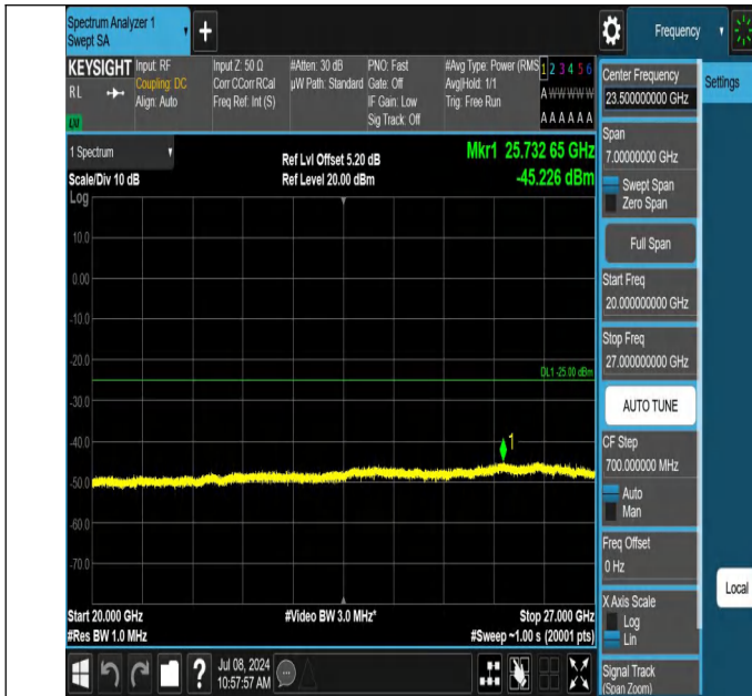
7-7-10MHz-20MHz-QPSK-QPSK-21206-21350-1RB#0-1RB#99-2 0000~27000MHz-PASS
