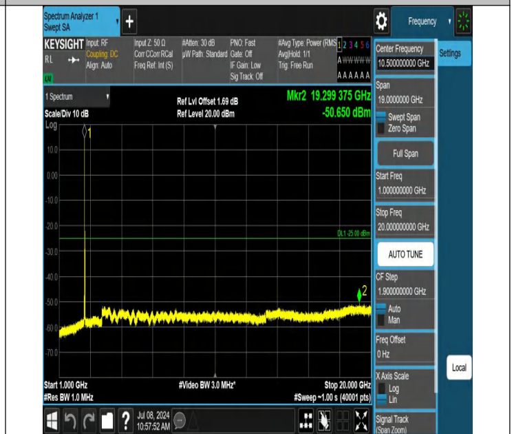
7-7-10MHz-20MHz-QPSK-QPSK-21206-21350-1RB#0-1RB#99-1 000~20000MHz-PASS
