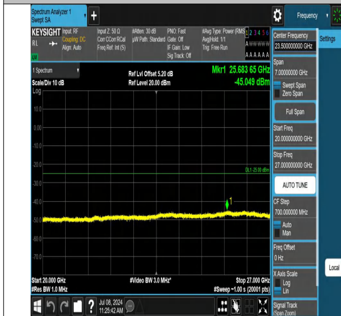
7-7-15MHz-20MHz-QPSK-QPSK-20828-20999-1RB#74-0RB#0-2 0000~27000MHz-PASS
