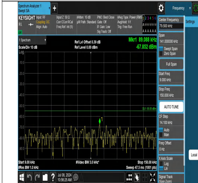
7-7-10MHz-20MHz-QPSK-QPSK-21206-21350-1RB#0-0RB#0-0. 009~0.15MHz-PASS
