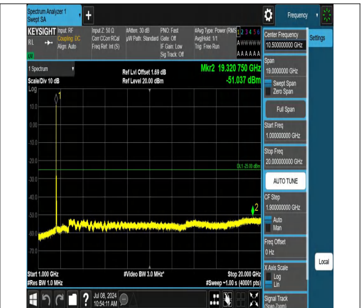
7-7-10MHz-20MHz-QPSK-QPSK-20805-20949-1RB#0-1RB#99-1 000~20000MHz-PASS
