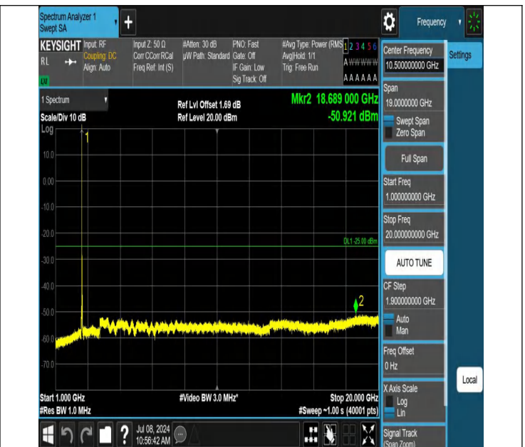
7-7-10MHz-20MHz-QPSK-QPSK-21206-21350-1RB#0-0RB#0-10 00~20000MHz-PASS
