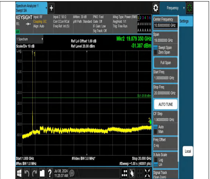
7-7-15MHz-20MHz-QPSK-QPSK-20828-20999-1RB#74-0RB#0-1 000~20000MHz-PASS
