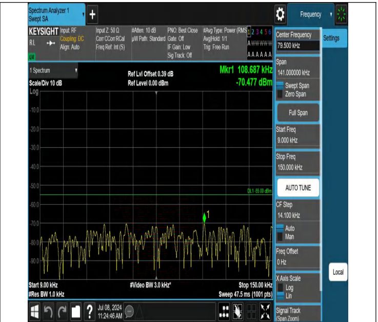
7-7-15MHz-20MHz-QPSK-QPSK-20828-20999-1RB#0-0RB#0-0. 009~0.15MHz-PASS
