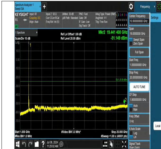
7-7-15MHz-20MHz-QPSK-QPSK-20828-20999-1RB#0-0RB#0-10 00~20000MHz-PASS
