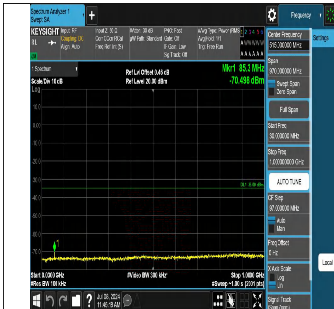
7-7-20MHz-15MHz-QPSK-QPSK-21026-21197-1RB#0-0RB#0-30 ~1000MHz-PASS
