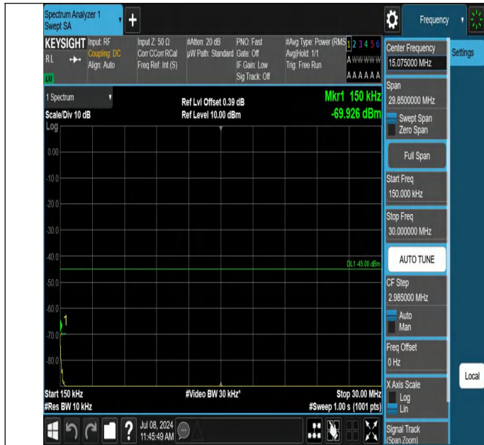
7-7-20MHz-15MHz-QPSK-QPSK-21026-21197-1RB#99-0RB#0-0 .15~30MHz-PASS
