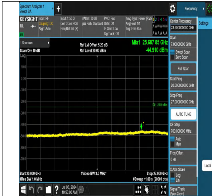
7-7-10MHz-20MHz-QPSK-QPSK-20805-20949-1RB#0-0RB#0-20 000~27000MHz-PASS
