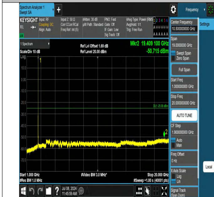
7-7-20MHz-15MHz-QPSK-QPSK-21026-21197-1RB#99-0RB#0-1 000~20000MHz-PASS
