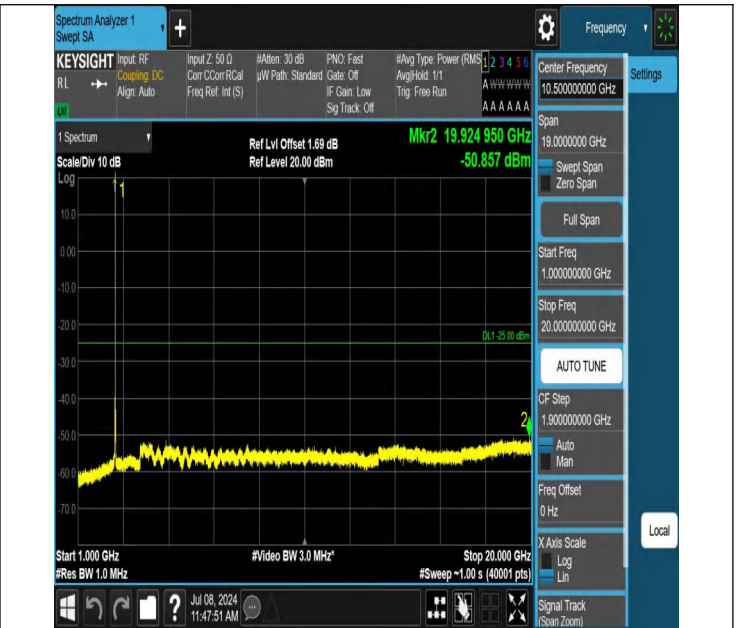
7-7-20MHz-15MHz-QPSK-QPSK-21201-21372-1RB#99-0RB#0-1 000~20000MHz-PASS
