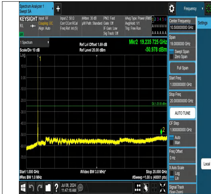
7-7-20MHz-15MHz-QPSK-QPSK-21201-21372-1RB#0-0RB#0-10 00~20000MHz-PASS
