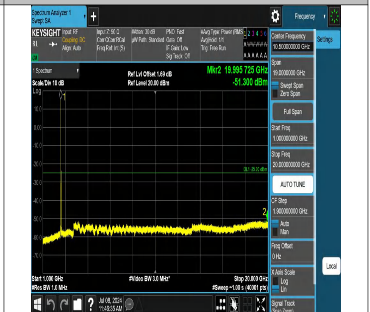
7-7-20MHz-15MHz-QPSK-QPSK-21026-21197-1RB#0-1RB#74-1 000~20000MHz-PASS
