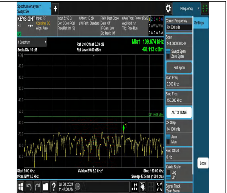
7-7-20MHz-15MHz-QPSK-QPSK-21201-21372-1RB#0-0RB#0-0. 009~0.15MHz-PASS
