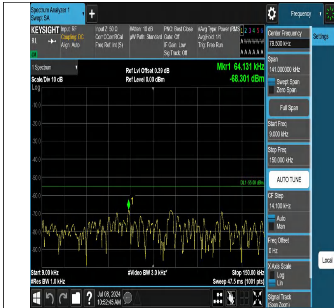
7-7-10MHz-20MHz-QPSK-QPSK-20805-20949-1RB#0-ORB#0-0. 009~0.15MHz-PASS
