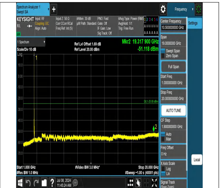
7-7-20MHz-15MHz-QPSK-QPSK-21026-21197-1RB#0-0RB#0-10 00~20000MHz-PASS
