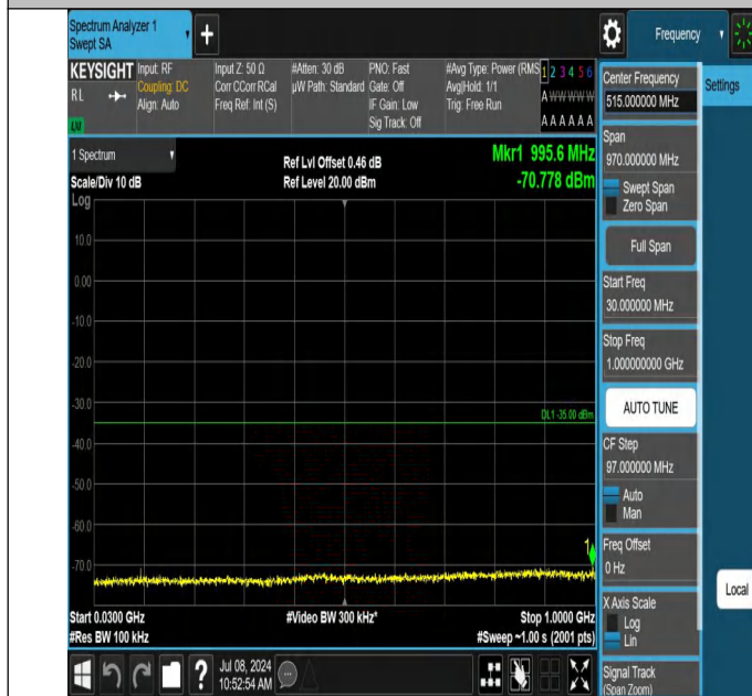
7-7-10MHz-20MHz-QPSK-QPSK-20805-20949-1RB#0-ORB#0-30 ~1000MHz-PASS
