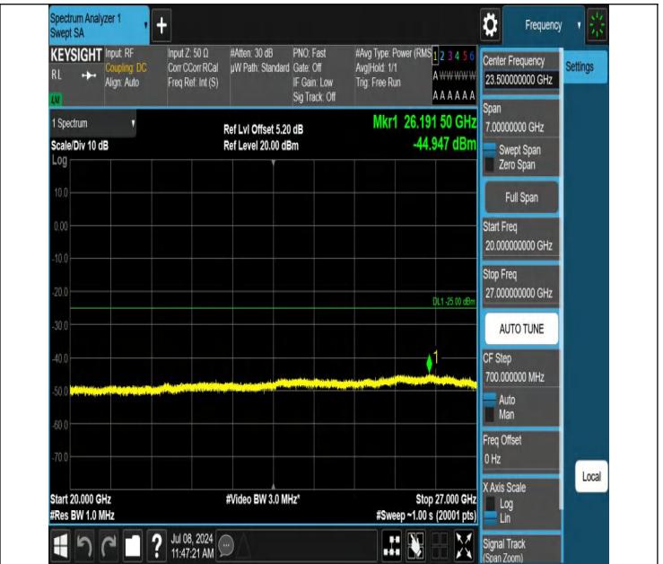
7-7-20MHz-15MHz-QPSK-QPSK-21201-21372-1RB#0-0RB#0-20 000~27000MHz-PASS
