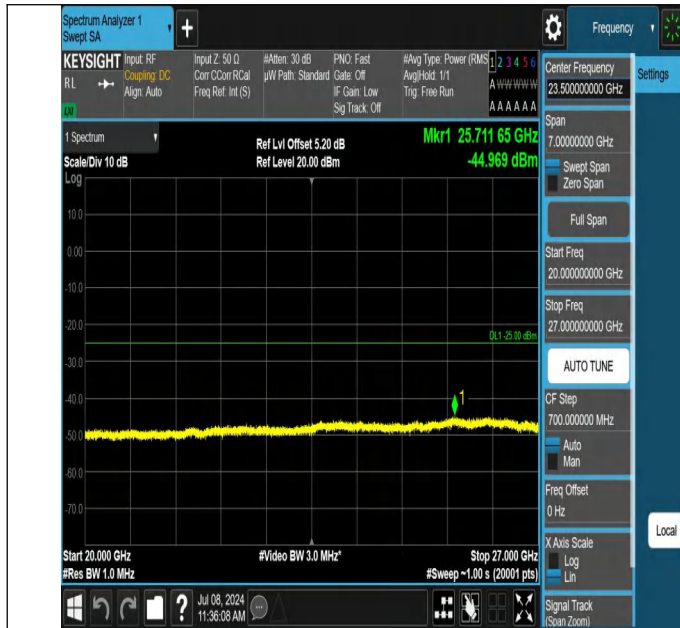
7-7-20MHz-10MHz-QPSK-QPSK-21051-21195-1RB#0-0RB#0-20 000~27000MHz-PASS
