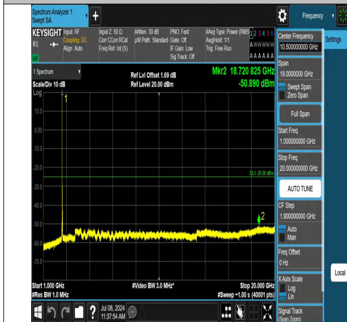
7-7-20MHz-10MHz-QPSK-QPSK-21251-21395-1RB#0-0RB#0-10 00~20000MHz-PASS
