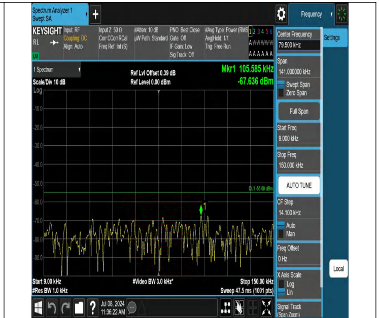
7-7-20MHz-10MHz-QPSK-QPSK-21051-21195-1RB#99-0RB#0-0. 009~0.15MHz-PASS
