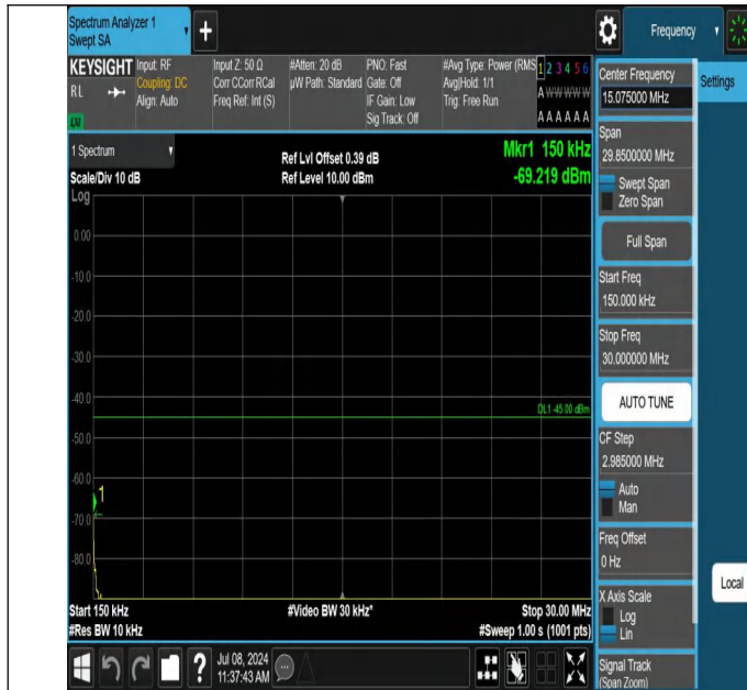
7-7-20MHz-10MHz-QPSK-QPSK-21251-21395-1RB#0-0RB#0-0. 15~30MHz-PASS
