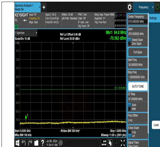
7-7-20MHz-10MHz-QPSK-QPSK-20850-20994-1RB#99-0RB#0-3 0~1000MHz-PASS
