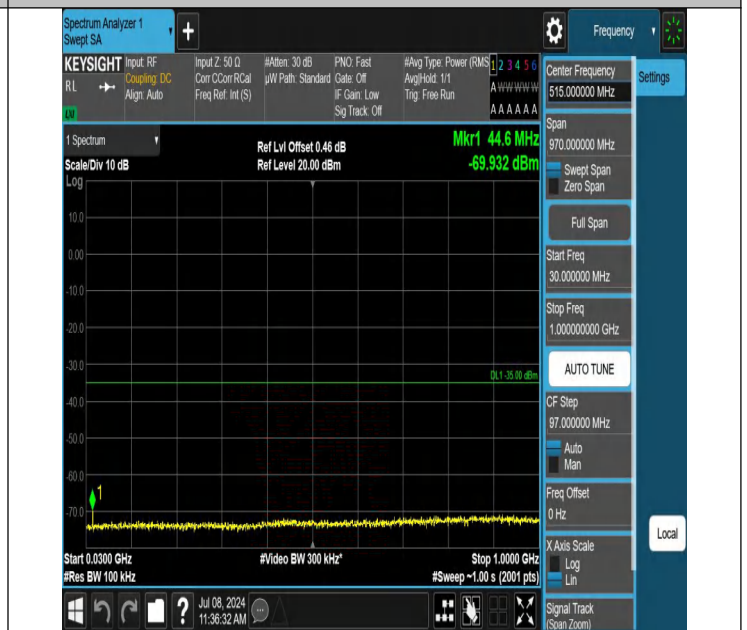
7-7-20MHz-10MHz-QPSK-QPSK-21051-21195-1RB#99-0RB#0-3 0~1000MHz-PASS
