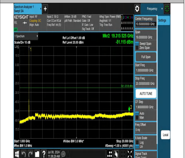
7-7-20MHz-10MHz-QPSK-QPSK-21251-21395-1RB#99-0RB#0-1 000~20000MHz-PASS
