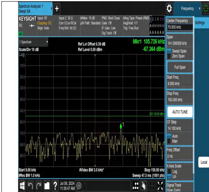
7-7-20MHz-10MHz-QPSK-QPSK-21051-21195-1RB#0-0RB#0-0. 009~0.15MHz-PASS
