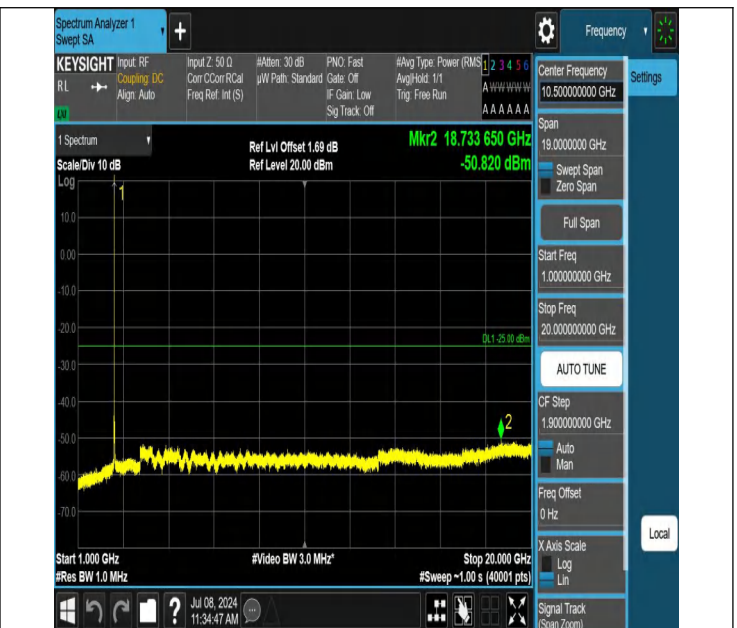
7-7-20MHz-10MHz-QPSK-QPSK-20850-20994-1RB#99-0RB#0-1 000~20000MHz-PASS
