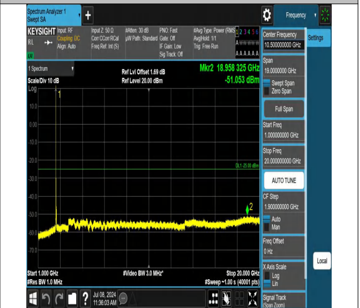
7-7-20MHz-10MHz-QPSK-QPSK-21051-21195-1RB#0-0RB#0-10 00~20000MHz-PASS
