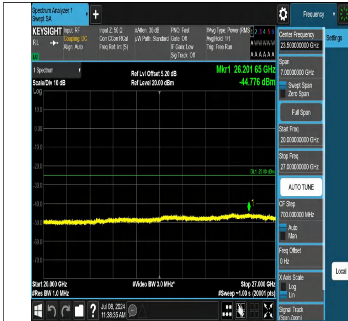
7-7-20MHz-10MHz-QPSK-QPSK-21251-21395-1RB#99-0RB#0-2 0000~27000MHz-PASS
