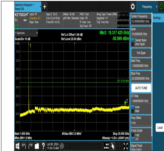
7-7-20MHz-10MHz-QPSK-QPSK-20850-20994-1RB#0-0RB#0-10 00~20000MHz-PASS
