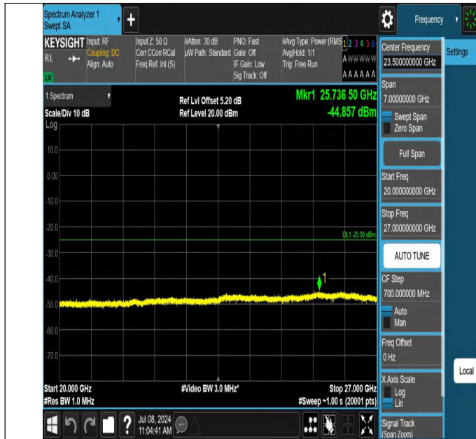
7-7-15MHz-10MHz-QPSK-QPSK-21051-21171-1RB#74-0RB#0-2 0000~27000MHz-PASS
