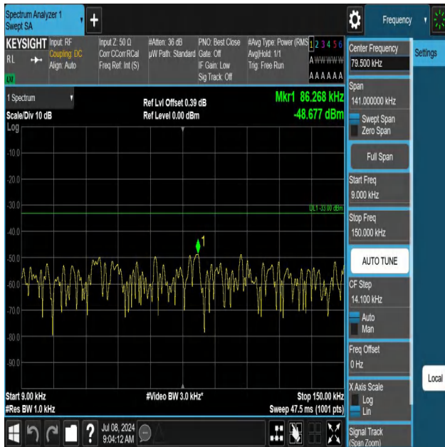
5-5-10MHz-10MHz-QPSK-QPSK-20501-20600-1RB#0-0RB#0-0. 009~0.15MHz-PASS
