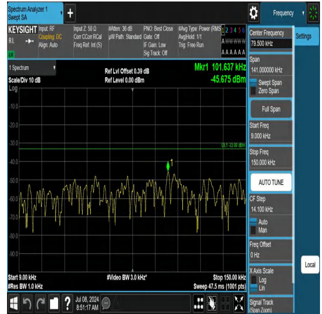
5-5-5MHz-10MHz-QPSK-QPSK-20528-20600-1RB#0-0RB#0-0.0 09~0.15MHz-PASS
