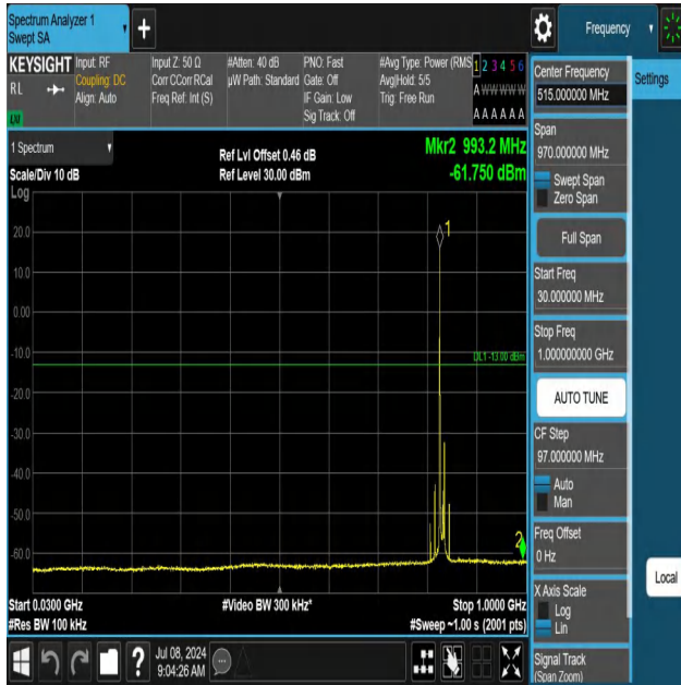
5-5-10MHz-10MHz-QPSK-QPSK-20501-20600-1RB#0-ORB#0-30 ~1000MHz-PASS
