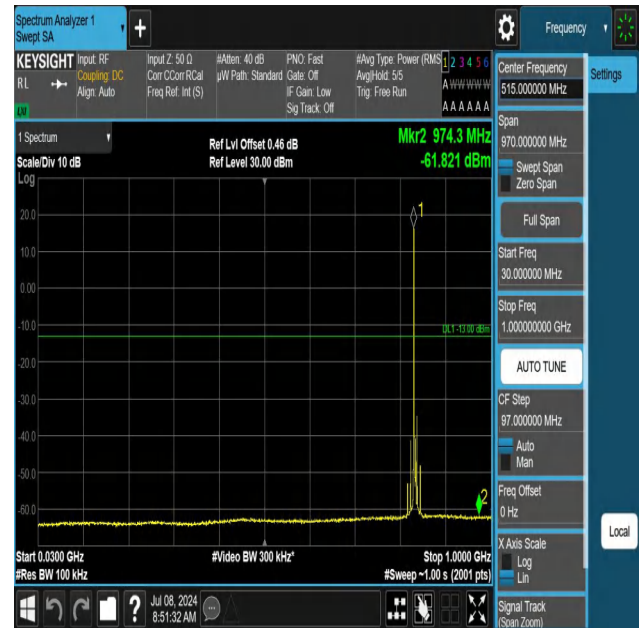
5-5-5MHz-10MHz-QPSK-QPSK-20528-20600-1RB#0-0RB#0-30~ 1000MHz-PASS
