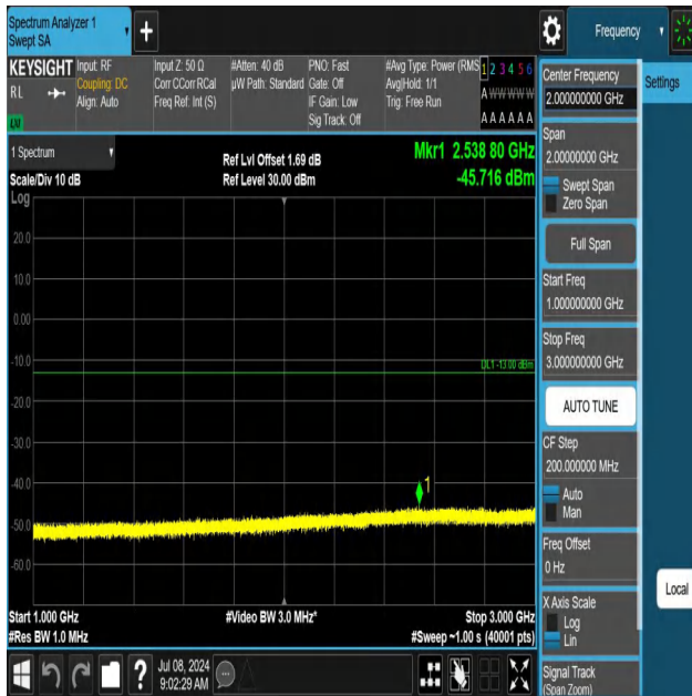
5-5-10MHz-10MHz-QPSK-QPSK-20476-20575-1RB#0-ORB#0-10 00~3000MHz-PASS
