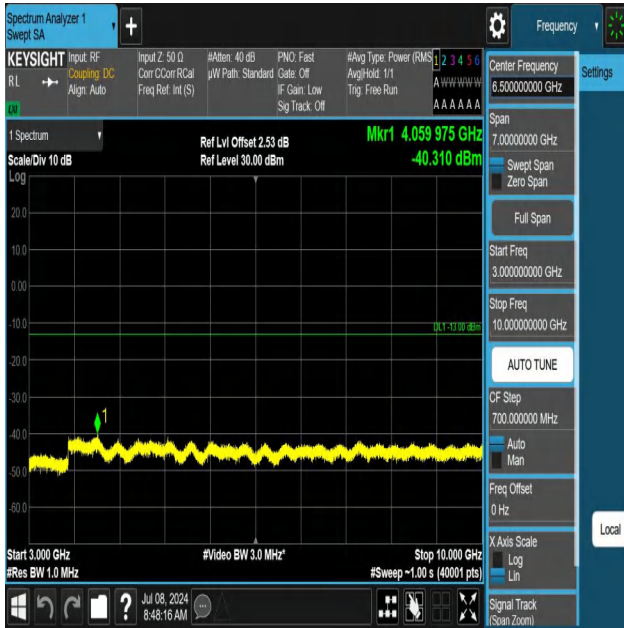
5-5-5MHz-10MHz-QPSK-QPSK-20428-20500-1RB#24-0RB#0-30 00~10000MHz-PASS
