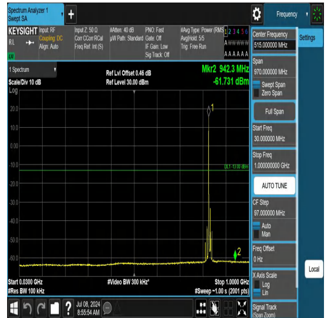
5-5-10MHz-5MHz-QPSK-QPSK-20500-20572-1RB#0-0RB#0-30~ 1000MHz-PASS
