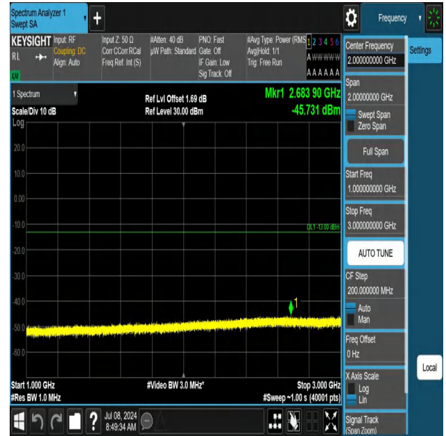
5-5-5MHz-10MHz-QPSK-QPSK-20478-20550-1RB#0-ORB#0-100 0~3000MHz-PASS
