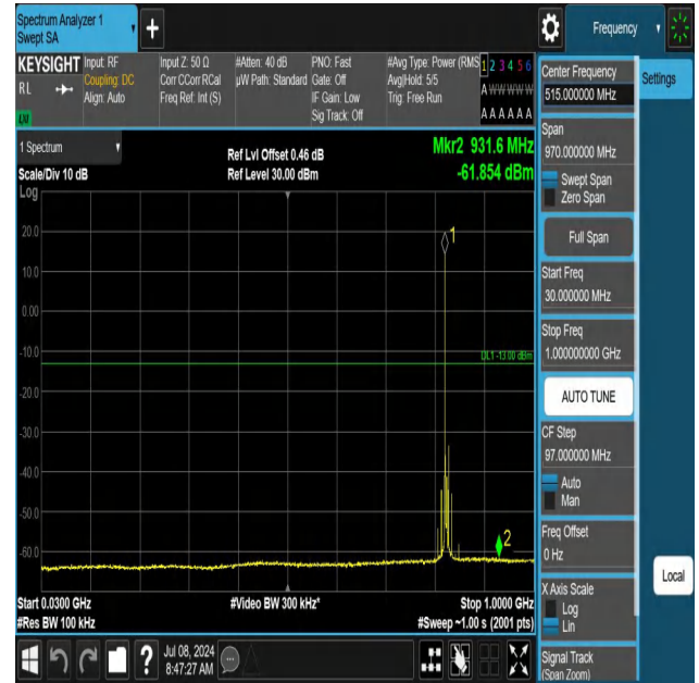
5-5-5MHz-10MHz-QPSK-QPSK-20428-20500-1RB#0-ORB#0-30~ 1000MHz-PASS
