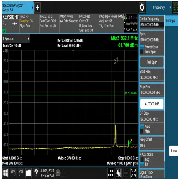
5-5-5MHz-10MHz-QPSK-QPSK-20478-20550-1RB#0-ORB#0-30~ 1000MHz-PASS
