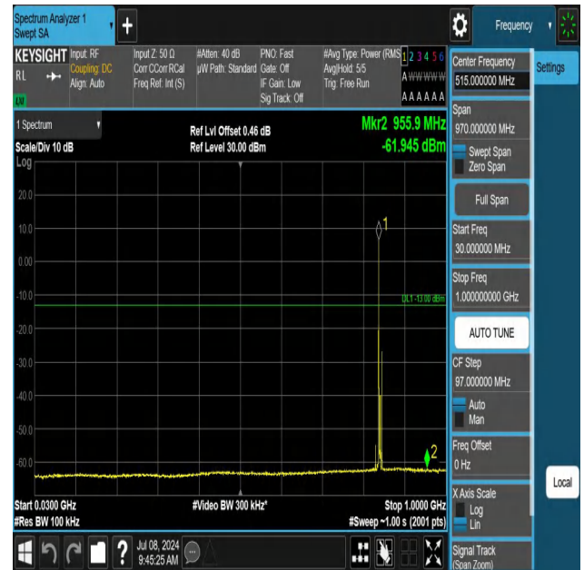
5-5-3MHz-5MHz-QPSK-QPSK-20586-20625-1RB#0-1RB#24-30~ 1000MHz-PASS
