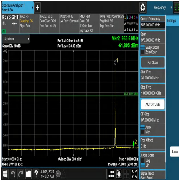
5-5-3MHz-5MHz-QPSK-QPSK-20416-20455-1RB#14-0RB#0-30~ 1000MHz-PASS
