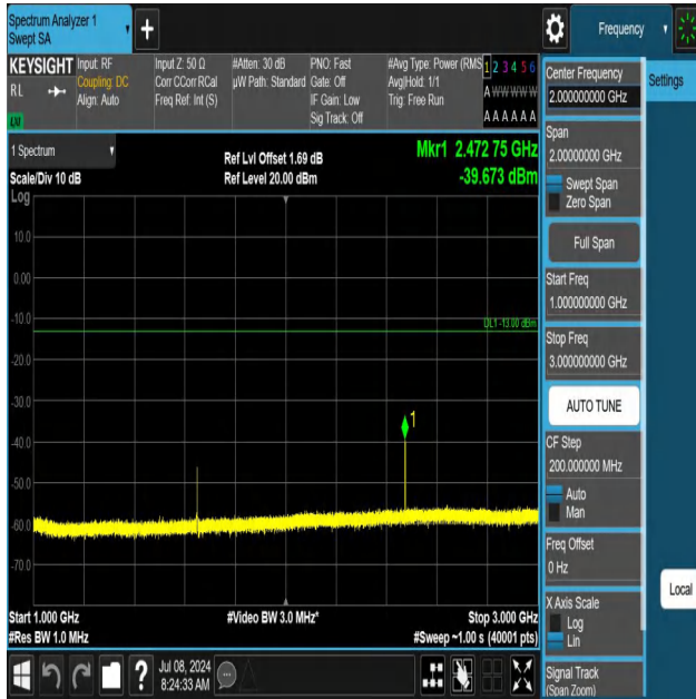
5-5-3MHz-5MHz-QPSK-QPSK-20416-20455-1RB#0-0RB#0-1000 ~3000MHz-PASS
