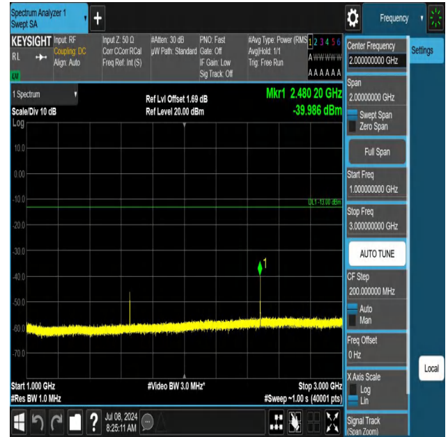
5-5-3MHz-5MHz-QPSK-QPSK-20416-20455-1RB#14-0RB#0-100 0~3000MHz-PASS
