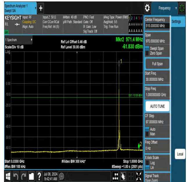
5-5-3MHz-5MHz-QPSK-QPSK-20416-20455-1RB#0-0RB#0-30~1 000MHz-PASS
