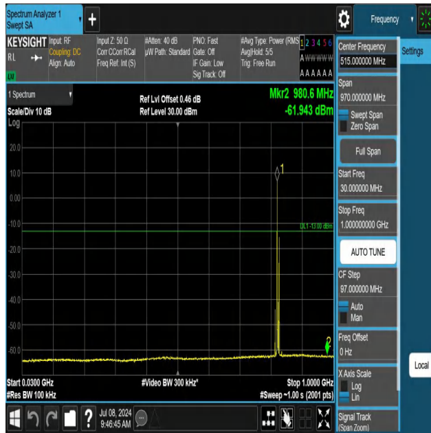
5-5-5MHz-3MHz-QPSK-QPSK-20425-20464-1RB#0-1RB#15-30~ 1000MHz-PASS
