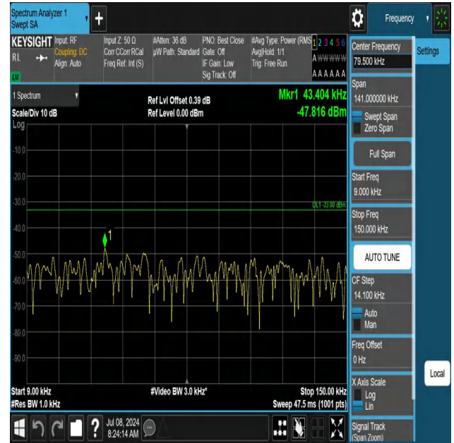
5-5-3MHz-5MHz-QPSK-QPSK-20416-20455-1RB#0-0RB#0-0.00 9~0.15MHz-PASS
