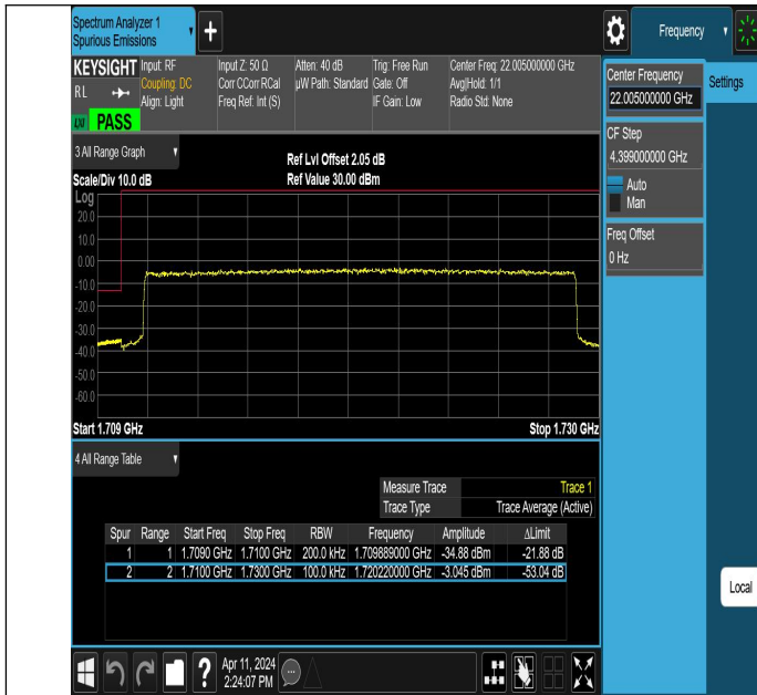
Band66_20MHz_QPSK_132072_100RB#0
