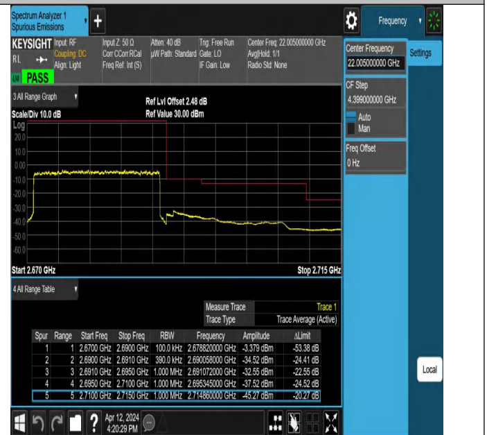
Band41_20MHz_QPSK_41490_100RB#0
