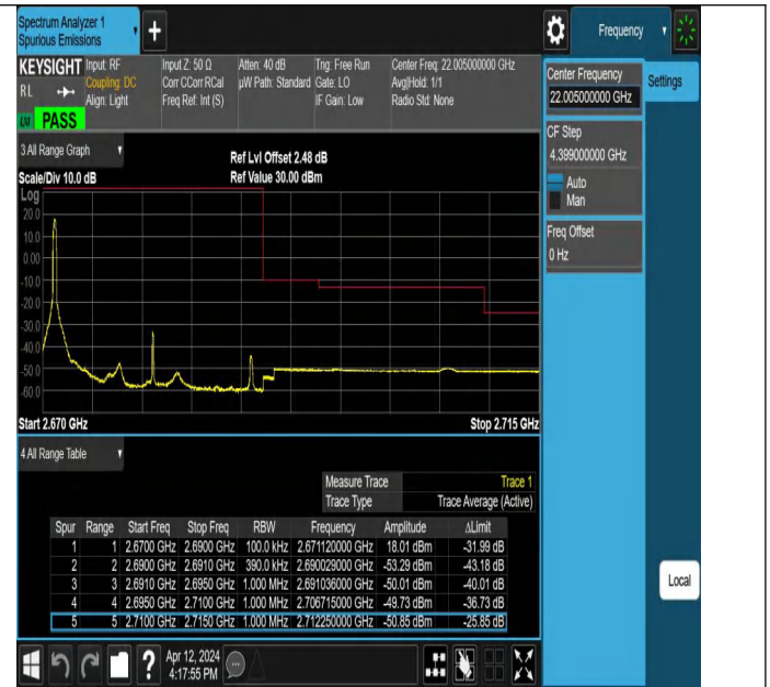
Band41_20MHz_QPSK_41490_1RB#0
