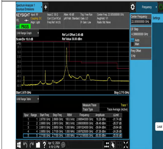
Band41_20MHz_QPSK_41490_1RB#99
