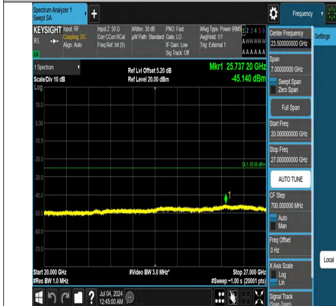
Band41-15MHz-QPSK-39725-1RB#0-20000~27000-PASS
