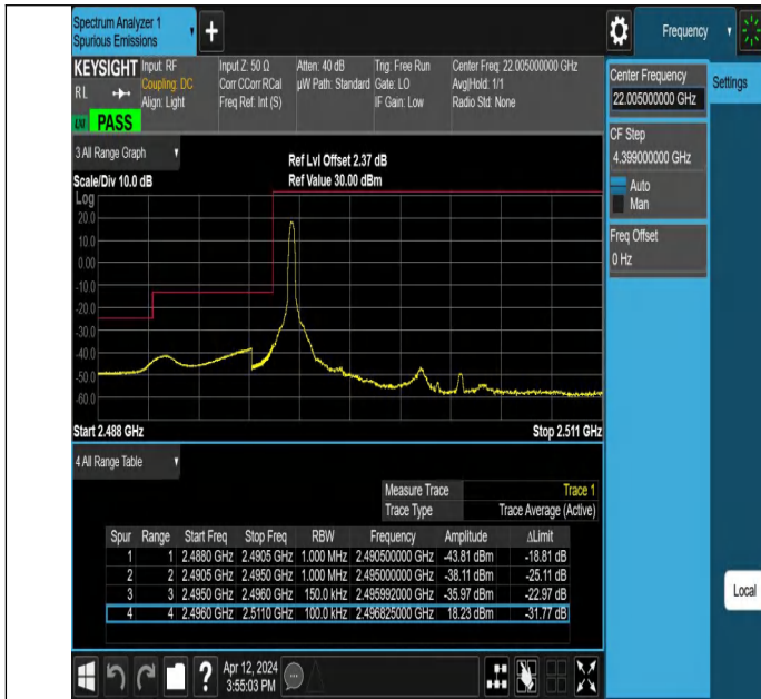
Band41_15MHz_QPSK_39725_1RB#0
