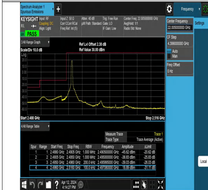
Band41_20MHz_QPSK_39750_1RB#0
