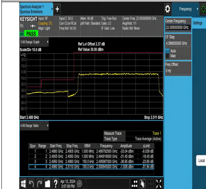
Band41_15MHz_QPSK_39725_75RB#0
