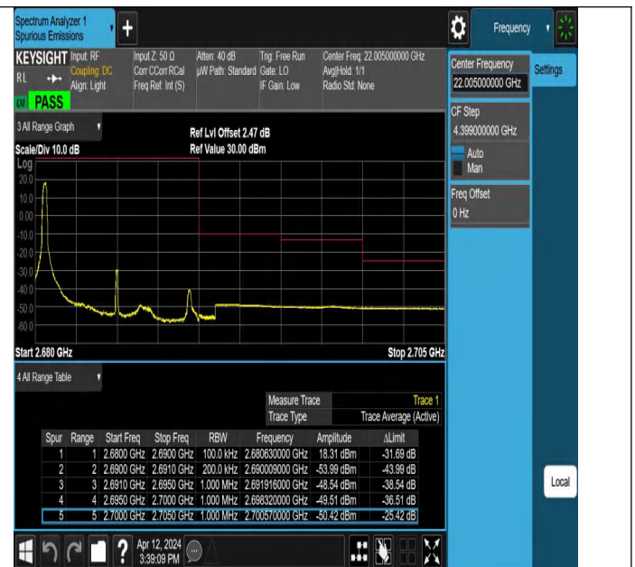
Band41_10MHz_QPSK_41540_1RB#0
