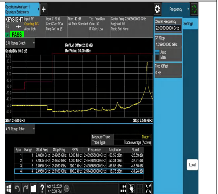
Band41_20MHz_QPSK_39750_1RB#99
