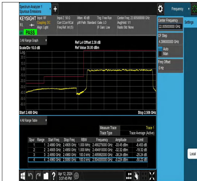
Band41_10MHz_QPSK_39700_50RB#0
