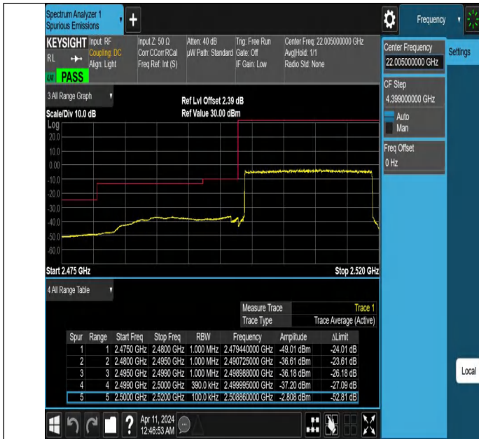
Band7_20MHz_QPSK_20850_100RB#0
