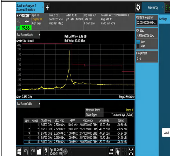
Band7_20MHz_QPSK_21350_1RB#99
