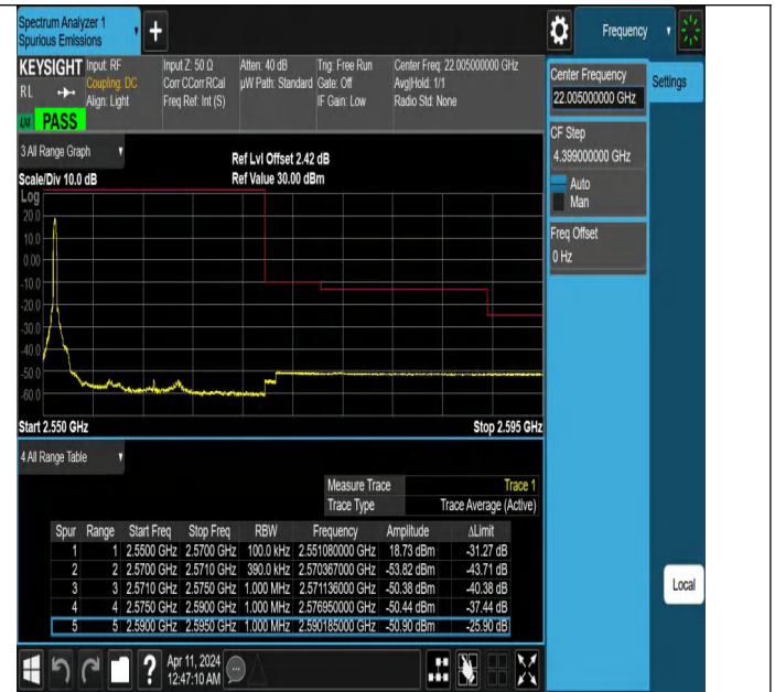
Band7_20MHz_QPSK_21350_1RB#0
