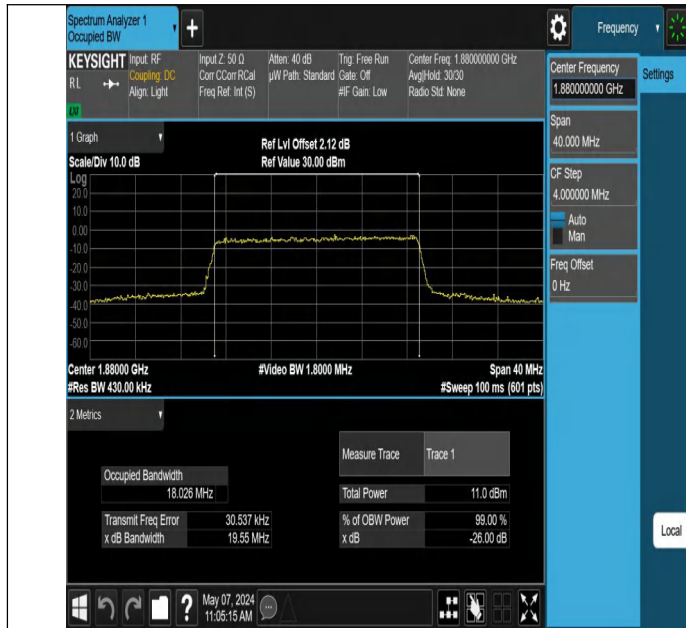
Band2-20MHz-QPSK-18900-100RB#0-PASS
