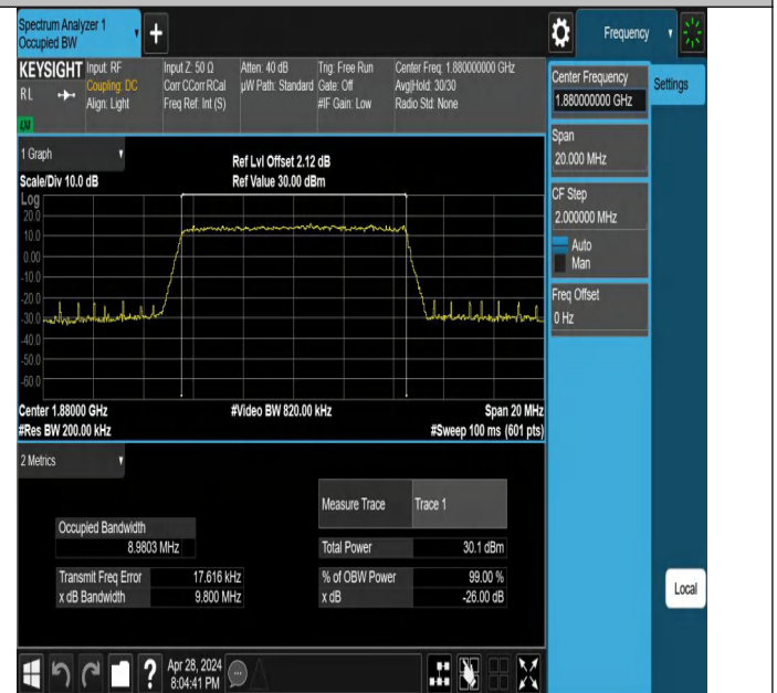
Band2-10MHz-16QAM-18900-50RB#0-PASS
